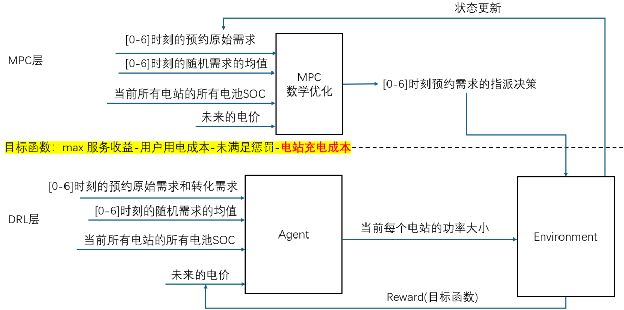
图 1: MPC-RL 协同优化框架（图中的随机需求均值是逐请求预测集合 \mathcal{R} 的站点-时段聚合表示；随机实际到达通过状态更新反馈，未在图中单列；站级功率在数学模型中展开为逐电池连续功率向量）
