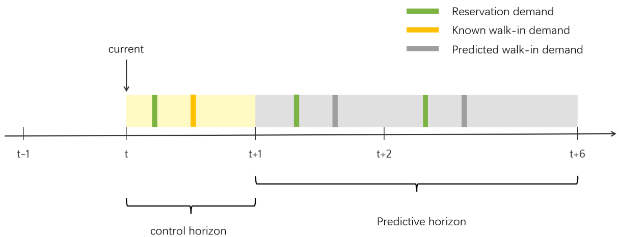
图 2: Rolling Horizon
