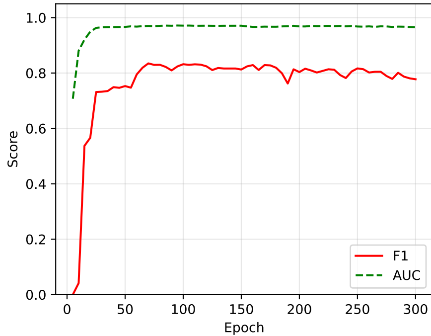
(b) Validation F1 & AUC
