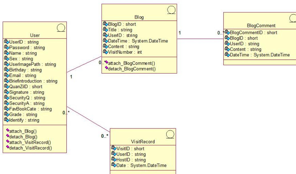
图 4-16 “个人博客管理”功能的类图
