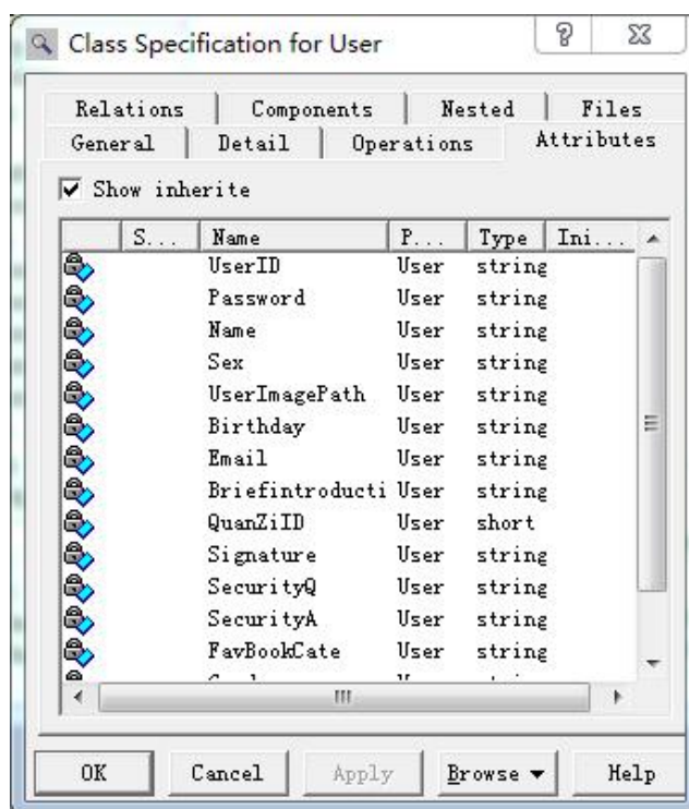
图 4-13 添加类的属性
