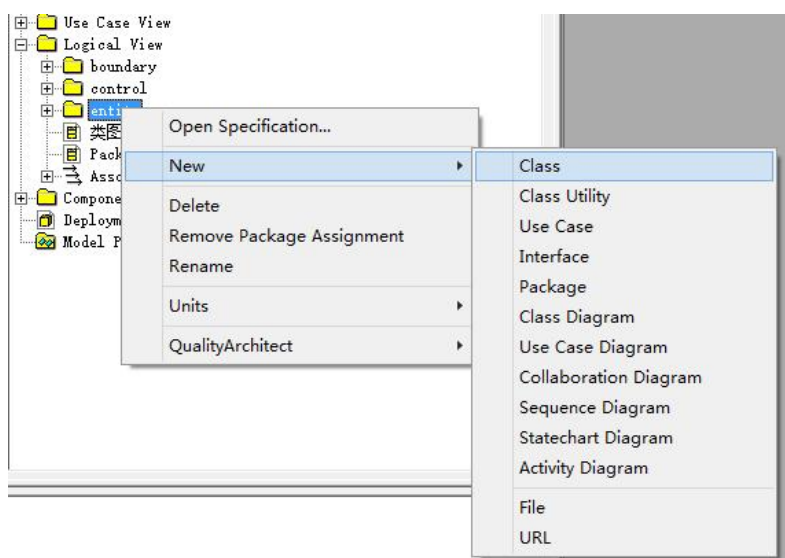
图 4-12 创建类
