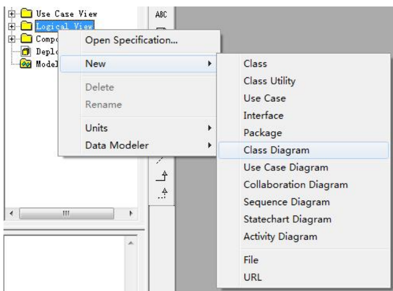
图 4-15 新建类图
