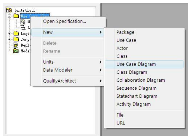
图 4-2 创建用例图
