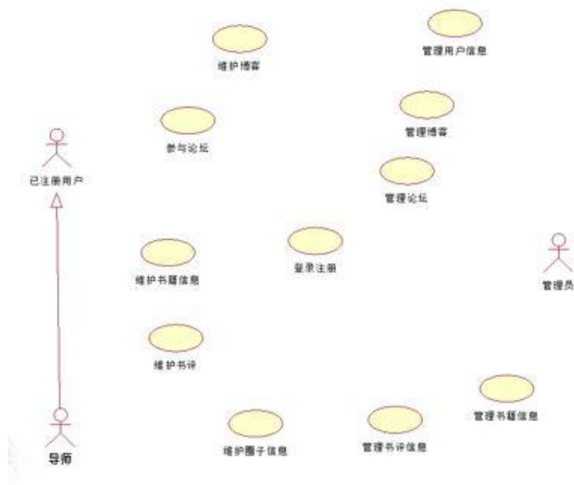
图 4-6 添加用例
