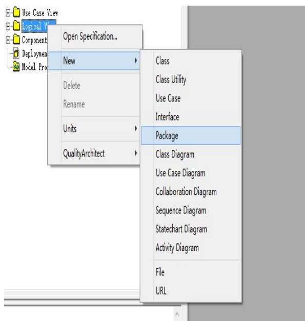
图 4-11 创建包
