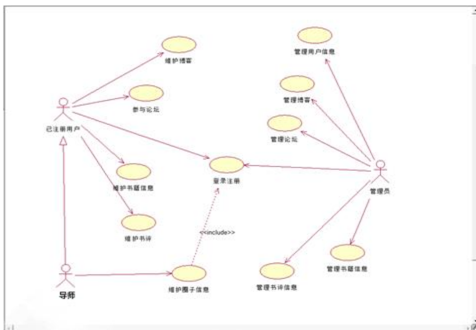
图 4-9 “‘墨韵’读书会书籍共享管理平台”的用例图
