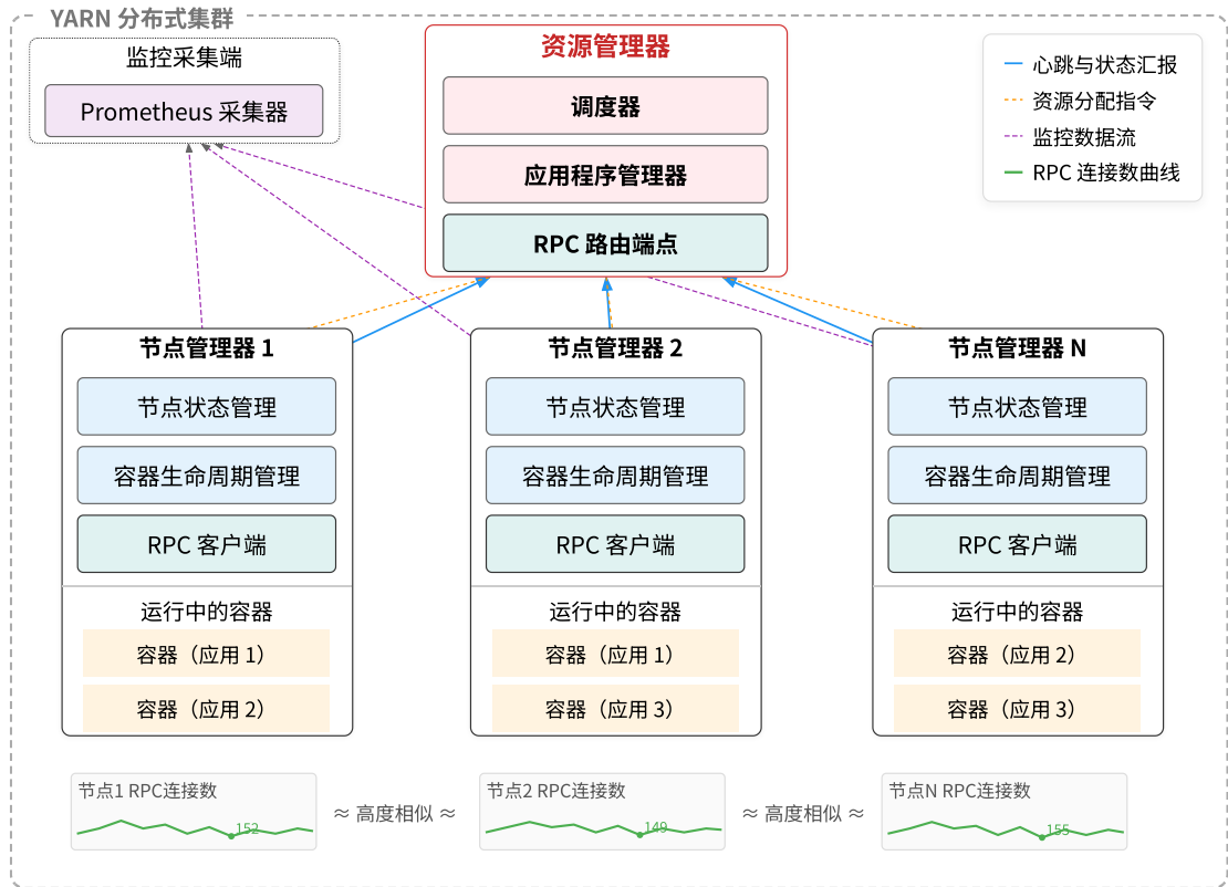
图 3-1 YARN 分布式集群架构与 RPC Router 连接数指标示意
