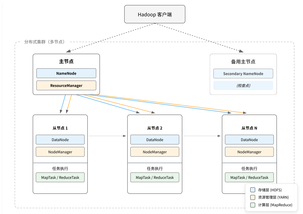
图 2-5 Hadoop 分布式集群架构示意图
