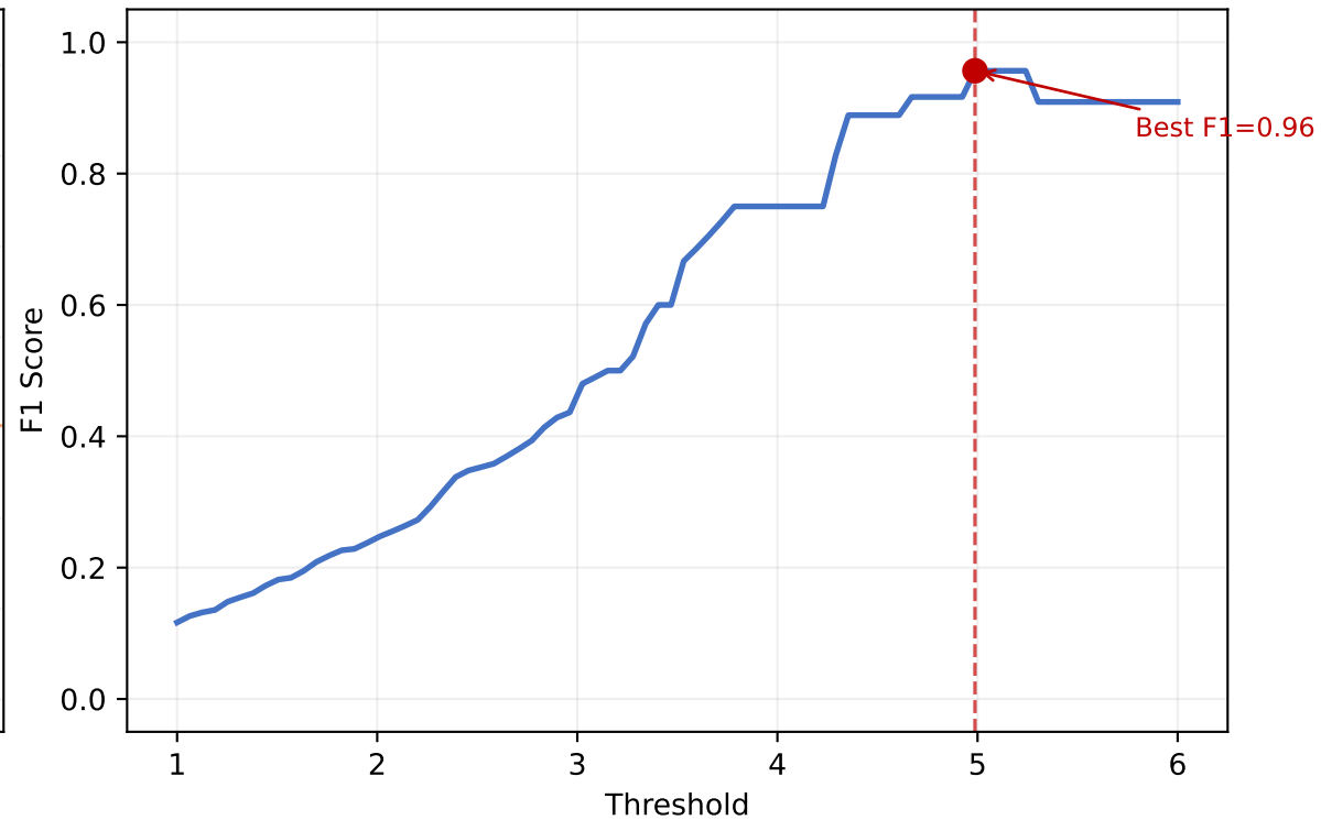
Threshold vs F1 Score
