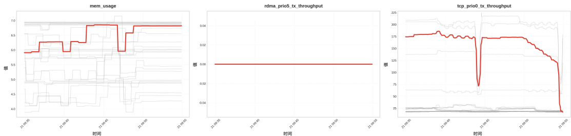
图 4-1 GPU 集群典型故障案例的多指标多节点时序可视化
