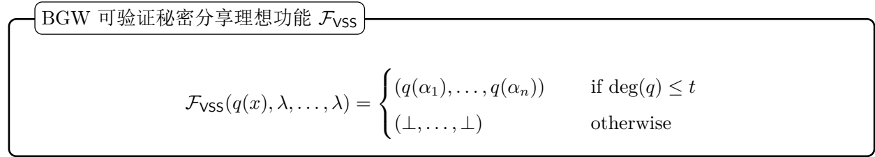
图 9.12: BGW 可验证秘密分享理想功能
