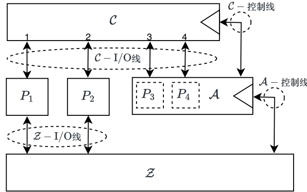
图 4.1: 真实协议运行，图中包括异步的安全信道 C ，敌手 \mathcal{A} ，环境 \mathcal{Z} ，诚实方 P_1, P_2 ，被攻陷方 P_3, P_4
