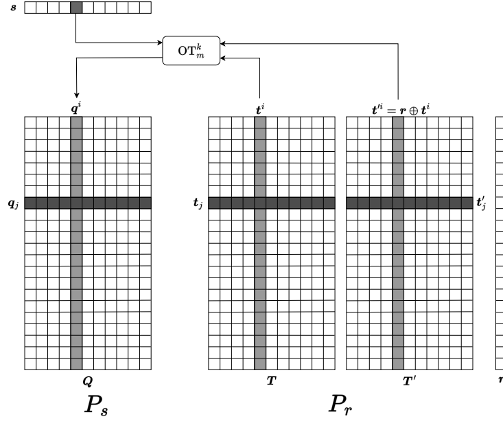
图 5.6: IKNP 协议示意图
