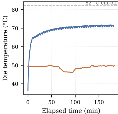
(b) Thermal trajectory
