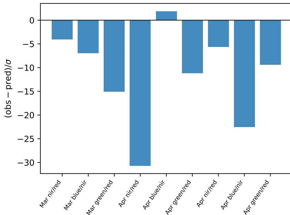
(d) Continuum bands
