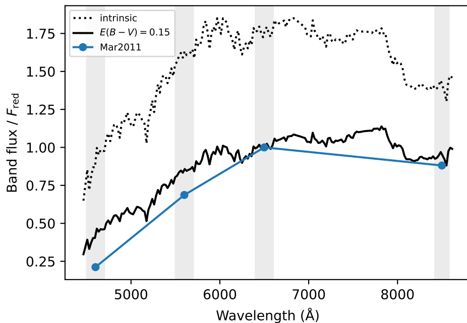
(d) Continuum bands
