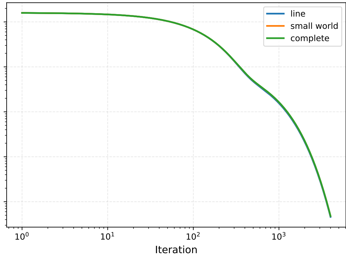
Gradient tracking
