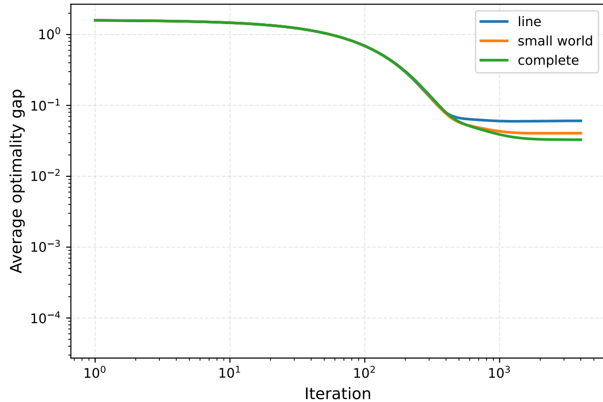
DGD
