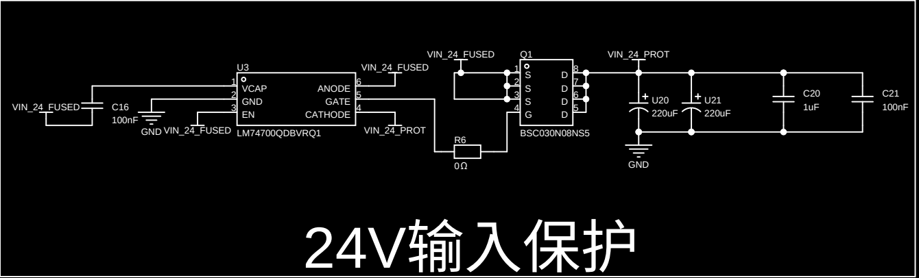
24V输入
