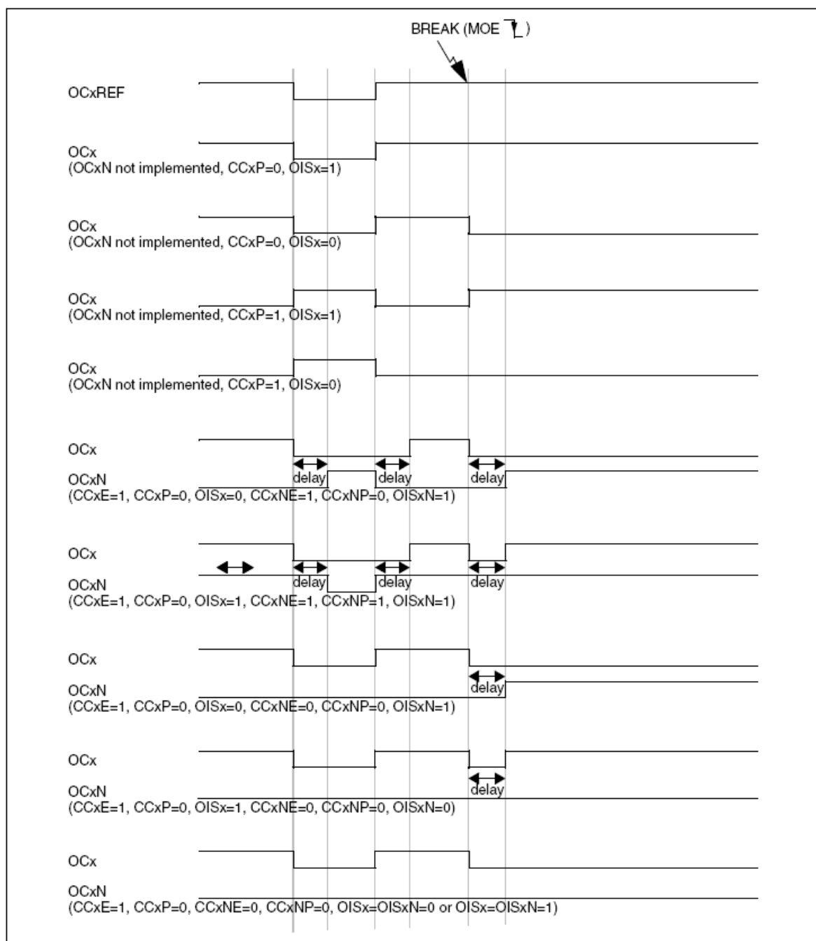
图83 响应刹车的输出
