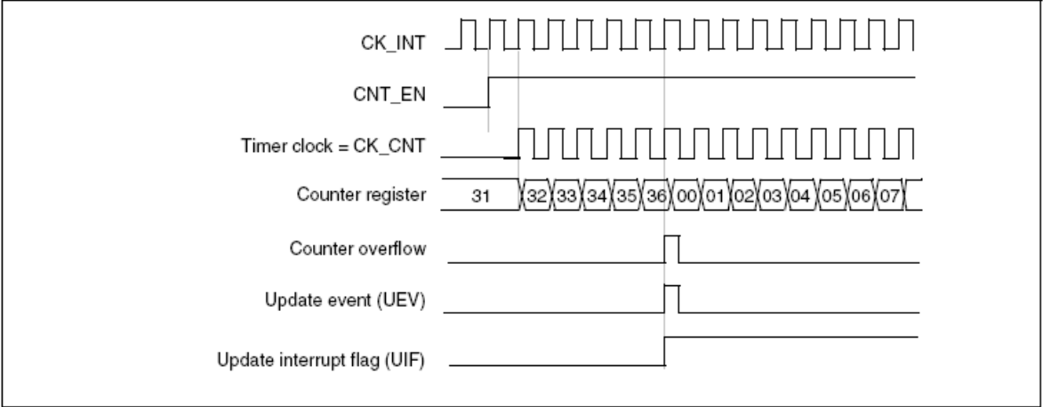
图143 计数器时序图, 内部时钟频率系数为1
