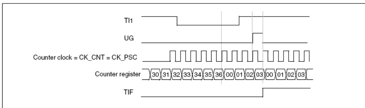
图130 复位模式下的控制电路
