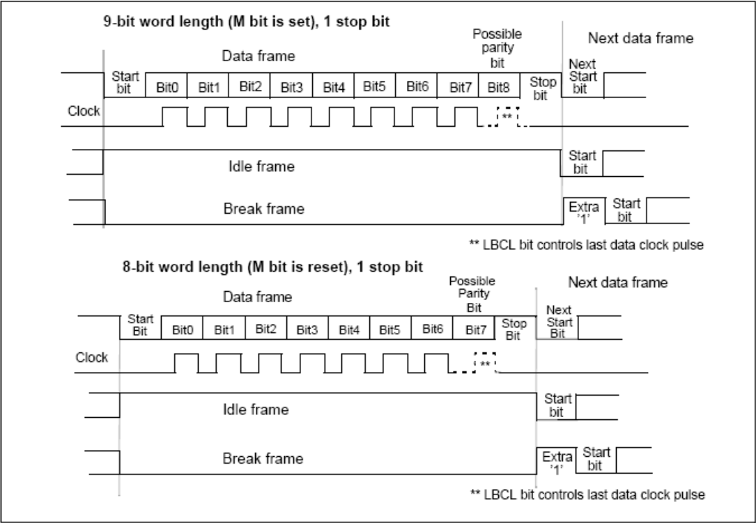
图237 字长设置
