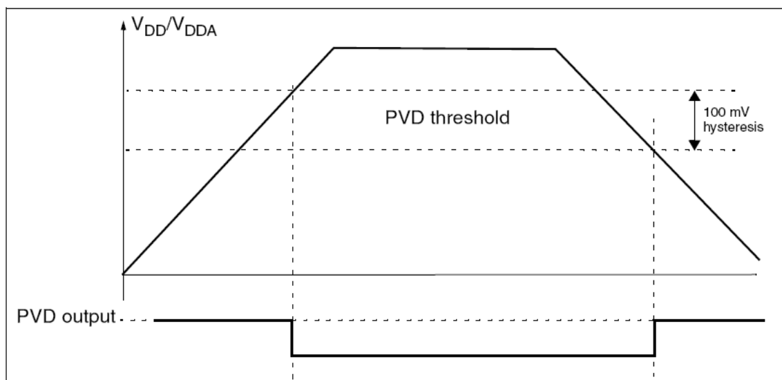
图5 PVD的门限
