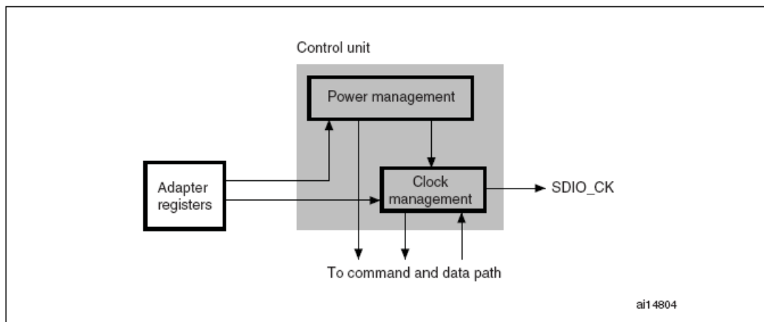
图182 控制单元
