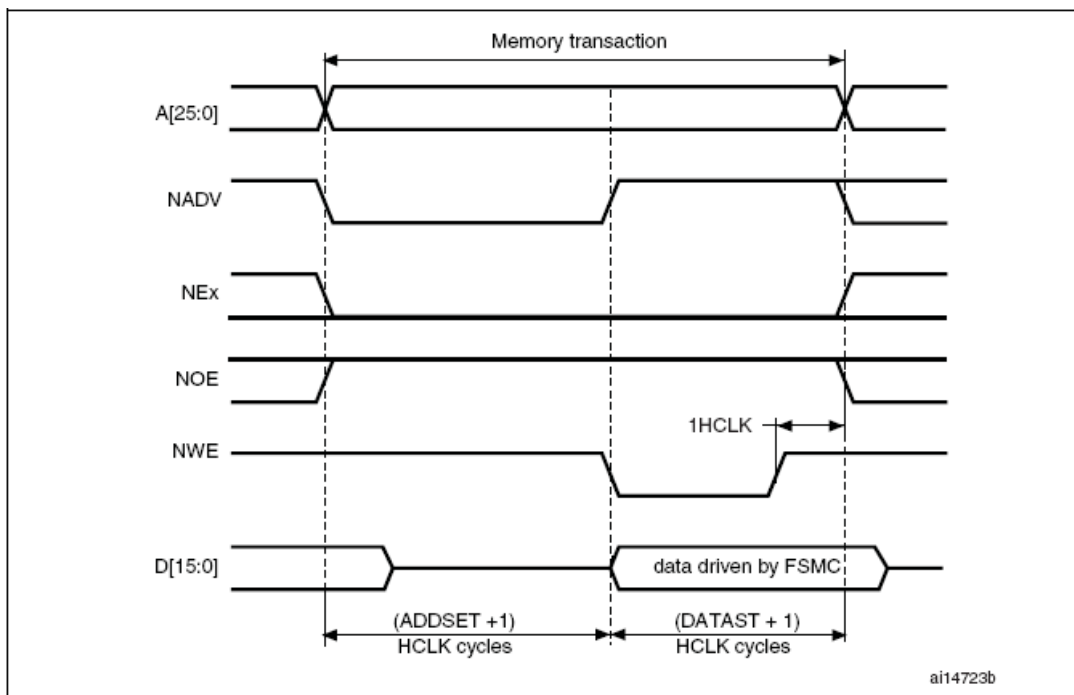
图163 模式2写操作
