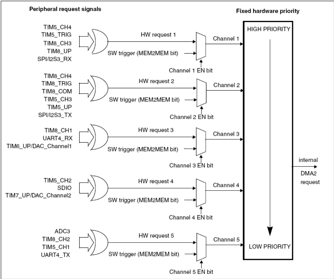
图19 DMA2请求映像
