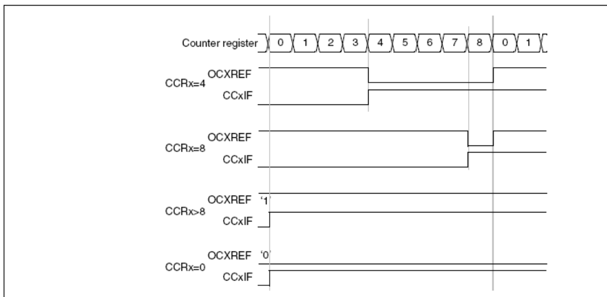
图78 边沿对齐的PWM波形(ARR=8)
