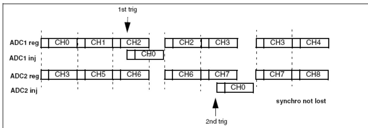
图34 交替+规则同步
