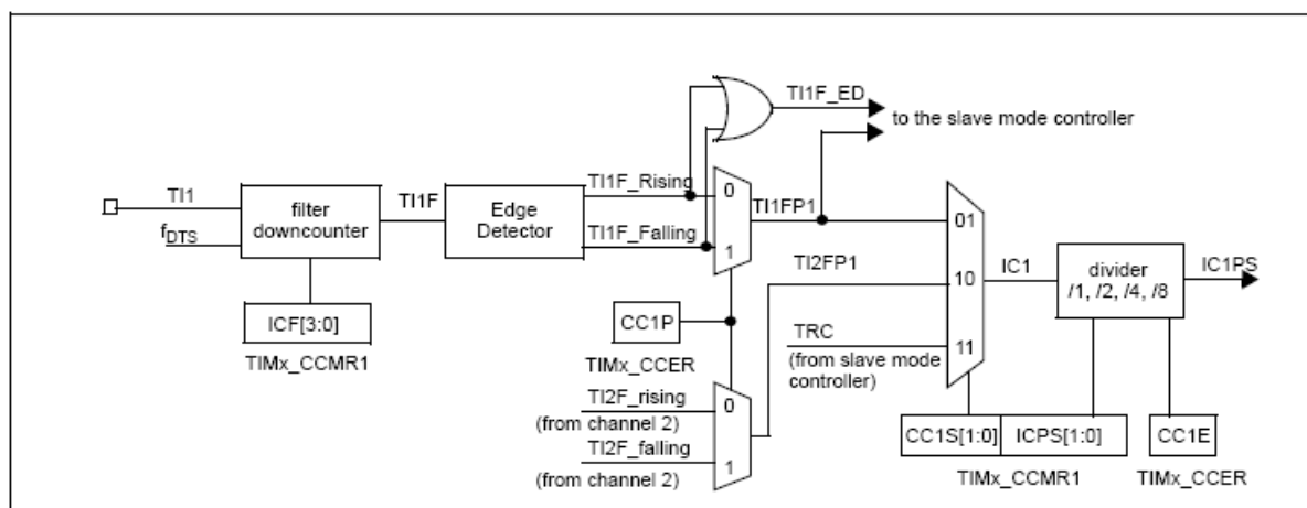
图72 捕获/比较通道(如: 通道1输入部分)
