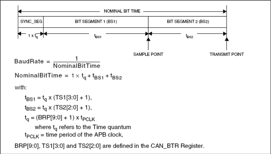
图202 位时序
