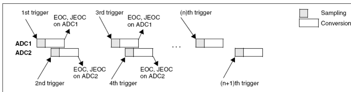
图32 交替触发：每个ADC1的注入通道组
