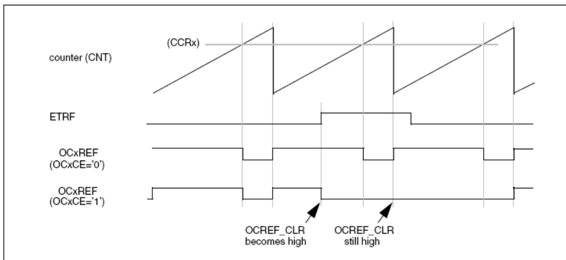
图84 清除TIMx的OCxREF
