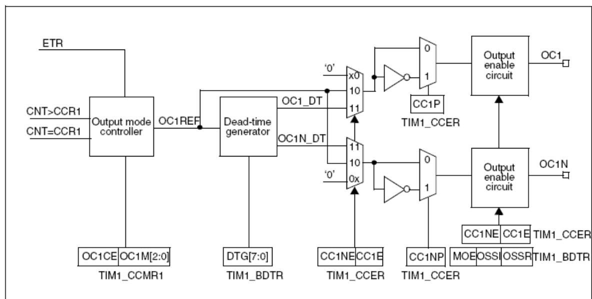
图74 捕获/比较通道的输出部分(通道1至3)
