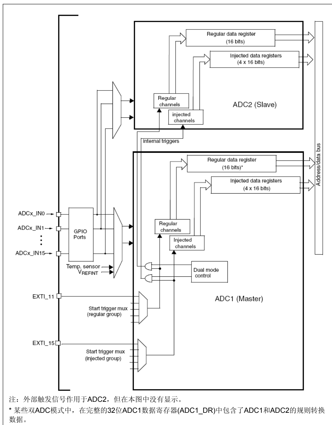
图27 双ADC框图
