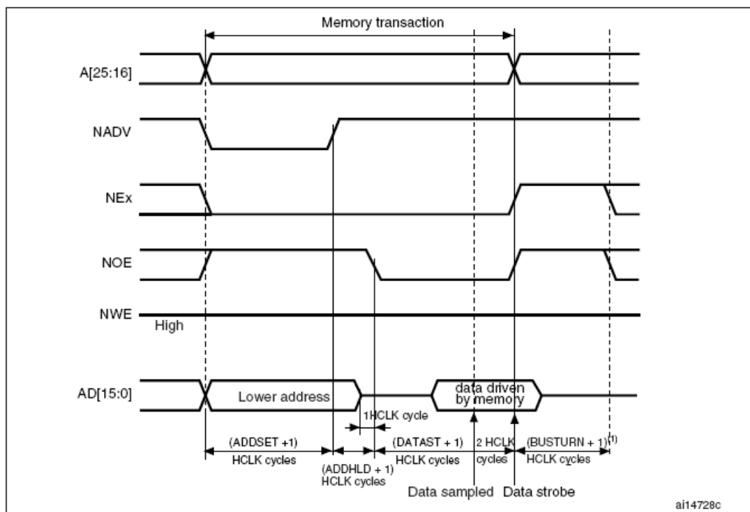
图169 复用读操作
