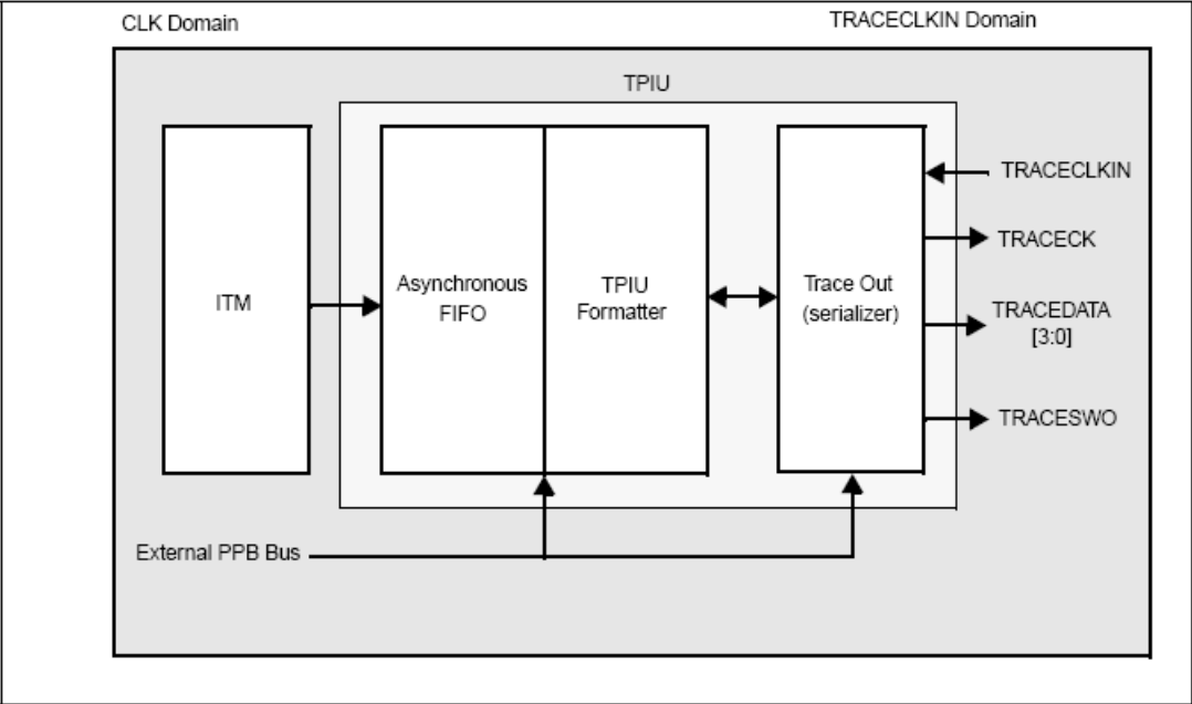
图260 TPIU框图
