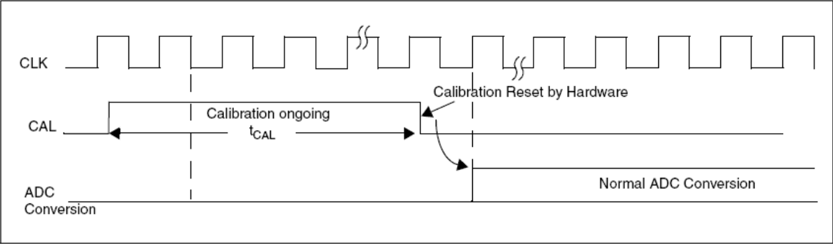
图24 校准时序图
