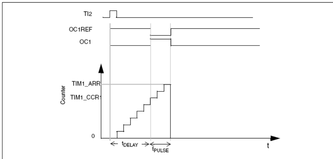
图126 单脉冲模式的例子
