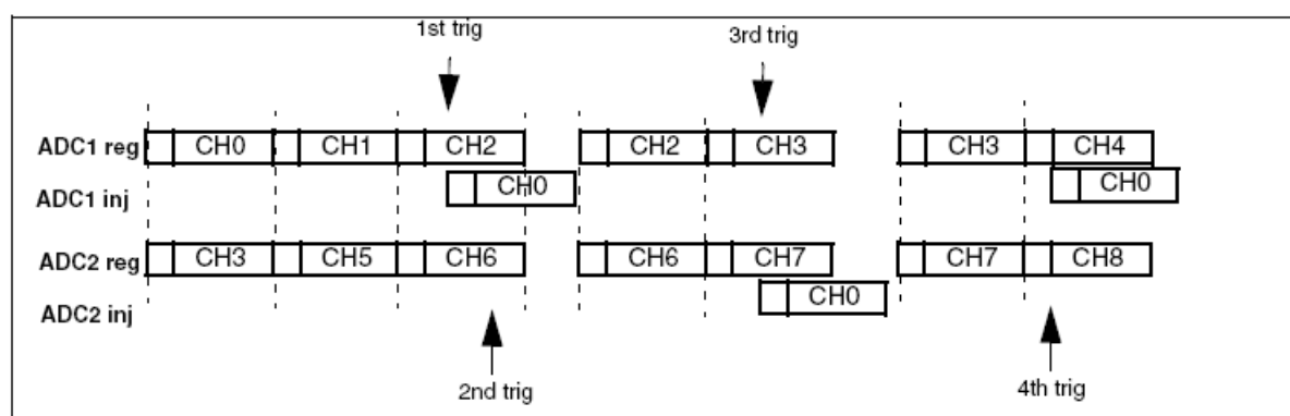
图35 触发事件发生在注入转换期间
