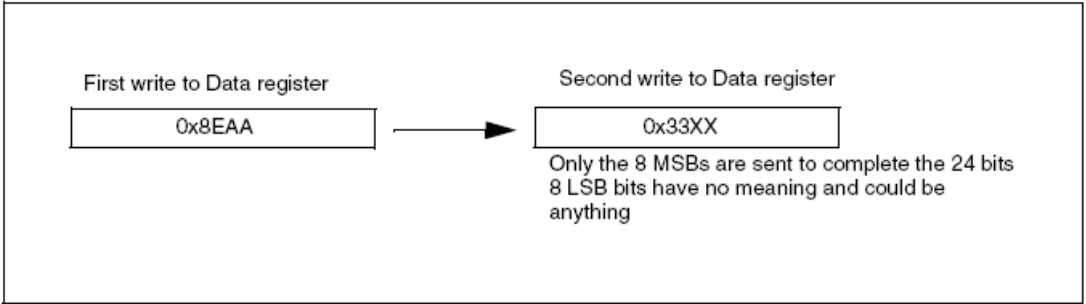
图212 发送0x8EAA33
