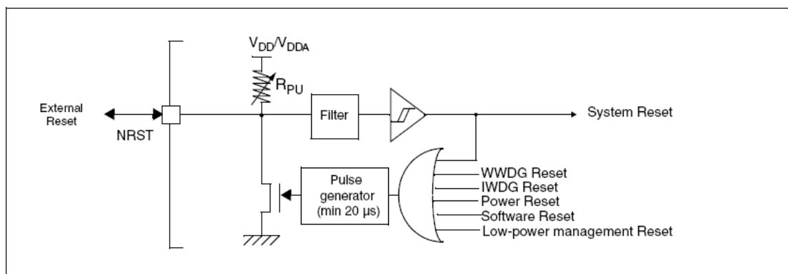
图6 复位电路
