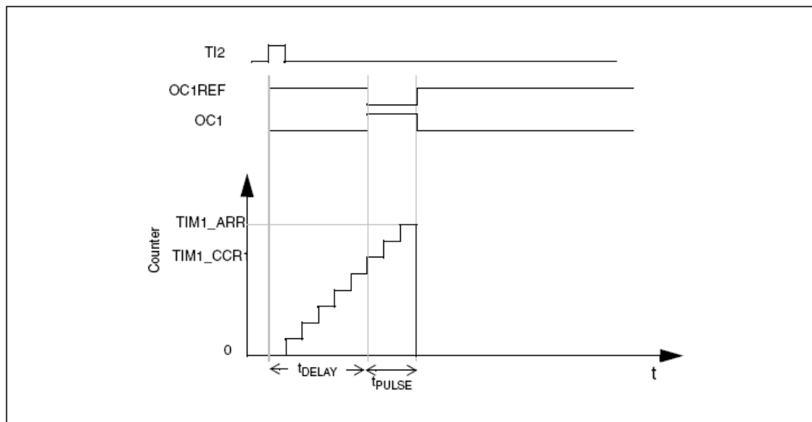
图86 单脉冲模式的例子
