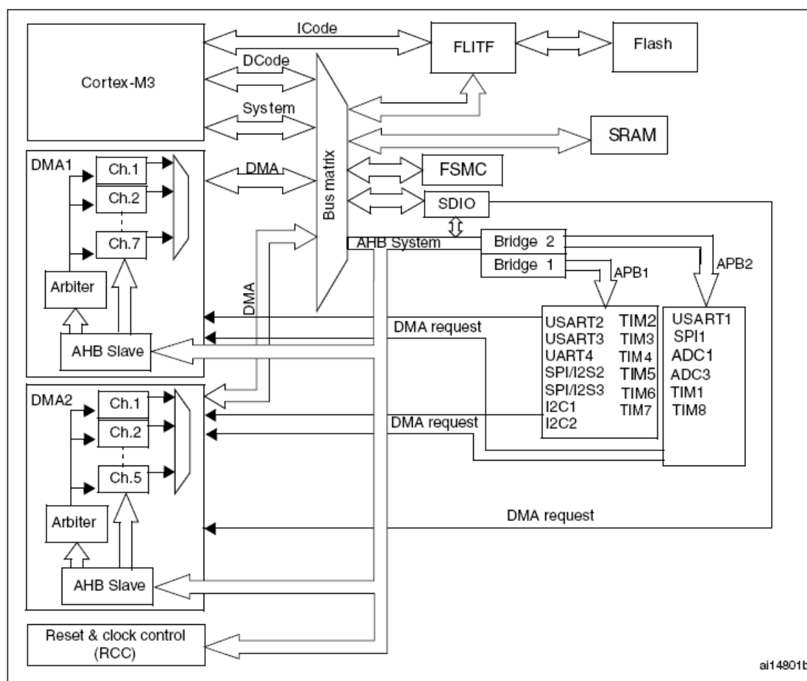
图17 DMA框图
