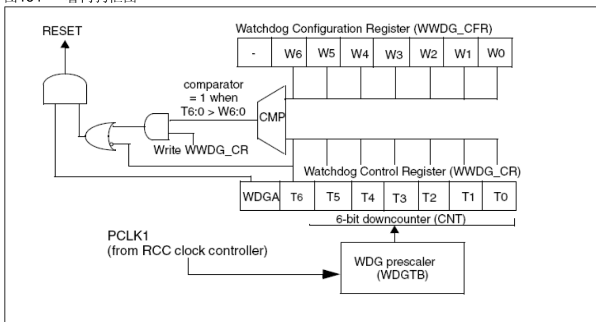
图154 看门狗框图
