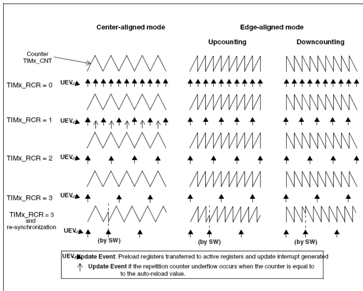
图66 不同模式下更新速率的例子，及TIMx_RCR的寄存器设置
