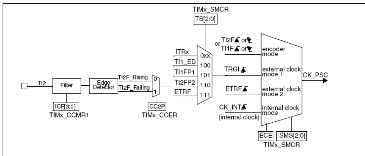
图68 TI2外部时钟连接例子
