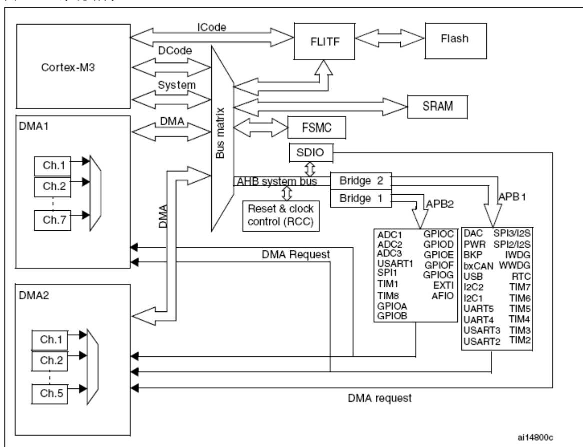
图1 系统结构
