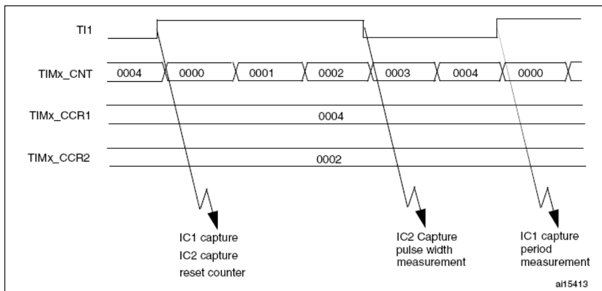
图76 PWM输入模式时序
