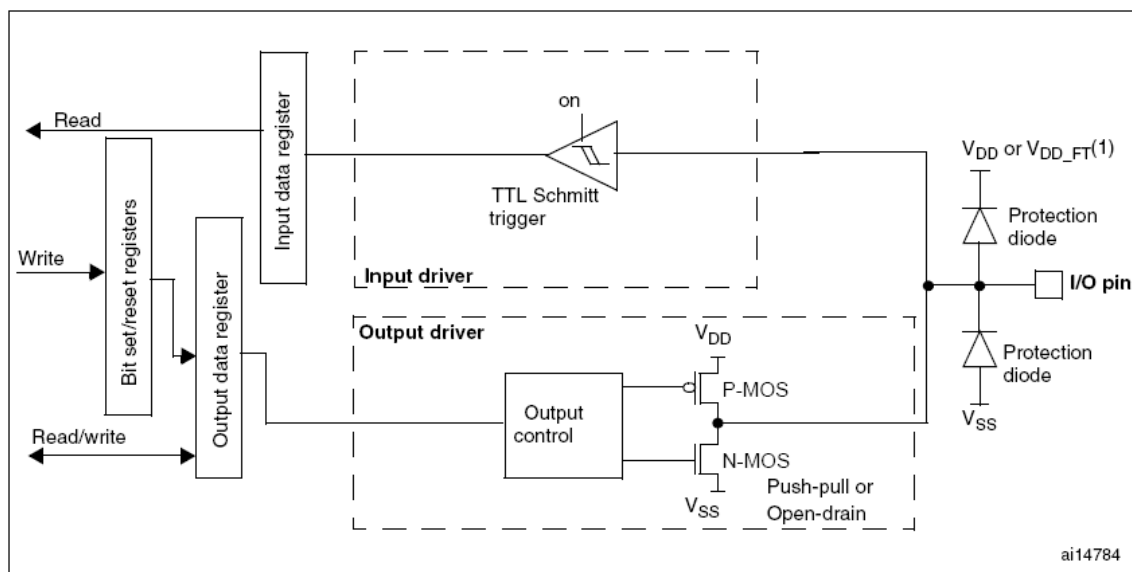
图12 输出配置
