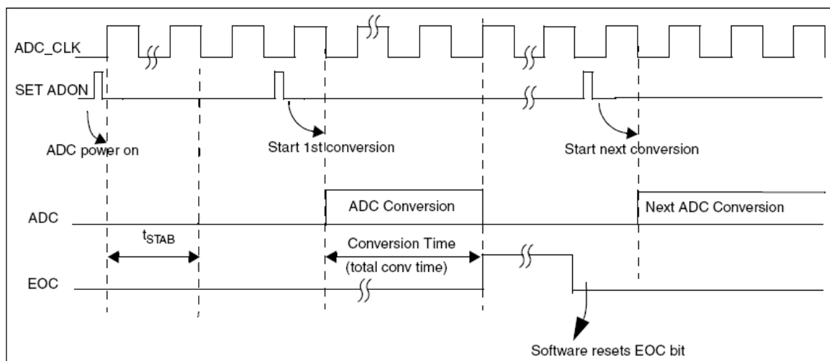
图21 时序图
