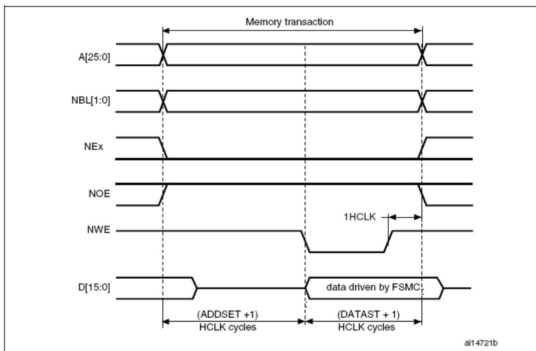
图159 模式1写操作
