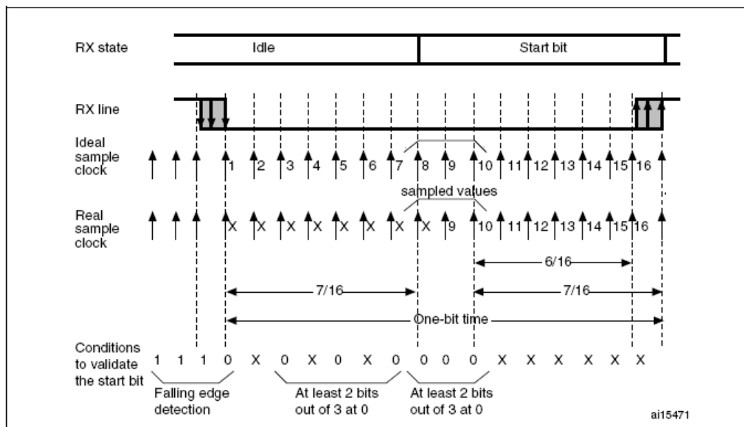
图239 起始位侦测
