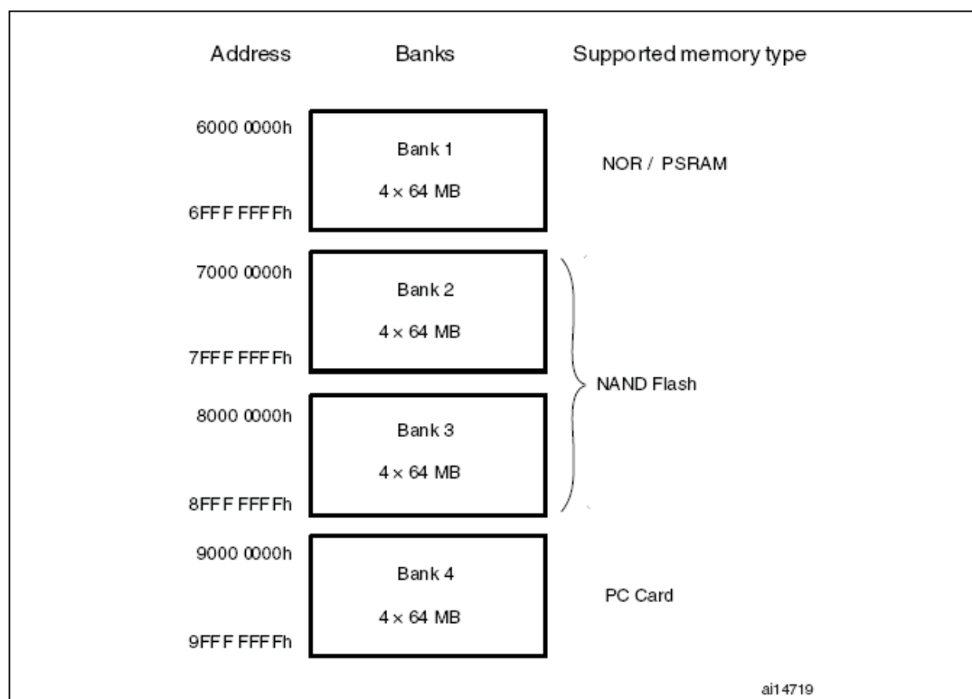
图157 FSMC存储块
