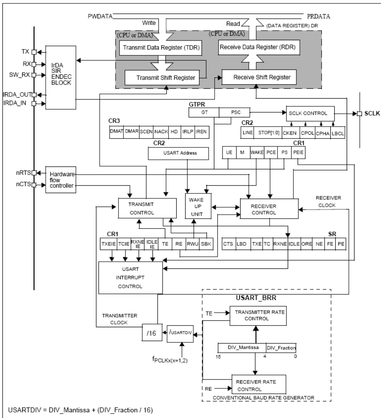
图236 USART框图
