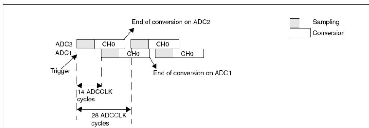
图31 在1个通道上的慢速交替模式
