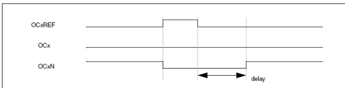
图82 死区波形延迟大于正脉冲
