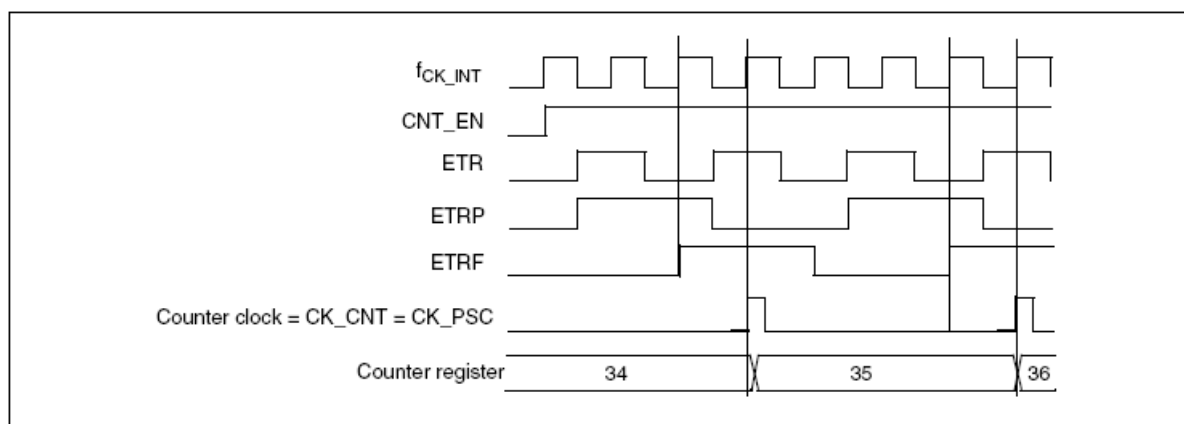
图71 外部时钟模式2下的控制电路
