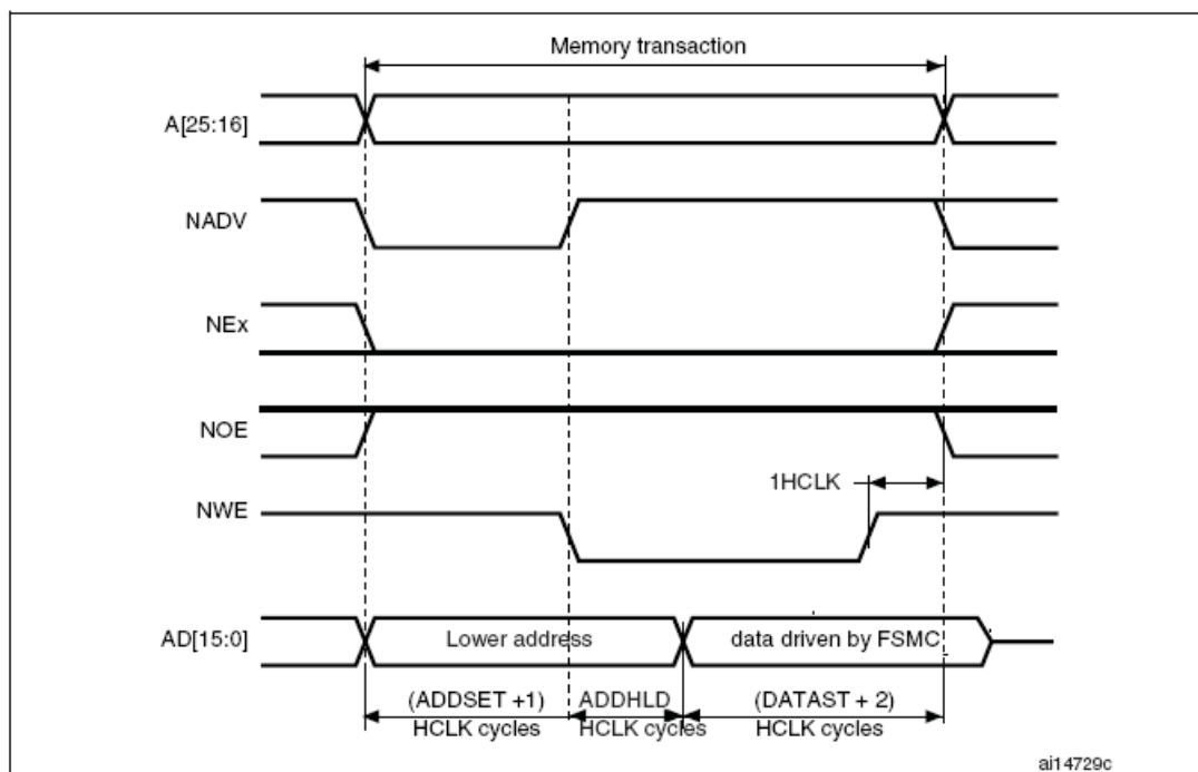
图170 复用写操作
