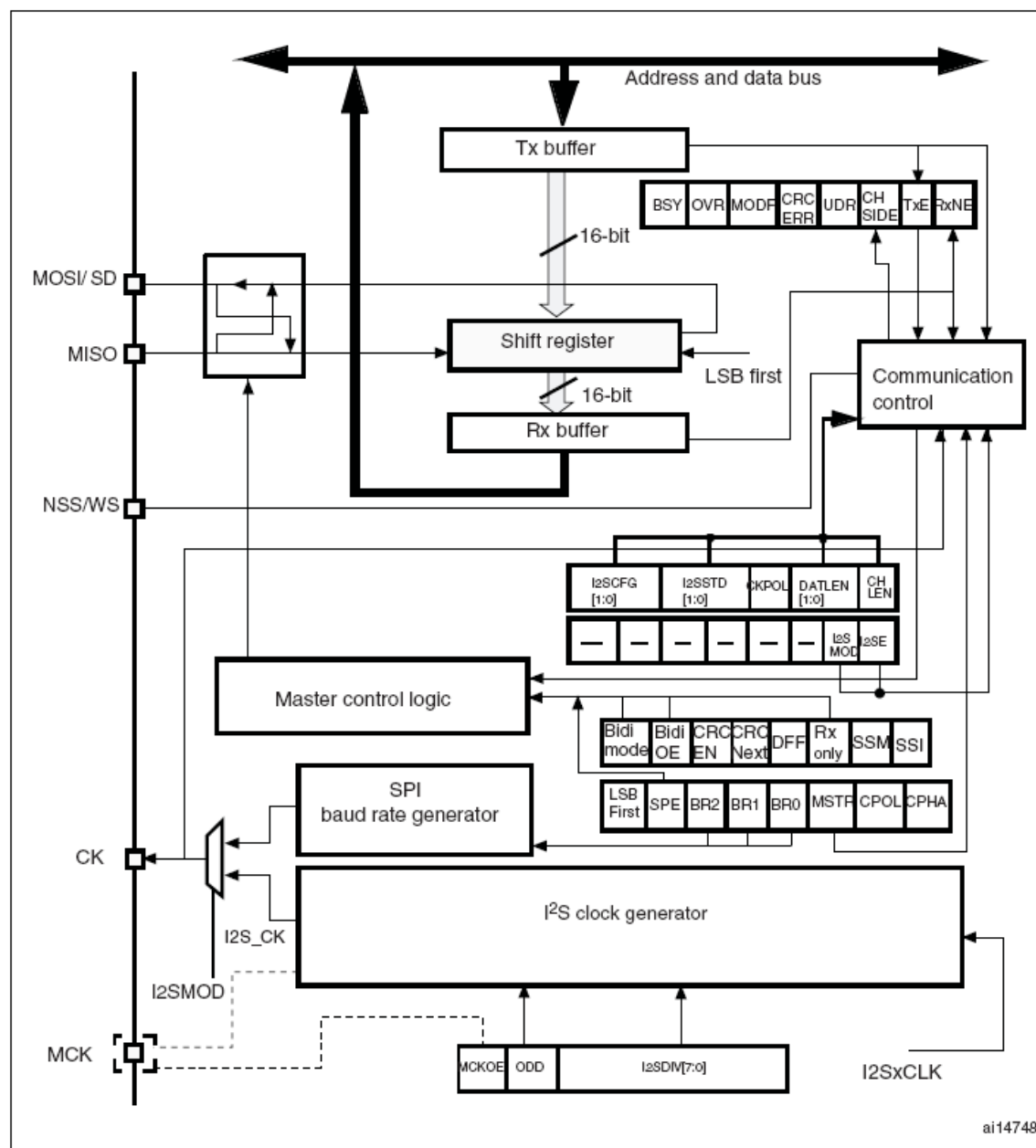
图209 I^2S 框图
