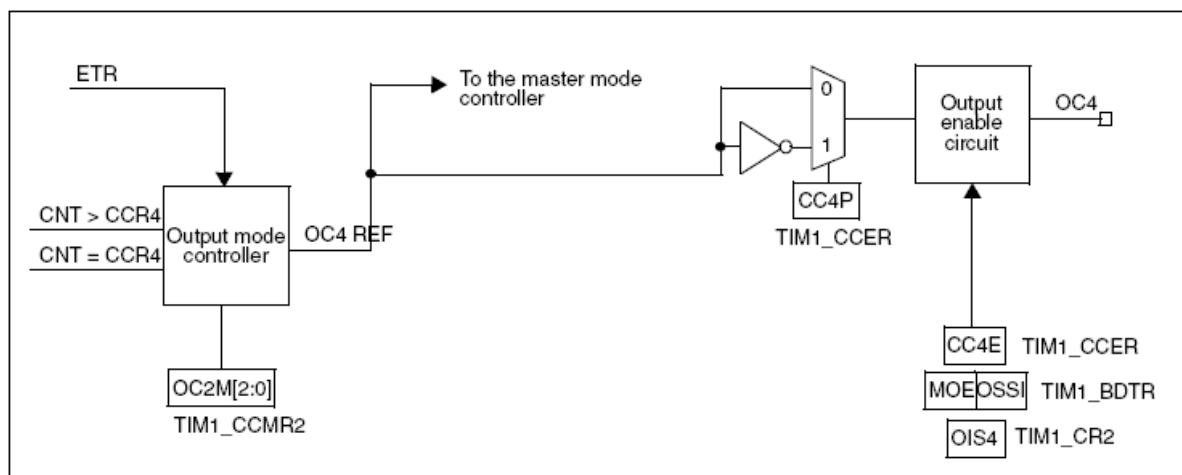
图75 捕获/比较通道的输出部分(通道4)
