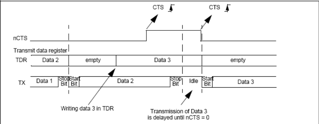
图255 CTS流控制
