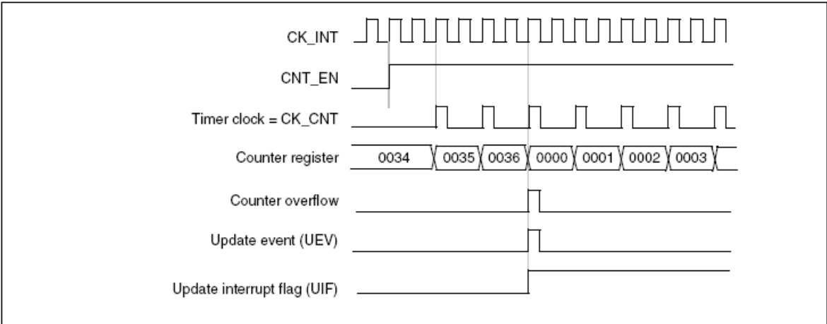
图145 计数器时序图，内部时钟分频系数为4
