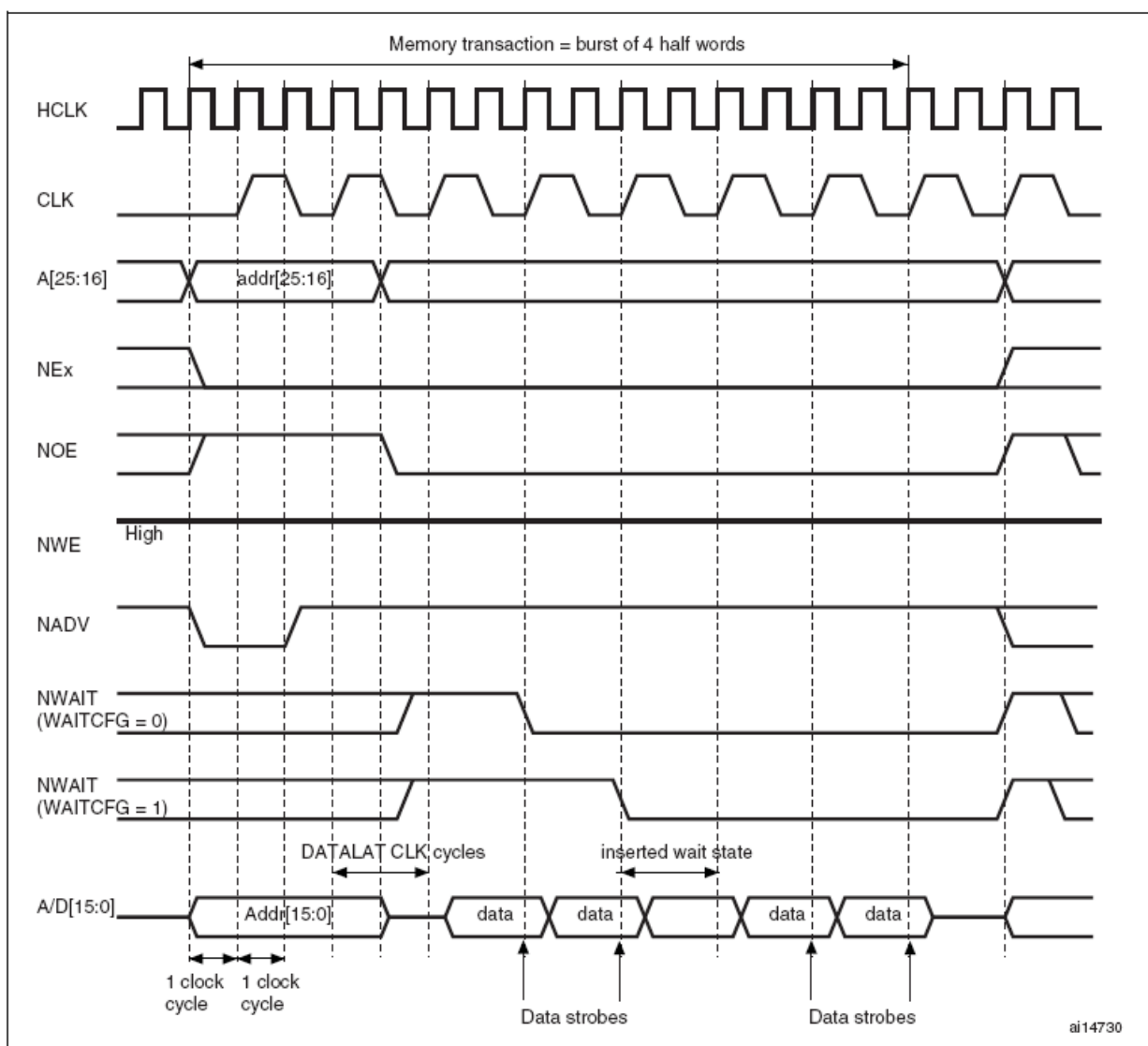
图171 同步读模式 – NOR, PSRAM(CRAM)
