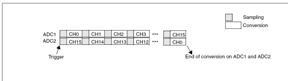
图29 在16个通道上的同时规则模式
