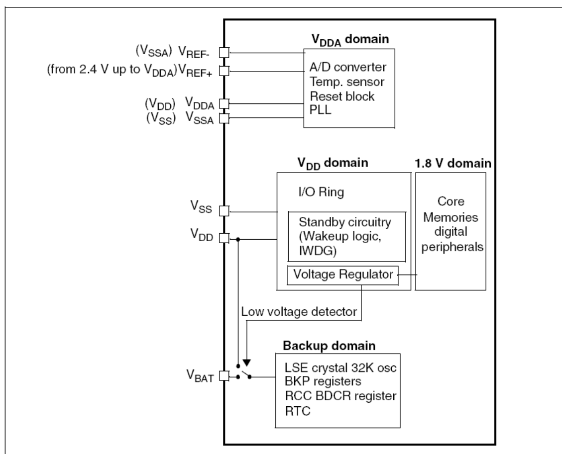
图3 电源框图
