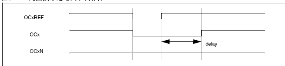
图82 死区波形延迟大于正脉冲
