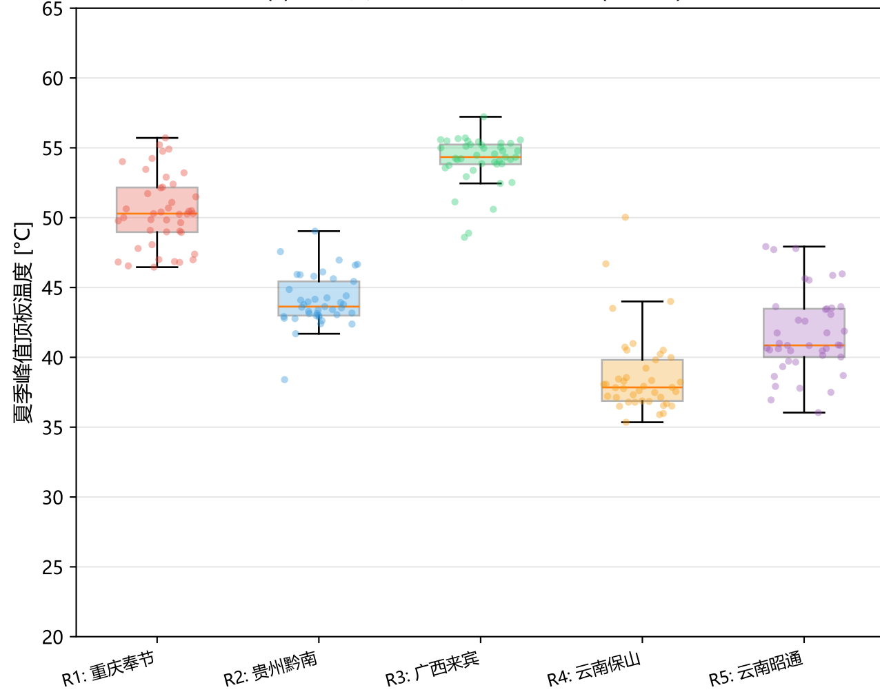
(a) 207 桥夏季峰值顶板温度分布 (按区域)
