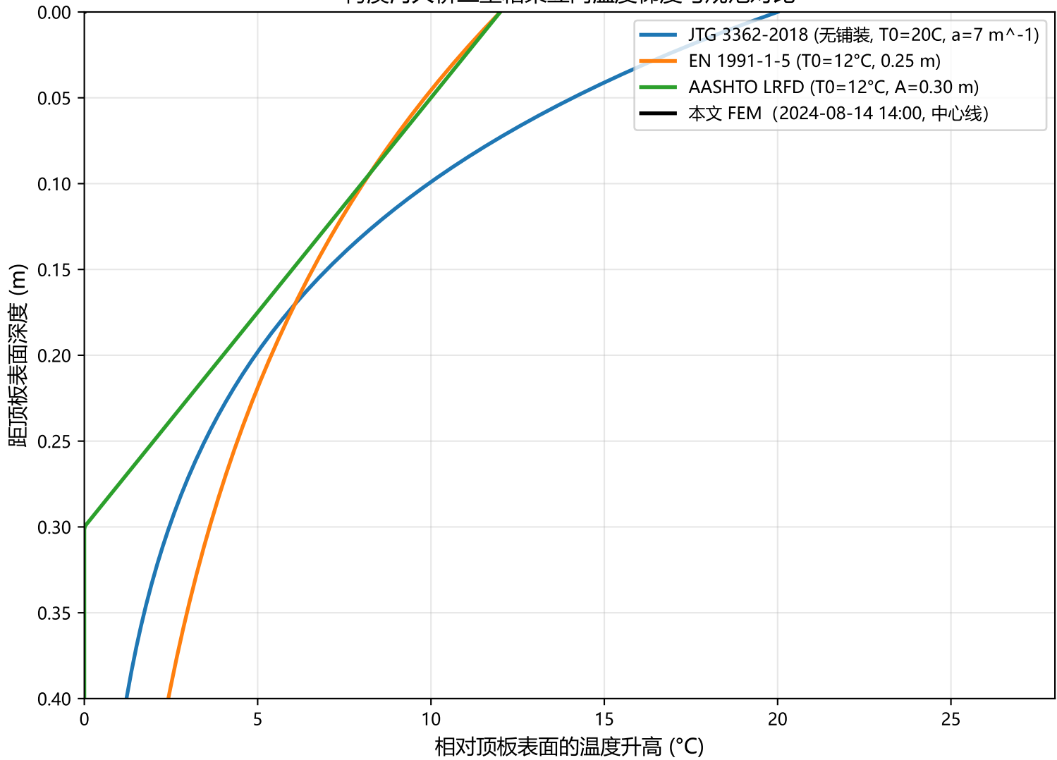
梅溪河大桥三室箱梁竖向温度梯度与规范对比
