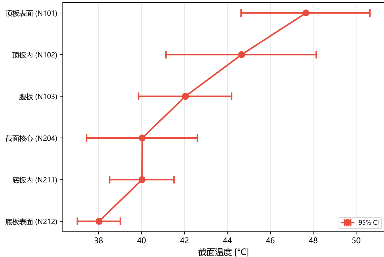
(b) M04 夏季峰值截面温度竖向分布及不确定性
