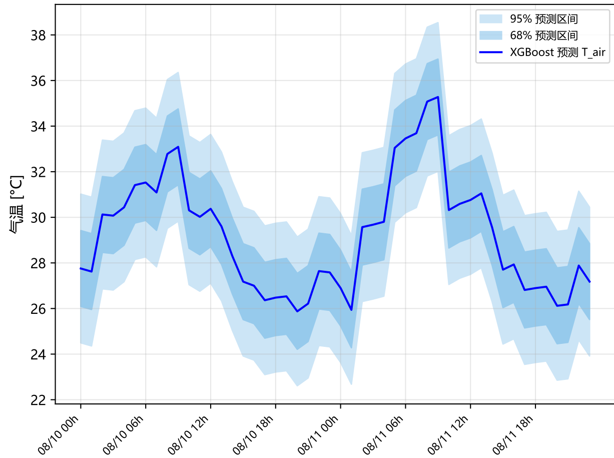
(a) M04 梅溪河大桥降尺度气温及预测区间
