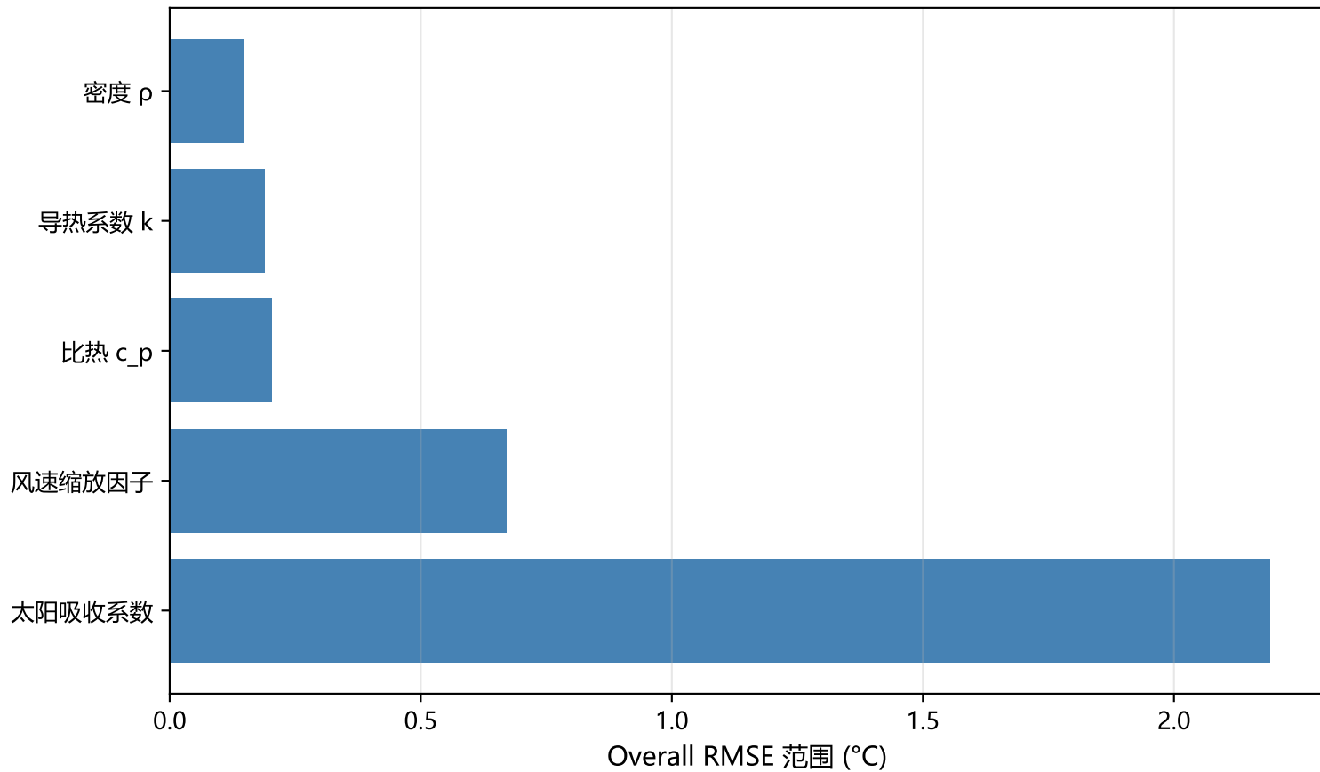
FEM 参数敏感性龙卷风图 (7 天连续晴天)
