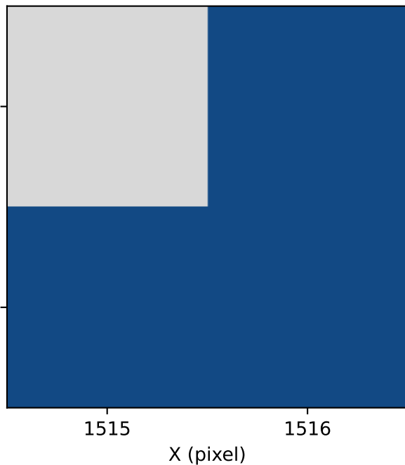
(b) Lower cloud: v_L
