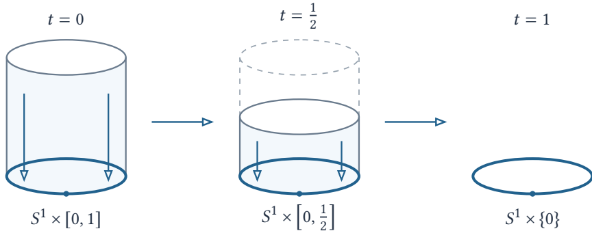
图 10 圆柱侧面的形变收缩. 三幅图画的是 H_t(X) ; 蓝色下边界始终固定, 圆柱不包含上下两个圆盘.
