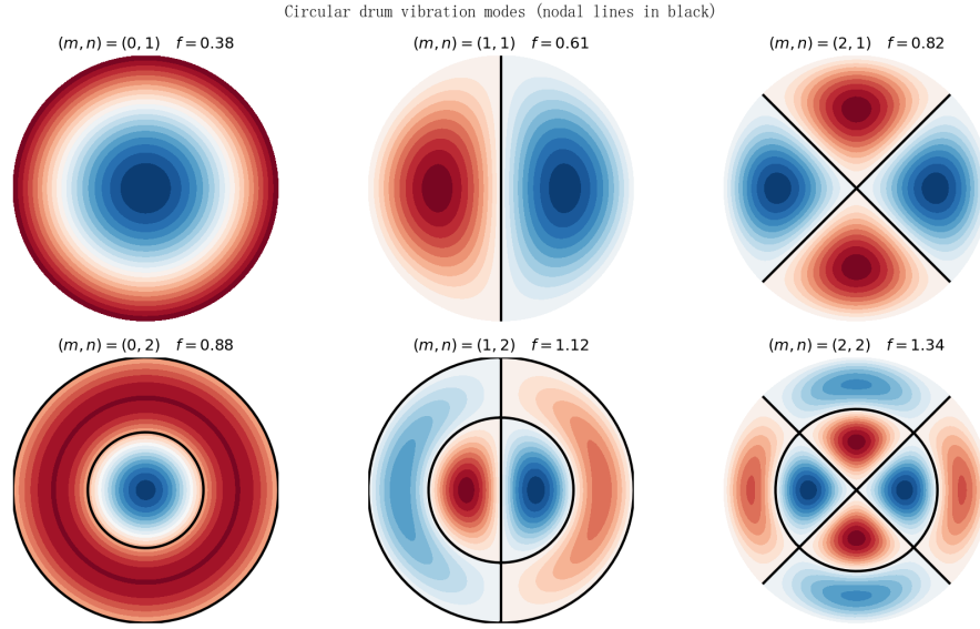
图 4.5: 圆膜的振动模式。颜色表示位移, 黑线为节线 (位移恒为零的线)。 (m, n) 中 m 为直径节线数, n 为环向节线数。频率 f 随 m, n 增大而增大。
