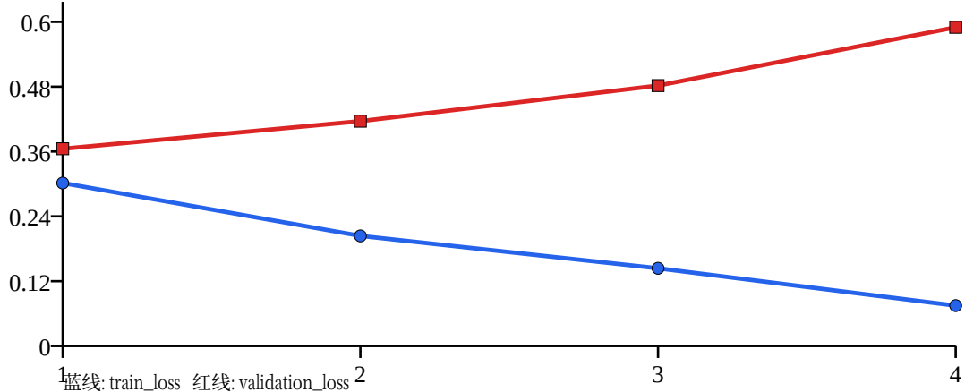
BiLSTM 训练曲线
