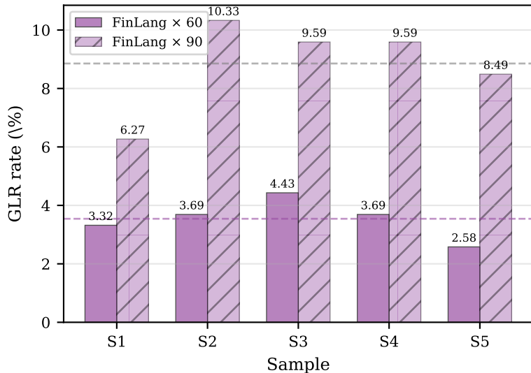
FinLang GLR per sample: 60 vs 90
