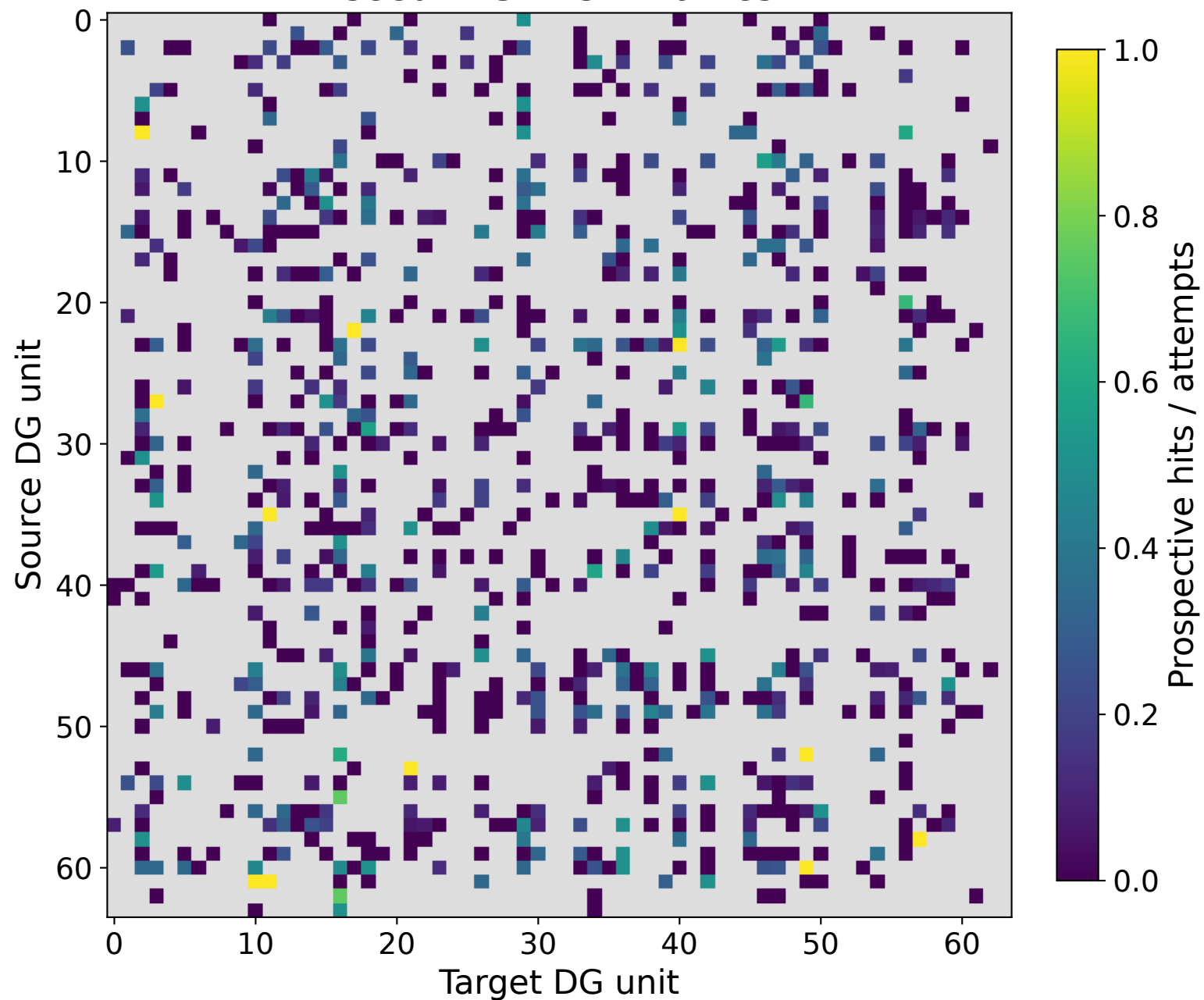
Waypoint F64 · DDQN+HER · cadence 2048 seed 123 · 25M frames
