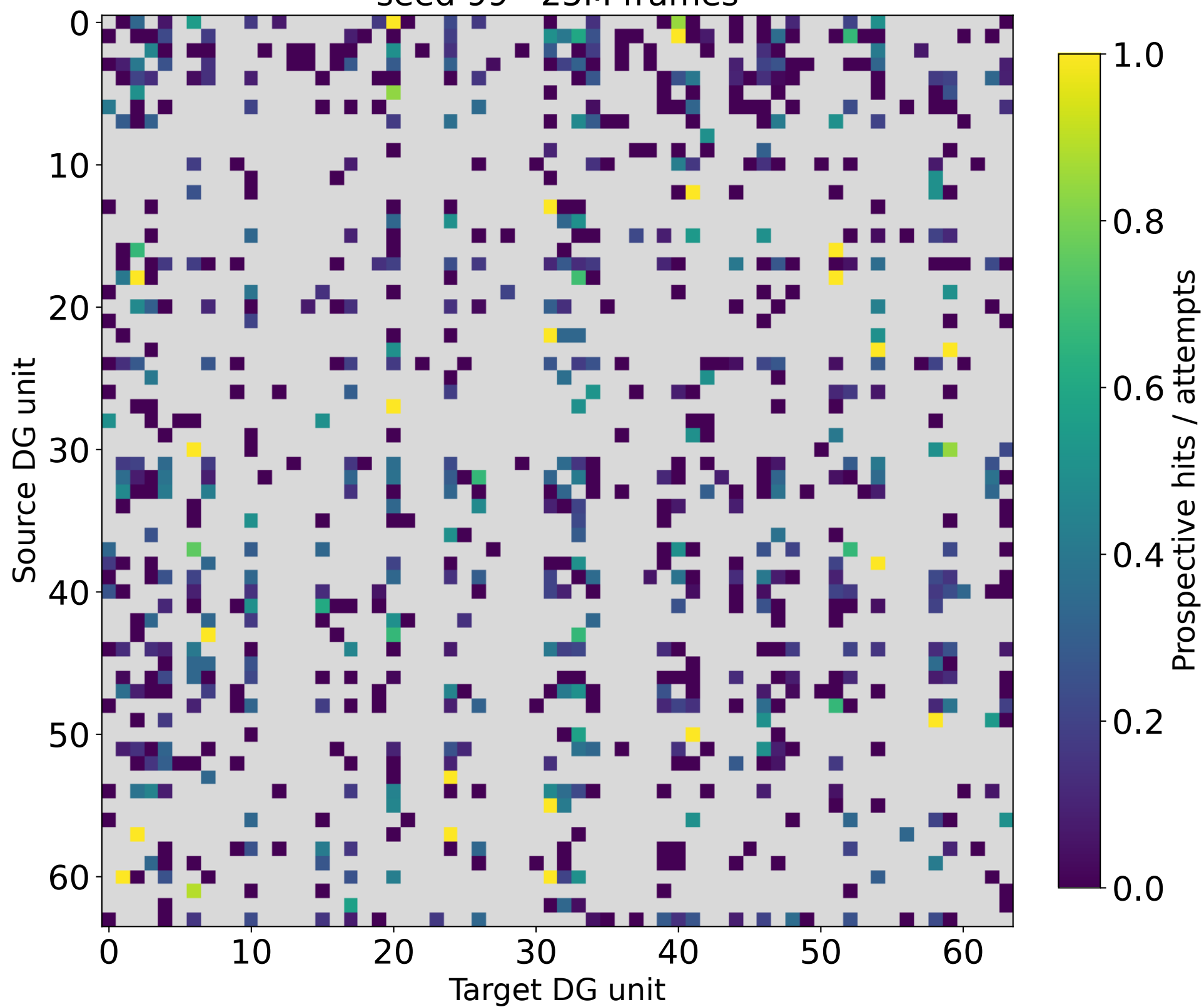
Waypoint F64 · DDQN · cadence 2048 seed 99 · 25M frames
