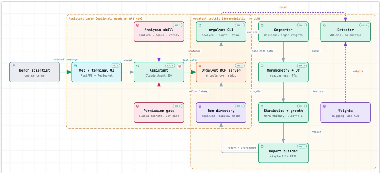
图 1a · 系统架构。用 archify 从代码仓库生成，每个节点都对应一个源码文件（节点右上角的 SRC 标记）。左侧虚线框是可选的助手层：界面、助手、分析技能与权限闸门；右侧虚线框是不依赖大模型的确定性工具包：命令行、分割器、检测器、形态计量与质控、统计与生长曲线、报告生成器，以及权重与运行目录。助手只能通过 MCP 服务器的六个工具进入工具包，命令行与助手走同一条代码路径，所以两种用法得到完全相同的数字。交互版（可点击节点查看上下游与源码）见 docs/orgalyst.architecture.html。
