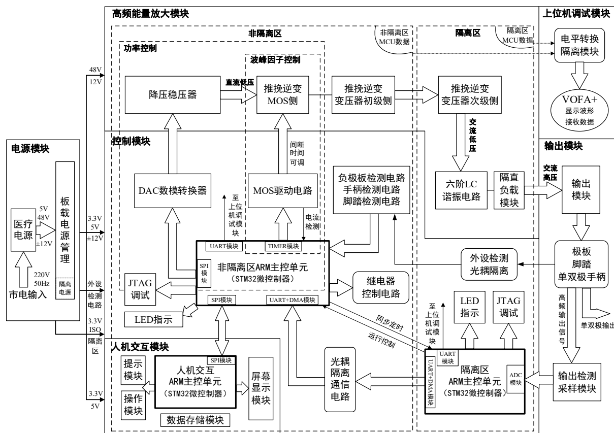
图 2-1 系统整体方案设计
