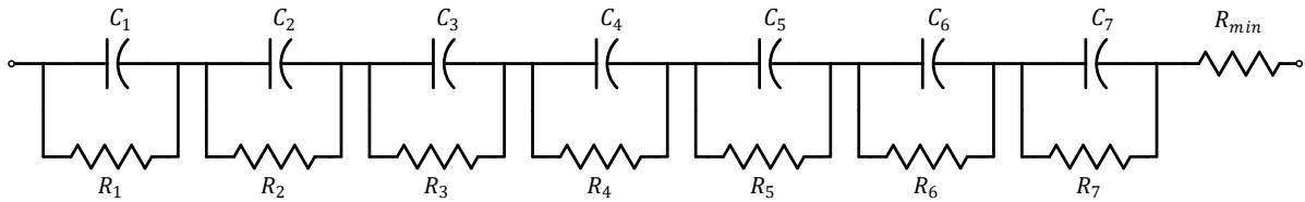
图 2-5 七元件级联生物组织阻抗模型
