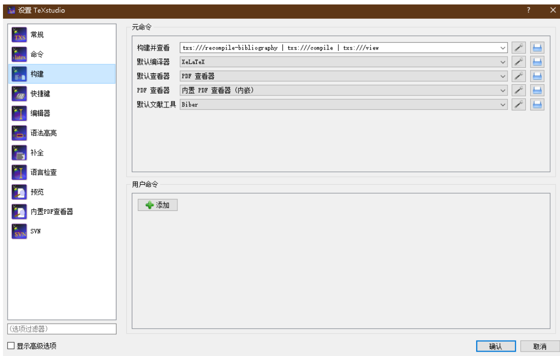
图 2-9 TeXstudio 环境
