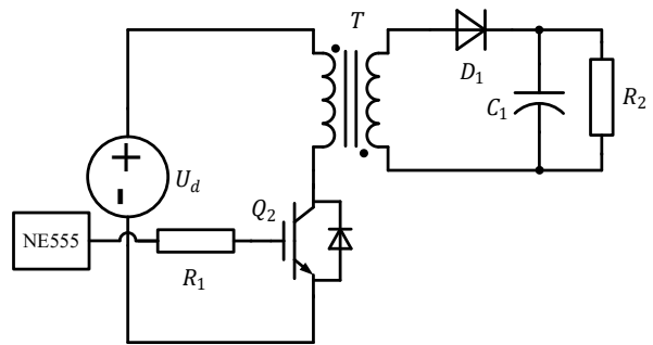
图 3-2 反激变换器拓扑结构
