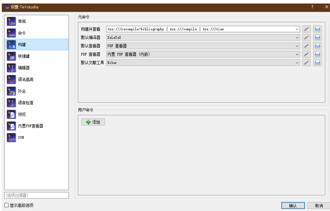
图 2-10 TeXstudio 环境
