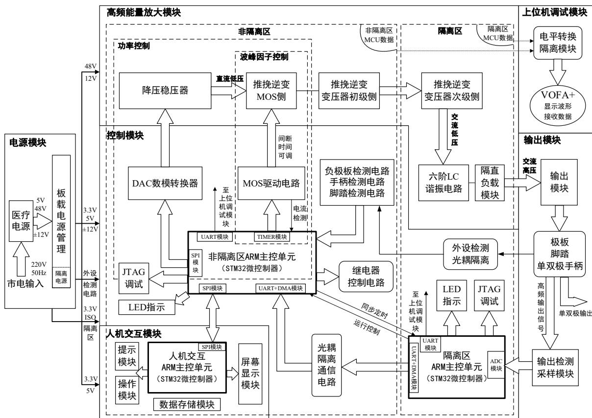
图 2-9 系统整体方案设计
