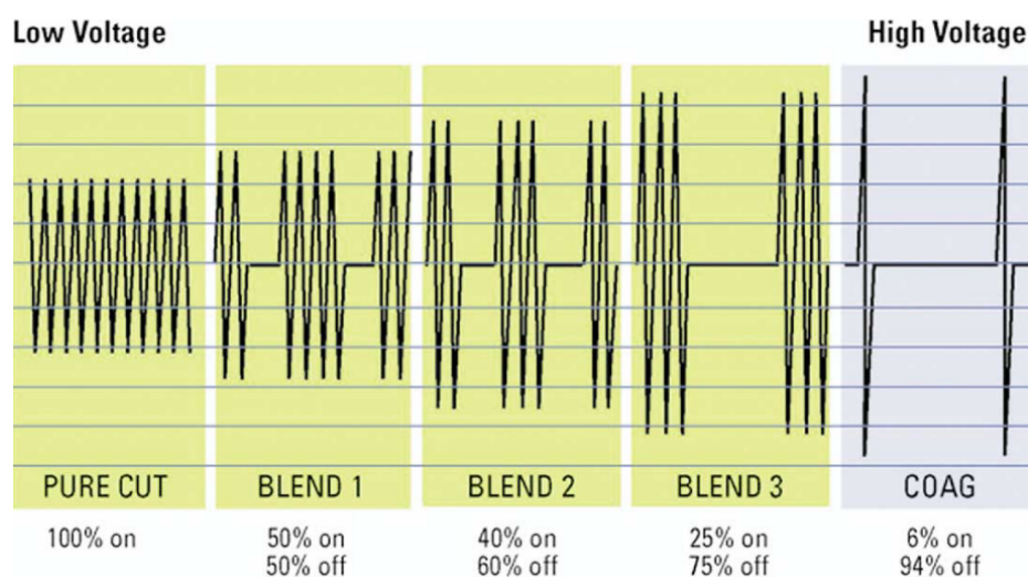
图 2-2 不同波峰因子的输出波形 [1]
