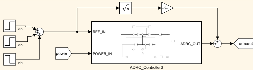
功率闭环控制器
