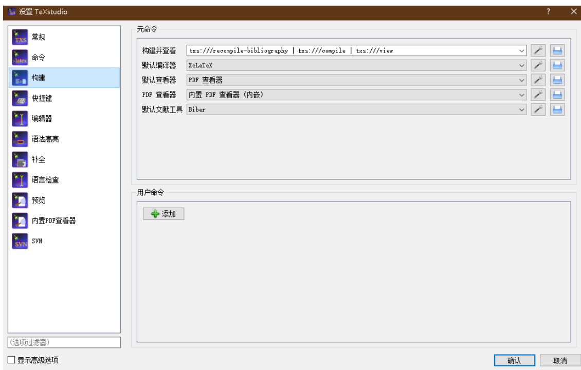
图 2-15 TeXstudio 环境
