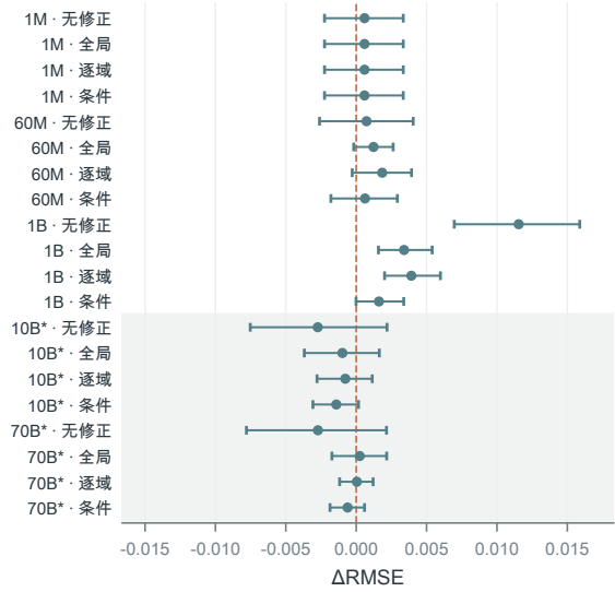
c 二阶 ilr-Ridge · RMSE
