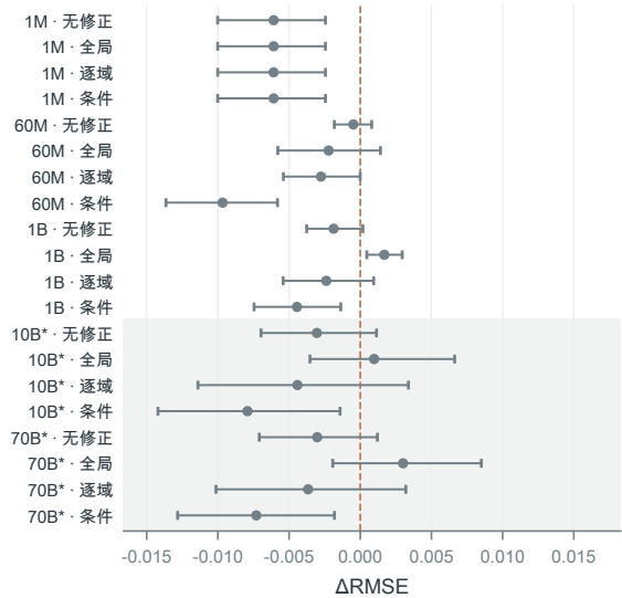
a 线性 ilr-Ridge · RMSE
