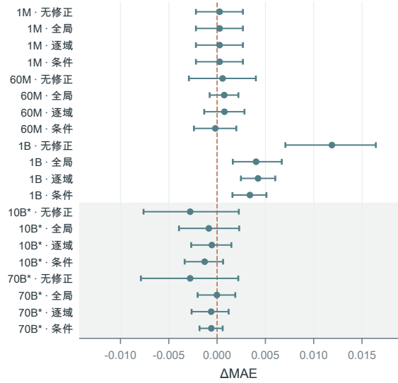
d 二阶 ilr-Ridge · MAE
