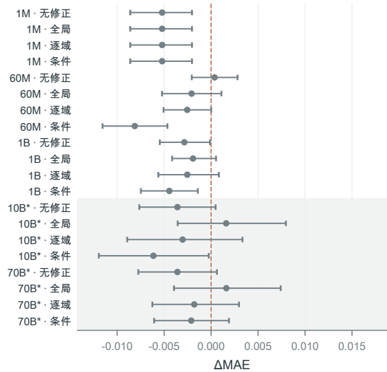
b 线性 ilr-Ridge · MAE
