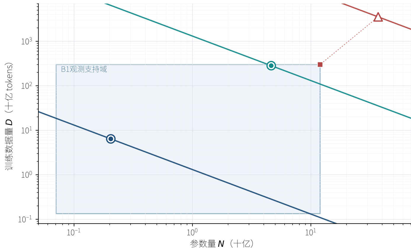
M0模型在预算约束下的N-D最优配置（上下文长度 L_{\text{ctx}} = 8192 ）
