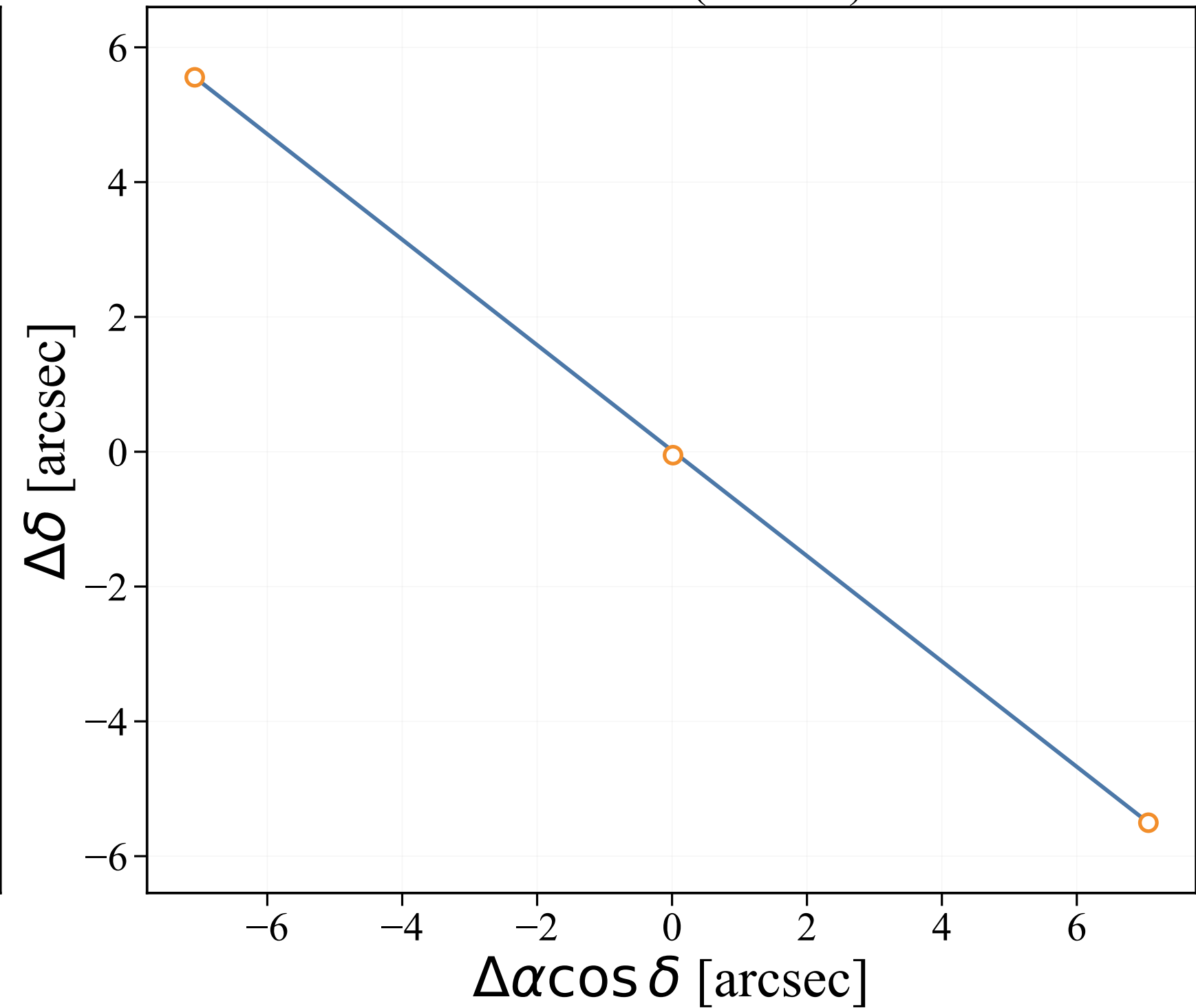
C/2025 Y1 (ATLAS)
