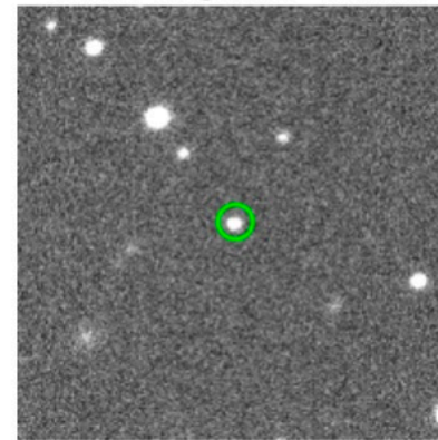
Eioneus magnitude = 16.7181
