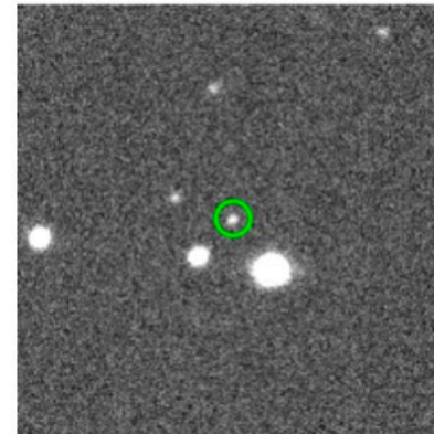
Fuchitatsu magnitude = 17.8154
