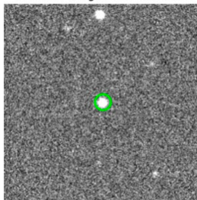
Naantali magnitude = 15.4042
