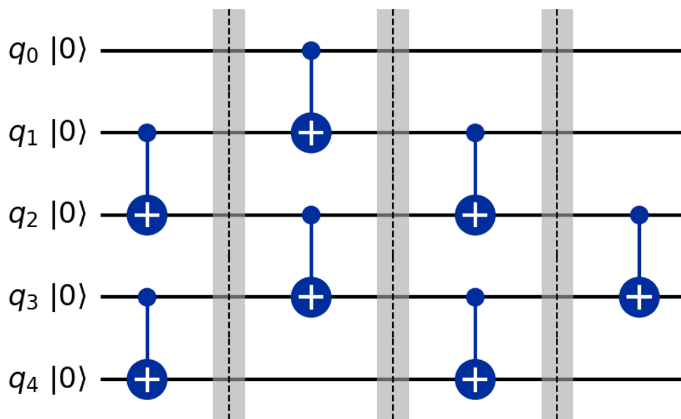
图 5: F_4 扇出的最优么正实现：7 个最近邻 CNOT，分 4 层（屏障分隔）并行，深度 4。
