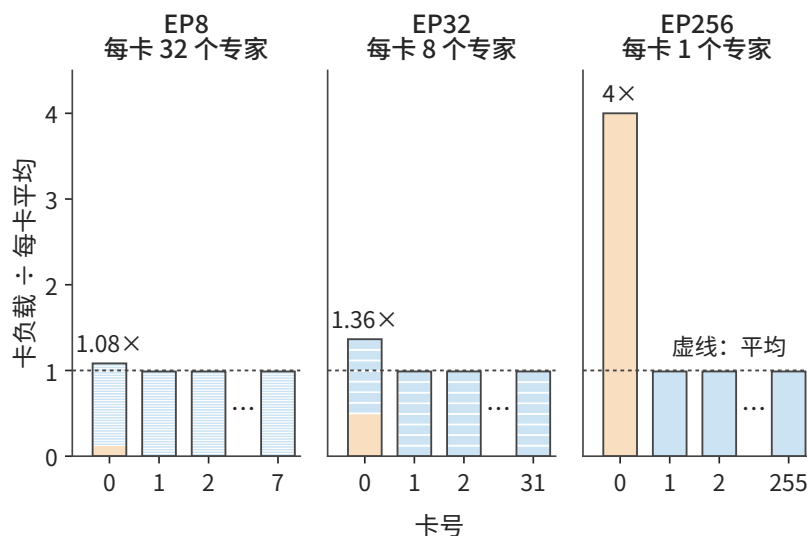
图 9-21：同一个热点专家在三种 EP 规模下造成的卡间 skew。256 个专家，1024 个 token 各选 8 个，专家 0 收到平均值 4 倍的 128 行。每根柱是一张卡，柱内每一段是这张卡上的一个专家，橙色为热点专家；纵轴为该卡行数除以每卡平均行数。每幅图只画卡 0、1、2 和最后一张卡，其余各卡与卡 1 相同。
