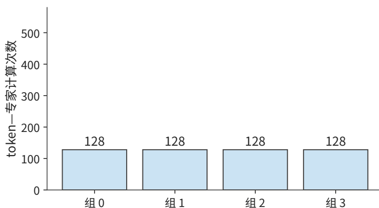
图 6-20：均匀使用 128 个专家时，四个 EP 组各处理 128 次 token—专家计算，合计读取 4.5 GiB 权重。
