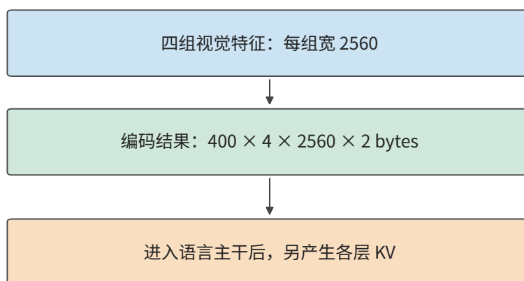
图 3-17 视觉 token 数与每 token 特征宽度分别计量。四组 2560 维 BF16 编码特征占 7.8125 MiB；这些视觉 token 进入语言模型后，另产生各层的 KV 状态。
