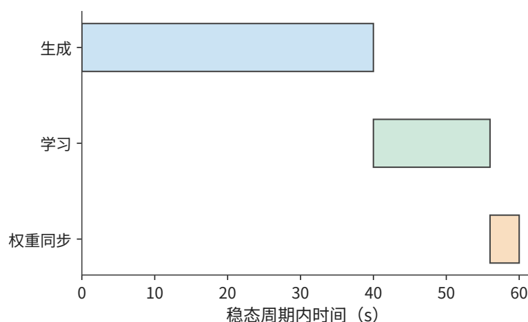
图 10-42：同步循环依次生成本批样本、学习本批样本、同步权重，分别用时 40、16、4 s，共 60 s。
