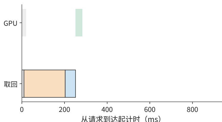
图 9-39：取回先查找 10 ms，再经 50 GbE 以 6.25 GB/s 读取 1.125 GiB 至主存，最后经 PCIe 以 25 GB/s 搬到 GPU。计算要等数据和 GPU 都就绪，首 token 约 282 ms 返回，比 A 慢约 1.6 ms。
