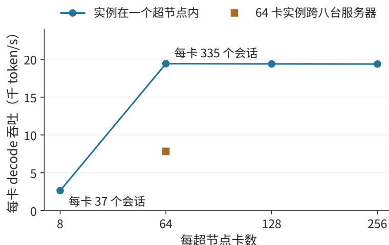
图 6-53: V4.1 Flash 在 256 张 H100 上的每卡 decode 吞吐随超节点大小的变化，服务目标为每 token 50 ms。蓝线：实例都在一个超节点内，8 卡到 64 卡提高约 7.4 倍，此后不再增长；橙点：同样 64 张卡分散在八台服务器上组成专家并行组。
