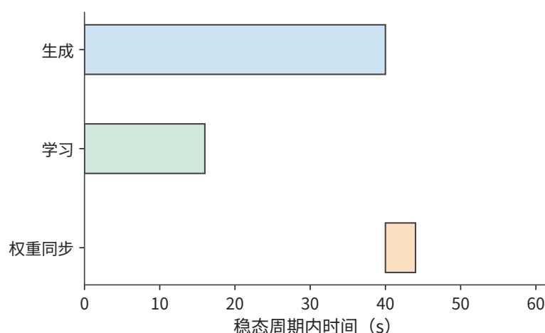
图 10-43：稳态中生成下一批与学习上一批在独立资源上重叠；两者完成后同步权重，周期为 44 s。橙色同步阶段阻塞两侧。
