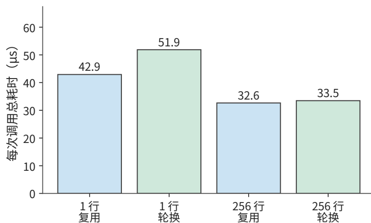
图 4-37 RTX PRO 6000 的投影总耗时。每个条件测十一轮、每轮十六次调用，取每轮平均耗时的中位数；计时包含提交与同步。“复用”表示多次调用读取相同权重地址；“轮换”表示调用之间更换权重地址。
