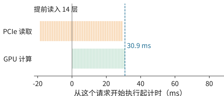
图 9-34：在这个请求开始执行之前，利用上一个 batch 的执行时间先读入前 14 层（448 MiB）；其余 22 层的读取被计算完全掩盖，总时间等于计算本身的 30.9 ms。三幅图的横轴相同。
