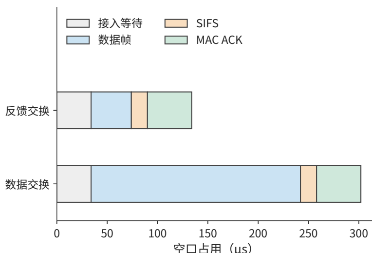
图 12-24：报文变短后，固定交换开销仍然存在，因此空口占用时间不会按相同比例缩短。两种成功交换采用相同的 34 μs 接入等待、16 μs SIFS、44 μs MAC ACK，区别只在数据 PPDU：208 μs 或 40 μs。条件为 OFDM54 / 6、无聚合、无重传的参考模型。
