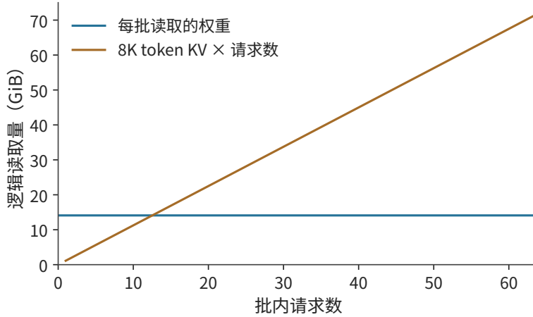
图 2-8 同一 batch 的主要投影权重可共享读取，各请求则各有一份上下文。图中固定每请求 8K 上下文，分别累计共享权重与独立 KV 的逻辑读取量。权重项按整个 decode batch 读取一次计量；KV 项累加各独立请求在本步读取的上下文状态。
