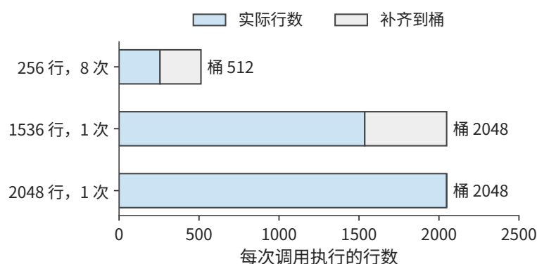
图 5-34：256 行的调用补齐到 512 行的桶，1536 行的调用补齐到 2048 行的桶，2048 行恰好落在桶的边界上。灰色部分是补齐后多算的行；10 次调用合计实际 5632 行，执行 8192 行。
