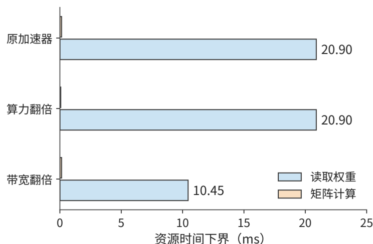
图 1-9 保持运算量与读取量不变，分别把算力或带宽翻倍。蓝条是权重读取下界，橙条是矩阵计算下界；较长的读取项决定这组条件下的优化方向。各柱分别表示计算或数据读取的时间下界，完整执行仍须满足依赖关系。
