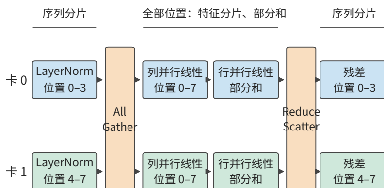
图 6-10: LayerNorm 和残差只用到本 token 的数据，两张卡各处理一半位置；进入列并行线性层前用 AllGather 收集全部位置，行并行线性层的部分和用 ReduceScatter 求和并重新按位置分片。
