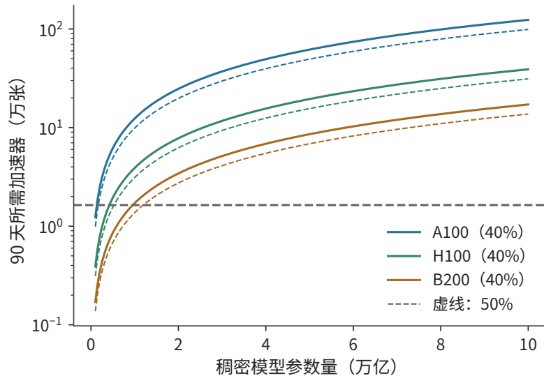
图 10-47：固定 90 天执行期限，稠密模型规模增大要求更多的卡。数据量为 20T token，算法工作为 6ND ，实线的 MFU 为 40%，虚线为 50%，使用 BF16 稠密矩阵峰值。各线为向上取整前的连续计算边界；横线标出 16,384 张卡。
