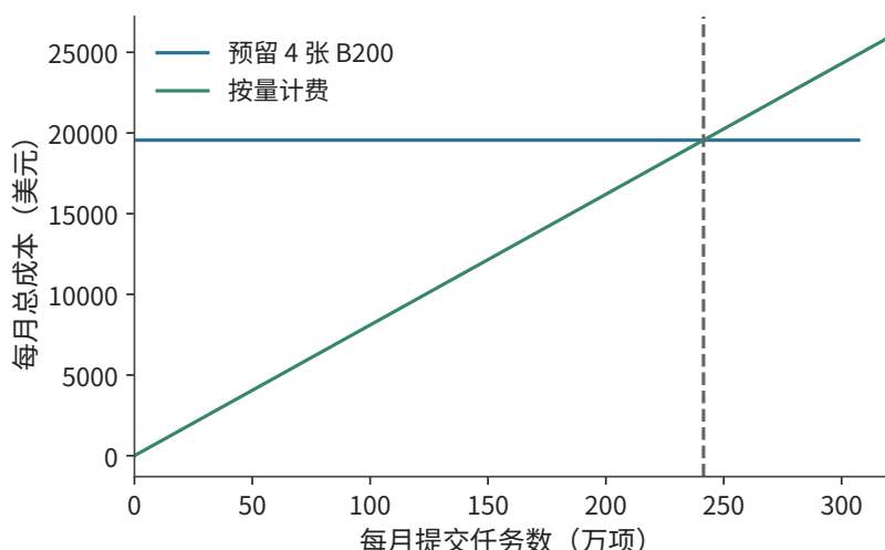
图 11-33：4 张 B200 预留一个月共 19,555.2 美元，按量成本为 0.0081N 美元，N 为提交任务数。两条线在约 241 万项相交，对应预留 GPU 约 78.6% 的利用率；预留线止于每月 307.2 万项的处理上限。
