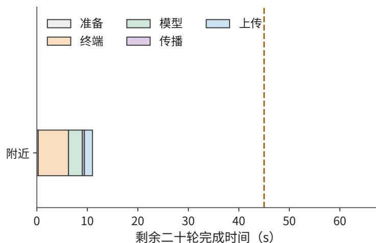
图 12-29：附近工作站 (RTX PRO 6000)：准备 0.27 s，二十轮终端 6 s、模型 2.7 s、传播 0.4 s、上传 1.6 s，共 11.0 s，满足 45 s 期限。虚线表示 45 s 完成期限。
