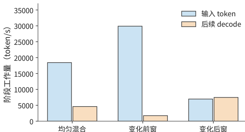
图 3-5 三个时间窗中，请求组成对应的输入与后续生成需求。输入数按 token 计，后续生成按每请求的一次 decode 步计；每请求首输出已计入 prefill。输入项统计每秒新处理的输入 token；decode 项统计所有请求每秒需要执行的后续 decode 步，每步推进一个 token。
