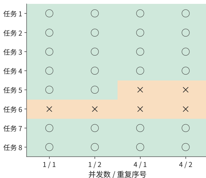
图 8-27: 同一任务与运行顺序，原 FP8 实现共 26/32 正确。这一比较包含实现选择对 Q 精度的影响。圆圈表示回答正确，叉号表示回答错误；每行对应同一道题，列表示并发数与重复运行序号。
