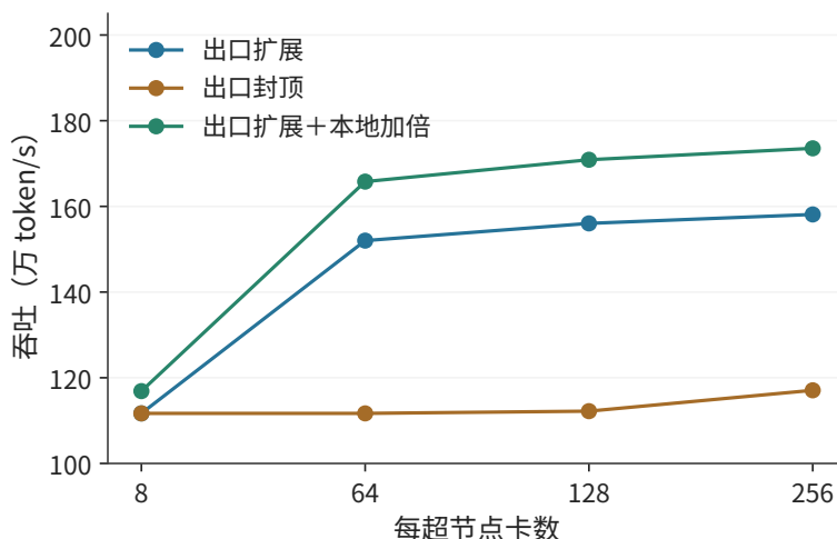
图 7-62：全局 token 数与总卡数固定。蓝线增加每节点外部出口，橙线将出口封顶在 400 GB/s，绿线在出口扩展的基础上将本地带宽从 450 翻倍到 900 GB/s。每点在声明的连续环与分层归约之间选择较快者；纵轴为固定调度估算的正常运行吞吐。
