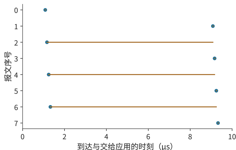
图 7-46：第二条路径传播时延增加到 9 \mu\text{s} 。快路径后续报文先到，仍需等待前方缺口；约 9.33 \mu\text{s} 全部可交付。圆点表示报文到达，横线表示到达后等待缺口补齐的时间，纵轴是报文序号。
