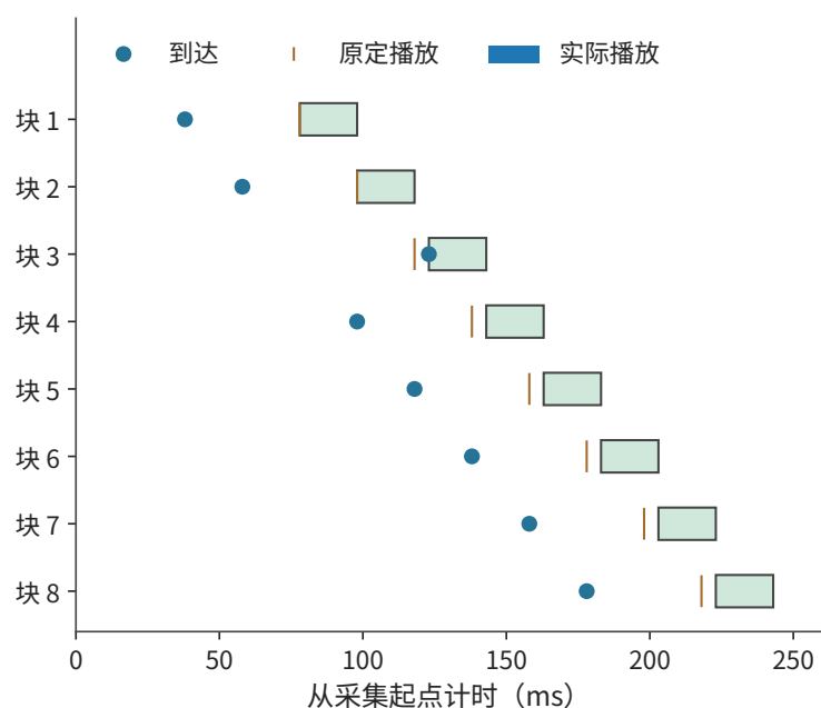
图 3-19 八块音频的教学播放时间线。每块长 20 ms，圆点标到达，短竖线标原定播放时刻，色条标实际播放；第三块晚到 5 ms，后续播放随之顺延。
