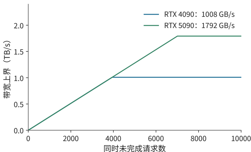
图 4-15 每事务 128 bytes、返回延迟 500 ns 时，增加在途请求数会提高带宽上界，直到碰到 RTX 4090 或 RTX 5090 显存接口本身的速率上限。
