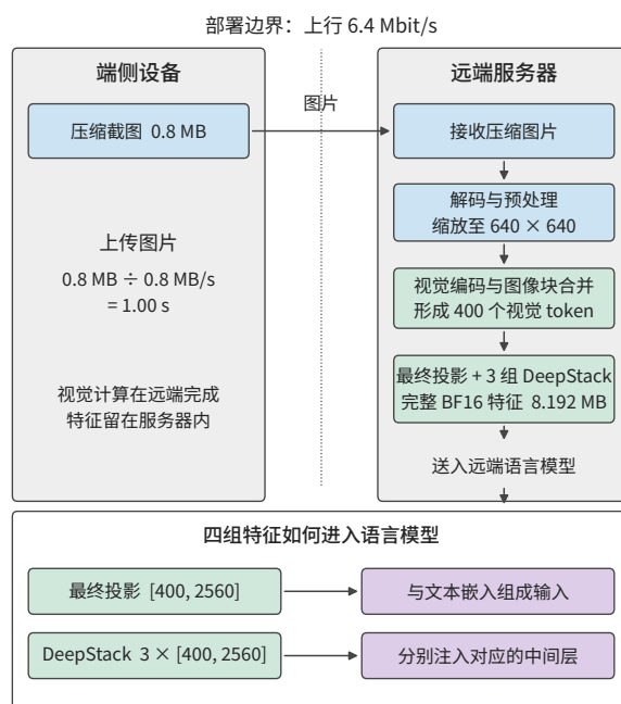
图 12-10：远端编码的执行路径。端侧上传 0.8 MB 压缩截图，远端依次完成解码与预处理、视觉编码和特征接入；最终投影与三组 DeepStack 特征均留在服务器内。6.4 Mbit/s 上行的图片发送时间为 1 秒，编码和排队时间另计。
