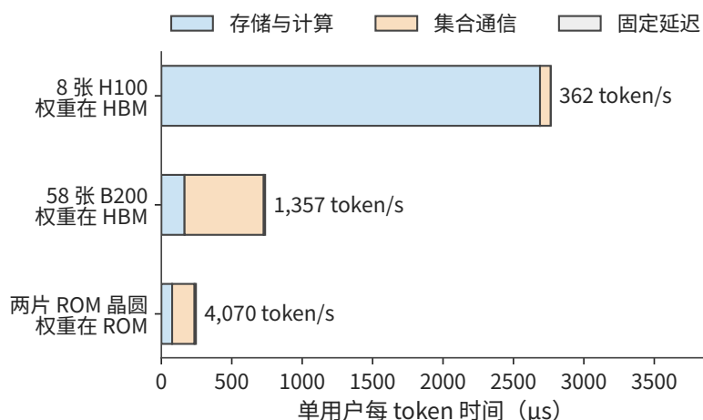
图 6-55: 三种机器上 V4.1 Flash 单用户每 token 时间的构成, 200K 上下文, batch 为 1。权重在 HBM 时存储读取占绝大部分, 权重进 ROM 之后集合通信成为最长的一项。
