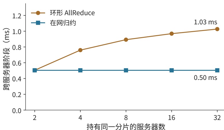
图 7-8: 持有同一分片的服务器从 2 台增至 32 台时，跨服务器阶段的时间。环的每网卡发送量趋近两个分片、轮数按 2(S-1) 增长；在网归约保持一个分片、一轮。两台服务器时两者只差一次启动。
