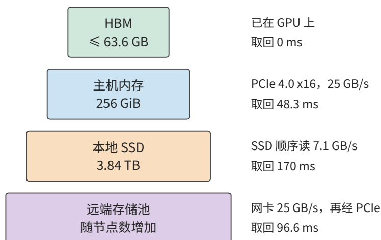
一张 A100 可用的 KV 存储层次
