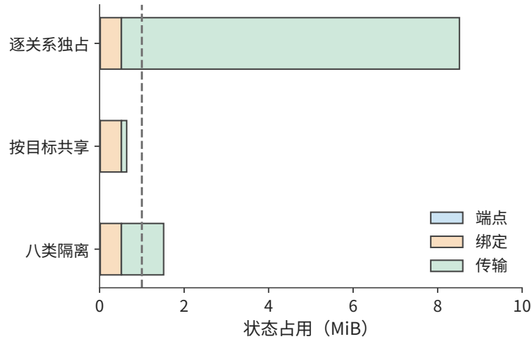
图 7-32: 64 个端点访问 128 个目标。蓝色为端点记录，橙色为关系绑定，绿色为传输状态。虚线为 1 MiB 容量；划分八个隔离组时，为各目标保存八份独立的传输状态。
