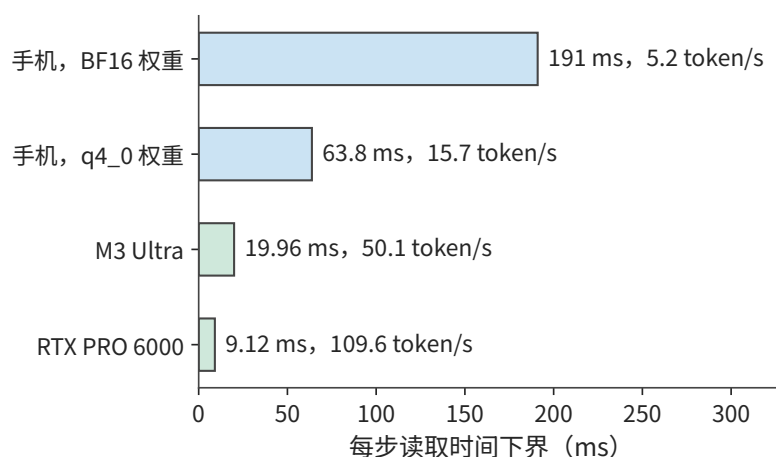
图 12-9: 三档本地设备读一遍 Qwen3-8B 单请求 8K decode 主要载荷 (16.345 GB) 的时间下界。手机按四条 x16 LPDDR5X 通道计, 合计 84.8 GB/s, BF16 与 q4_0 权重分别成行; M3 Ultra 与 RTX PRO 6000 取自第 4.8.2 节的设备表。柱端标注对应的 token/s 上限。
