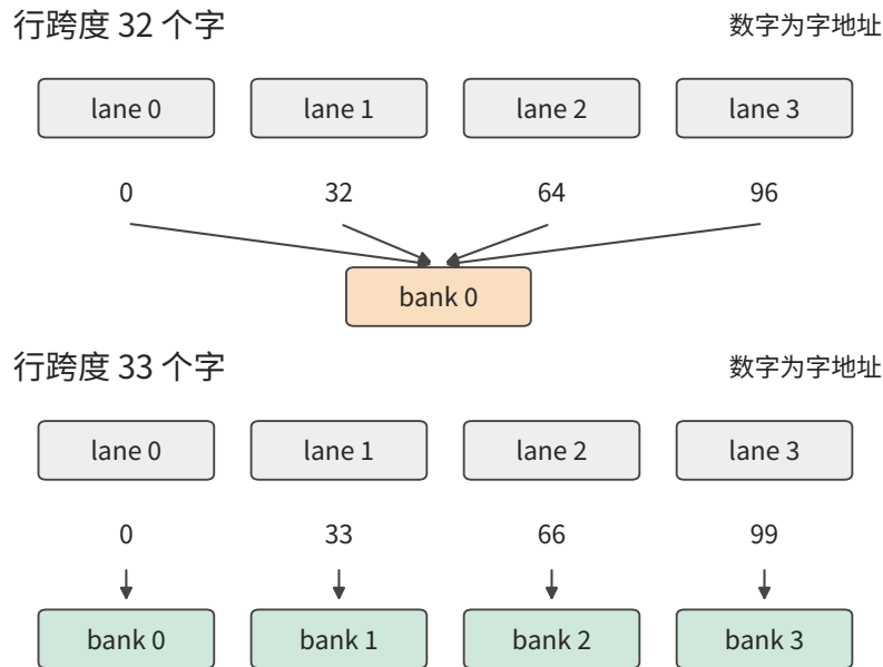
图 5-10：同一列的 32 个不同字由 32 个 lane 同时请求。上半图行跨度为 32 个字，请求集中到同一 bank；下半图补齐为 33 个字，请求分散到 32 个 bank。图中画出前四个请求；假设每个 bank 每轮提供一个 32-bit 字，不计广播。
