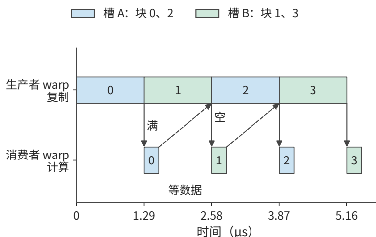
图 5-5：上行是生产者 warp 发出的异步复制，下行是消费者 warp 的计算；蓝、绿分别为槽 A、B。实线箭头为“满”栅栏，复制完成后计算才能开始；虚线箭头为“空”栅栏：块 0 在 1.57 \mu s 用完槽 A，块 2 的复制到 2.58 \mu s 才开始，生产者不必等槽。H100 一个 SM 上每块复制 1.29 \mu s、计算 0.28 \mu s；复制首尾相接，消费者每算完一块就等下一次“满”栅栏。
