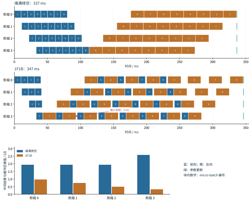
图 10-17：填满排空先完成八个 micro-batch 的前向，再执行反向，最后更新参数。蓝色为前向，橙色为反向，绿色为参数更新。四个阶段共用同一时间刻度，按正文的计算与传输条件共需 337 ms。
