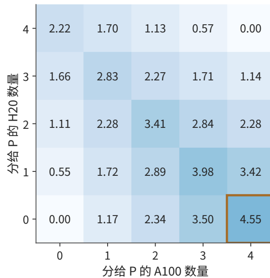
图 9-10：阶段配比如何限制请求率。四张 A100 与四张 H20，阶段能力见例 9.2；横轴为分给 P 的 A100 数，纵轴为分给 P 的 H20 数，其余分给 D。每格取两池能力与 25 GB/s 网卡交接能力的最小值，不含排队；颜色深浅表示可持续的请求率，单位为请求/s，框出的格子为最优配比。
