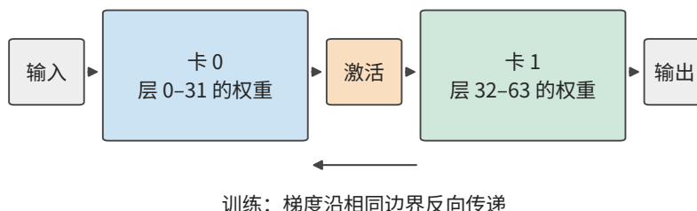
图 6-13：两个阶段各保存自己那些层的权重。相邻阶段之间只交接激活；训练时梯度沿同一边界反向传递。
