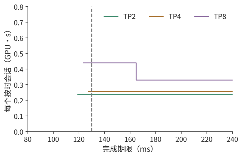
图 6-51：无故障时，按时完成会话的平均成本随期限变化。八卡计费至所有会话结束；曲线从至少三个会话按时完成处开始。TP 数值为每实例使用的卡数；成本以 H100 的 GPU·s 计。TP1 放不下 128K 会话，没有曲线。
