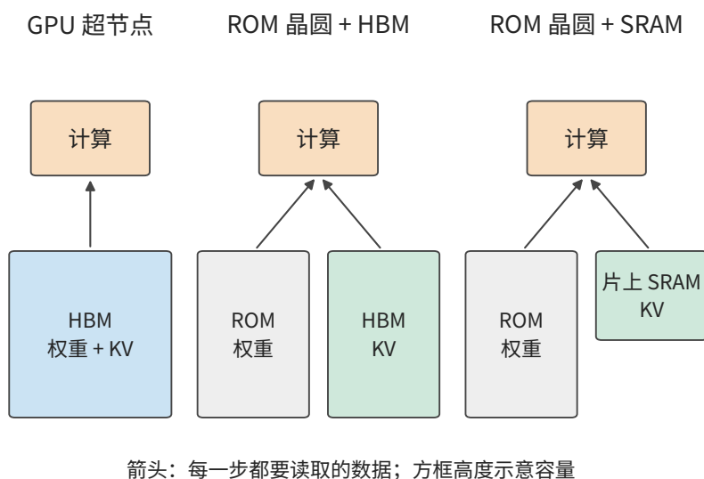
图 6-54: 权重与 KV 的三种放置方式。左：GPU 的权重与 KV 共用 HBM；中：权重在制造时写入 ROM，KV 放 HBM；右：权重在 ROM，KV 放片上 SRAM，容量小得多。箭头是每步都要读取的数据，方框高度示意容量。
