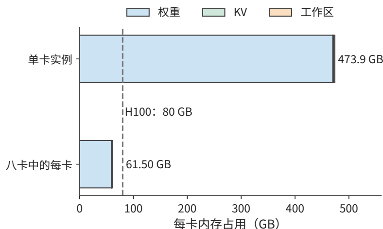
图 6-2: 单卡实例与分到八张卡后的每卡内存需求。单卡需要约 473.9 GB，远超 H100 的 80 GB（虚线）；分到八张卡后每卡约 61.50 GB。2 GiB 工作区在每张卡分别预留。
