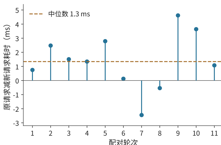
图 5-40：同轮替换前的请求时间减去替换后的请求时间，正值表示替换后更快。RTX PRO 6000 上的 Qwen3-8B，7239 个 token 的输入、强制 32 个 token 的输出，并发 1，BF16、eager，关闭前缀缓存；11 对交错计时，轮内顺序随机，期间有其他驻留服务。虚线为配对时间差的中位数约 1.3 ms。阶段表来自单独采集的性能分析记录。
