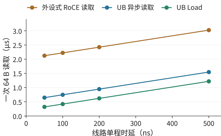
图 7-20：一次 64 B 读取的总时间随线路单程时延的变化。三条直线的斜率都是 2，截距是各自的固定开销；路径之间的差距来自固定开销，不随线路时延变化。
