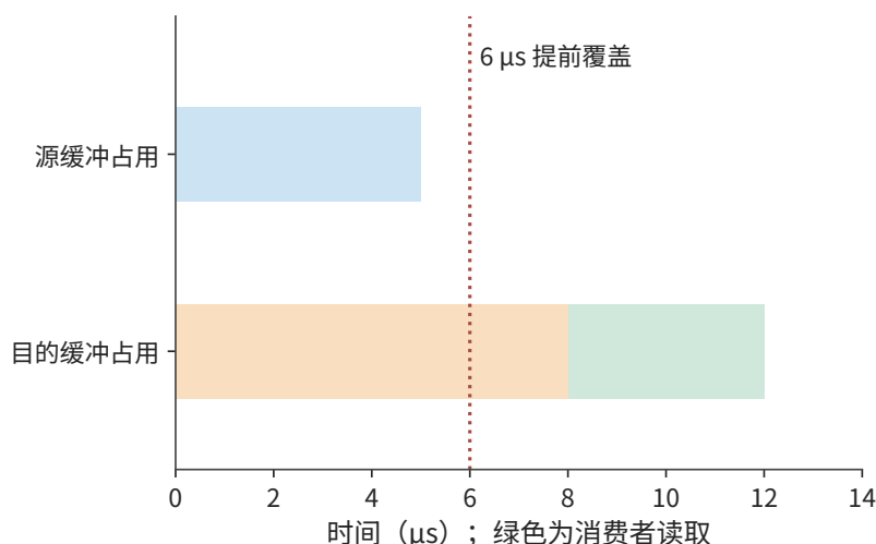
图 7-30：源缓冲占用到 5 μs 发送完成；目的缓冲持续占用到 12 μs 消费者用完。绿色为 8–12 μs 的读取区间。虚线标出 6 μs 提前覆盖目的地址的错误操作。
