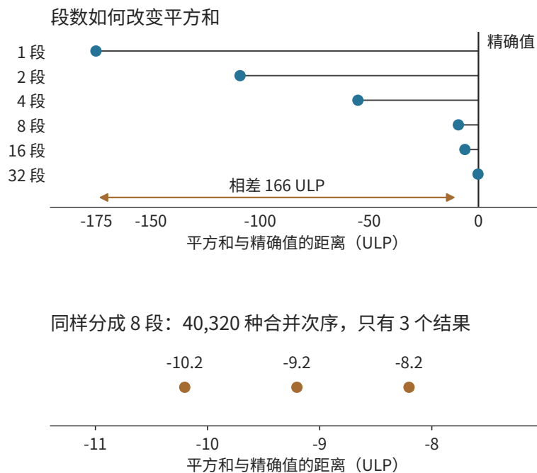
图 5-13：同一行 4096 个 BF16 元素的平方和与精确值的距离，横轴单位为 FP32 的 ULP。上半图比较 1 到 32 段的六种切分；下半图固定八个局部和，列出全部合并次序得到的结果。精确值用有理数算得，只作比较基准。
