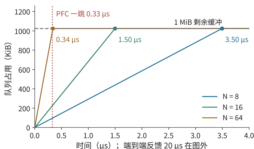
图 7-44： N = 8 、 16 、 64 时队列以 300 、 700 、 3100 \text{ GB/s} 的超额速率增长，圆点标出 1 \text{ MiB} 剩余缓冲被填满的时刻 3.50 、 1.50 、 0.34 \mu\text{s} 。竖直虚线是 PFC 的一跳反馈距离 0.33 \mu\text{s} ，三条线在这之前都没有填满；端到端反馈的 20 \mu\text{s} 在图的横轴之外。
