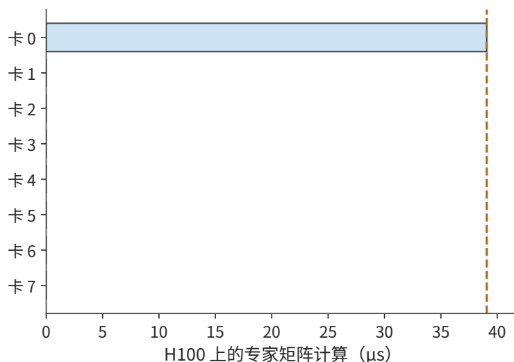
图 9-20：512 次全部落在卡 0，其他卡空闲。相同总计算量，需要等待卡 0 完成；两图使用相同时间尺度。
