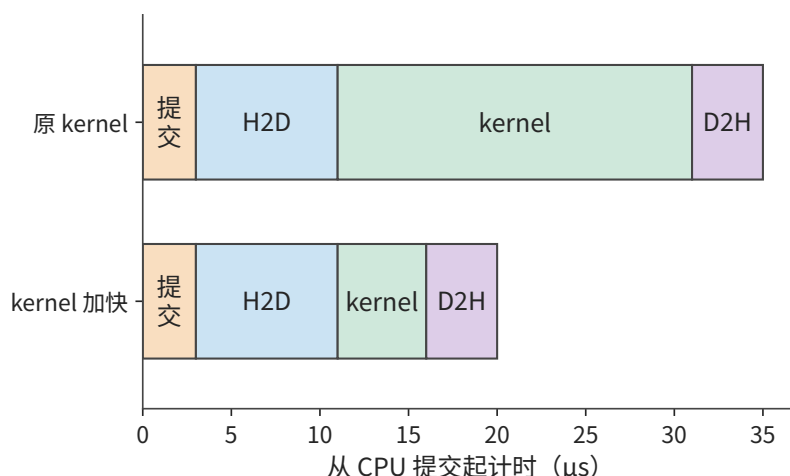
图 5-3: CPU 提交、H2D 输入复制、kernel 执行与 D2H 结果返回依次发生。上方 kernel 执行 20 \mu\text{s} , 结果在第 35 \mu\text{s} 可用; 下方 kernel 执行 5 \mu\text{s} , 结果在第 20 \mu\text{s} 可用。
