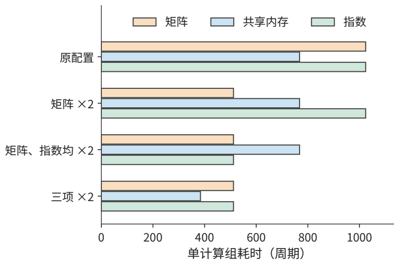
图 4-11 同一注意力块在四种资源配置下的服务周期。矩阵、共享内存和指数三项分别比较，单独增加一种能力后，其他资源可能成为较长的一项。“×2”表示相应资源的吞吐能力提高一倍，横轴为完成同一计算块所需的时钟周期数。
