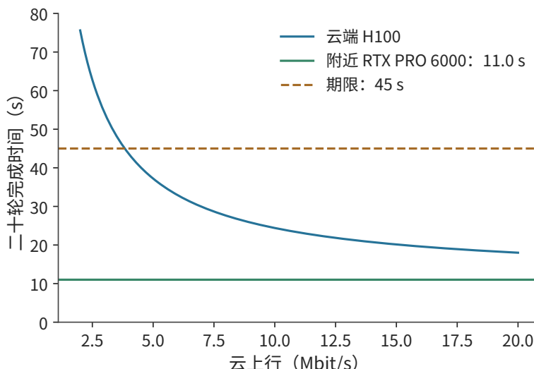
图 12-31: 云路径上行改变完整任务的部署选择。剩余 20 轮每轮上传 0.8 MB，云端准备 0.14 秒，每轮其余工作合计约 0.57 秒，因此总时间为 11.6 + 128/b 秒；附近工作站为 11.0 秒，期限为 45 秒。本例保持模型、处理时间和其他网络参数不变，忽略排队与故障。约 3.8 Mbit/s 起云方案可满足期限；上行再高，云端也不低于 11.6 秒，始终慢于附近工作站。
