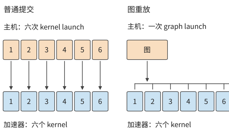
图 5-27：普通提交时，主机为每个 kernel 发起一次 launch；图重放时，主机只发起一次 graph launch，加速器仍然执行图中记录的六个 kernel。要减少 kernel 的数量，靠的是融合，不是图重放。
