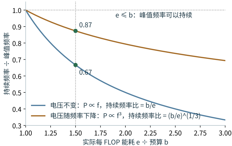
图 4-7 持续频率与峰值频率之比随每 FLOP 能耗 e 与预算 b 之比的变化：电压不变时为 b/e ，电压随频率下降时为 (b/e)^{1/3} 。 e/b 不超过 1 时峰值频率可以持续； e/b 为 1.5 时两条曲线分别给出 0.67 与 0.87 。
