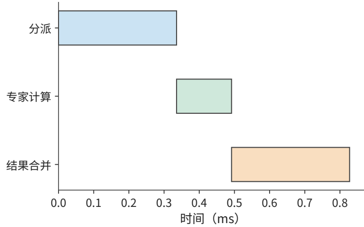
图 9-25: 整批依次分派 0.336 ms、计算 0.156 ms、合并 0.336 ms，总时间 0.827 ms；数值取自第 9.4.1 节表中跨服务器的均衡分布。
