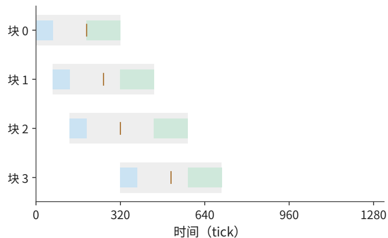
图 4-20 三个输入槽提前发起前三块，第一槽释放后接收第四块。矩阵单元从 192 连续计算到 704 tick，第四槽不再缩短完成时间。横轴一个 tick 为 B200 SM 的一个时钟周期；各行对应一个数据块，灰色表示输入槽占用，蓝色表示传输，绿色表示计算，竖标记表示数据就绪。
