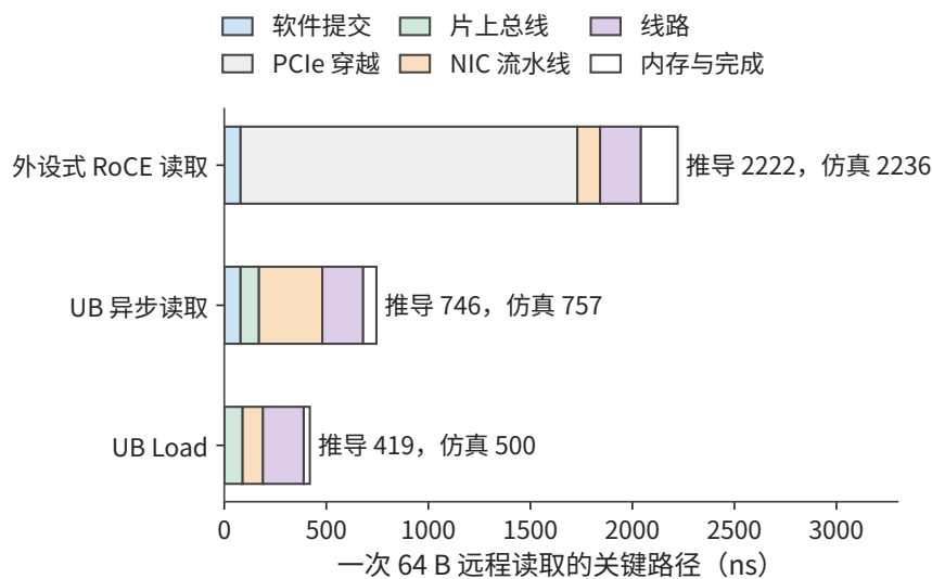
图 7-19：三条路径的关键路径按阶段类别堆叠。经 PCIe 外设网卡的路径中，浅灰色一段是五次 PCIe 穿越；两条片上总线路径没有这一段，Load 路径还省去了软件提交和完成轮询。条形右侧标出推导值和仿真值。
