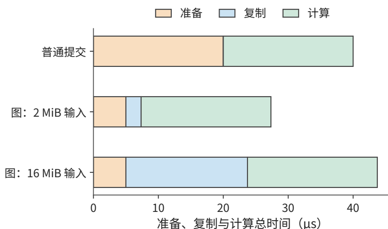
图 5-33：橙色为准备，蓝色为额外输入复制，绿色为加速器计算。普通方式 40 \mu\text{s} ；图的 2 MiB 输入约 27 \mu\text{s} ，16 MiB 输入约 44 \mu\text{s} 。复制按 RTX PRO 6000 的显存带宽 1792 GB/s 计。
