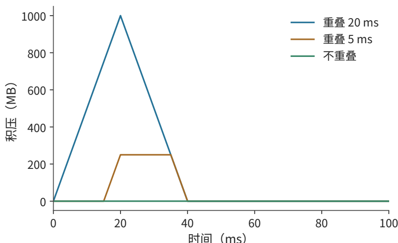
图 7-41：把到达速率与出口速率的差额随时间累积，得到 1000、250、0 MB 三种峰值。此算例按无限缓冲计算积压。
