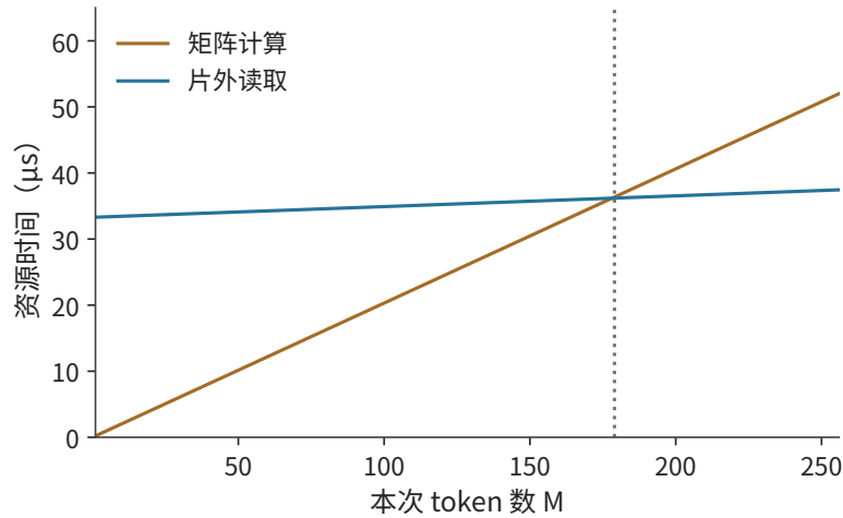
图 4-35 同一 Q 投影的计算与访存耗时随输入行数的变化。计算量按行数增长，片外访问同时包含固定权重和增长的输入输出；从 179 行起计算项较长。
