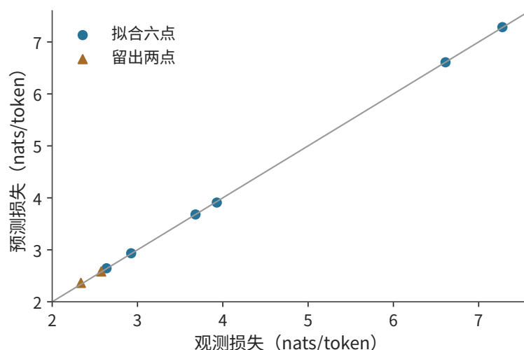
图 3-27 八个公开 C4 观测的预测与实际损失。6 点用于拟合，2 点预先留出作检验；对角线表示预测等于观测，点到线的偏差反映误差。
