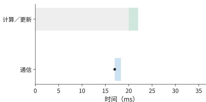
图 7-58：本图把分层归约的通信提前到 17 ms 开始。通信在 18.3 ms 结束，早于计算，更新从 20 ms 开始，整步 22 ms。灰色为计算，蓝色为通信，绿色为更新；圆点为通信数据就绪。
