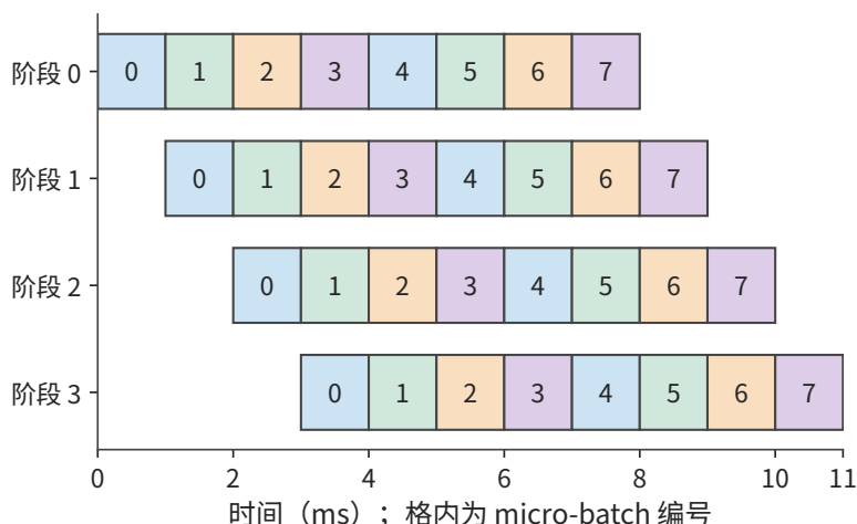
图 7-9: 四个前向阶段如何处理八个 micro-batch。每格为 1 ms，数字表示 micro-batch 编号；同一编号沿右下方移动，表示该 micro-batch 依次通过各阶段。每个阶段计算 8 ms，在 11 ms 的总时间中各空闲 3 ms。阶段耗时相同，图中忽略额外交接开销。
