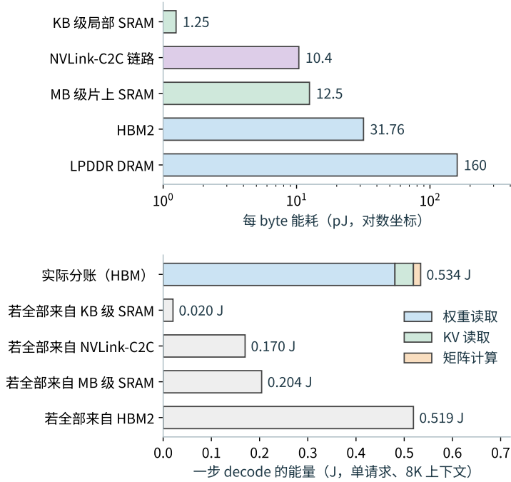
图 4-5 上：各级存储与链路每 byte 能耗，对数坐标。下：Qwen3-8B 单请求 8K decode 一步的能量分账（权重 0.481 J、KV 0.038 J、计算 0.015 J），以及同样 16.345 GB 全部来自某一层时的能量。
