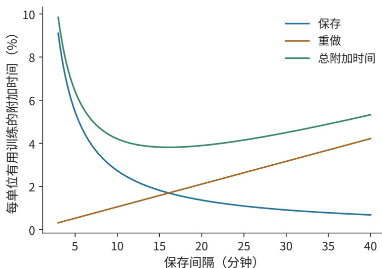
图 10-35: 蓝线为保存耗时占比，橙线为故障重做耗时占比，绿线为两者加上恢复耗时后的合计。使用 1024 卡作业平均 7.9 小时中断一次、保存约 16.4 s 和恢复 120 s 的一阶模型。最低点出现在两项随间隔变化的代价相互平衡处。
