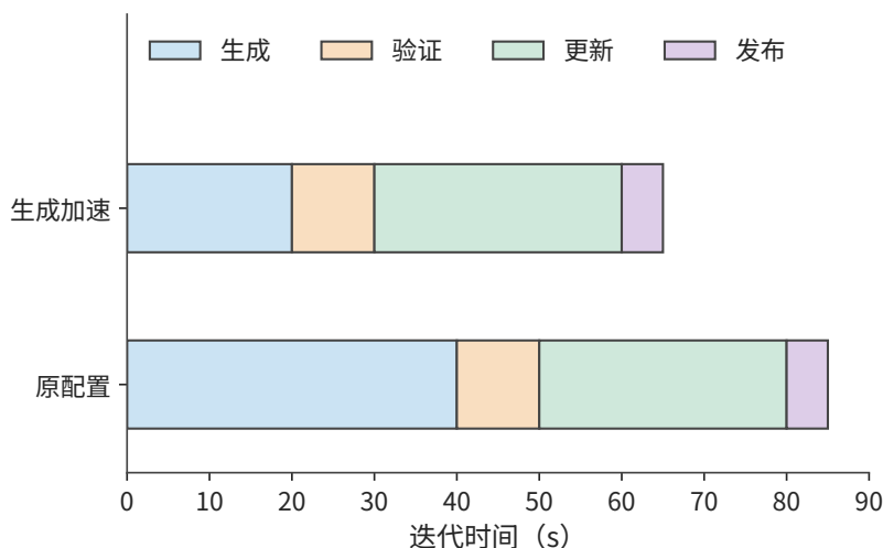
图 11-24：四个阶段依次执行。生成时间由 40 秒降至 20 秒，其余三段仍共需 45 秒，因此每轮总时间由 85 秒降至 65 秒。条形长度按时间比例绘制。
