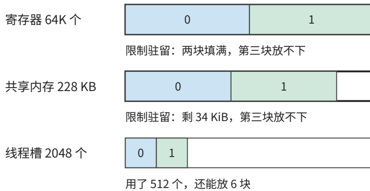
图 5-4：三条分别表示 SM 的寄存器、共享内存与线程槽总量，蓝、绿为两个驻留线程块的占用。寄存器恰好填满，共享内存剩余 34 KiB 放不下第三块的 97 KiB，两者同时限制驻留；线程槽只用了 512 个。每块 256 线程、每线程 128 个寄存器、96 KiB 共享内存，另加每块 1 KiB 预留。
