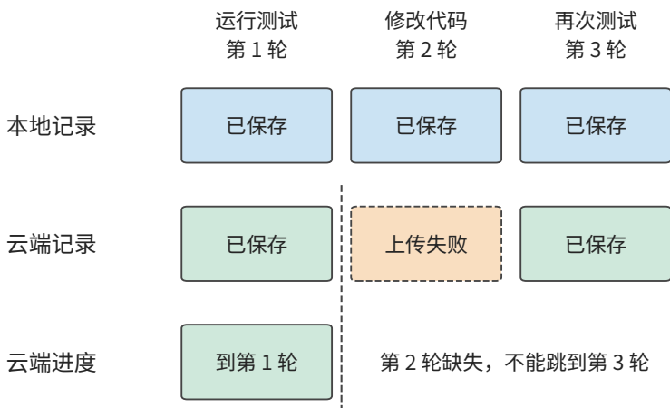
图 11-35：初始状态已在本地和云端保存，每列代表一个 ReAct 轮次。每轮先保存到本地，再异步上传该轮新增记录；本例允许上传失败后继续执行和上传后续轮次。第二轮上传失败后，即使第三轮上传成功，云端历史仍只完整到第一轮。横向排列表示轮次顺序，不表示耗时。
