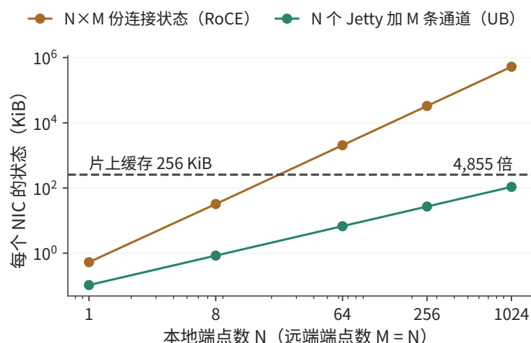
图 7-33: N 个本地端点访问 M = N 个远端端点时，两种组织方式下网卡保存的状态。逐对连接在 N 略大于 20 时就超过 256 KiB 的片上缓存，端点加通道到 N = 1024 时仍不到缓存的一半。
