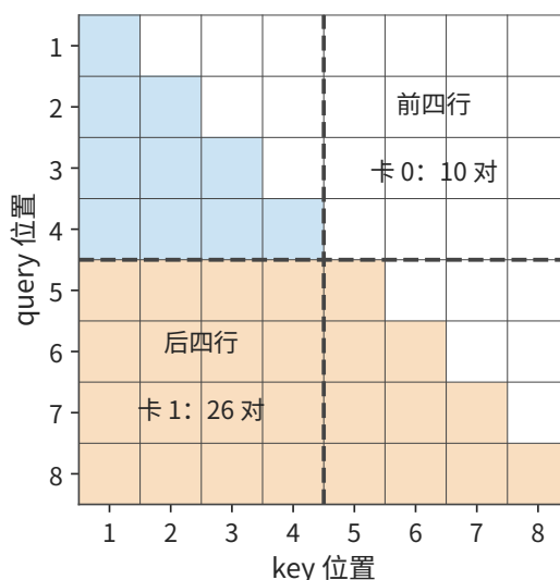
图 6-12：八个 token 的因果注意力，横轴为键的位置、纵轴为查询的位置。实色格是必须计算的查询—键配对；前四行归卡 0，后四行归卡 1。虚线只是设备边界，左下区域的远端依赖并不因此消失。
