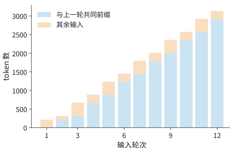
图 8-18：蓝色为与上一轮逐 token 相同的前缀，橙色为其余输入。此图描述输入内容的可复用程度，实际缓存命中还取决于状态是否保留。
