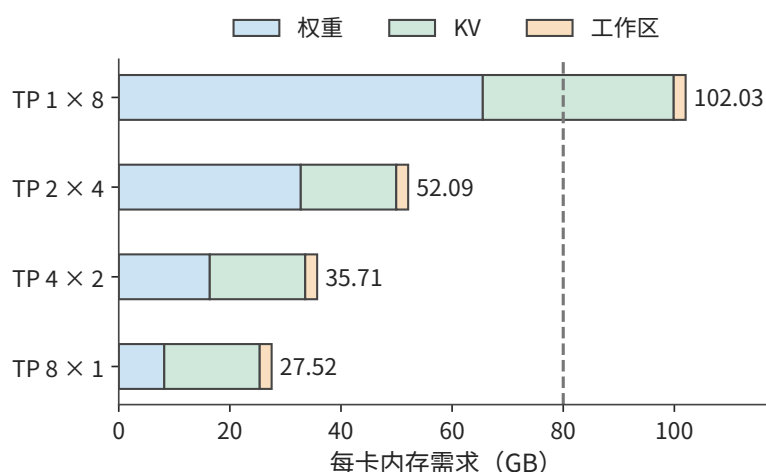
图 6-47：四种部署在 128K 会话下的每卡内存需求，包括权重、实例内全部排队会话的 KV 和 2 GiB 工作区。单卡实例每卡要 102.03 GB，超过 H100 的 80 GB（虚线）；两卡、四卡、八卡实例分别约为 52.09、35.71、27.52 GB。
