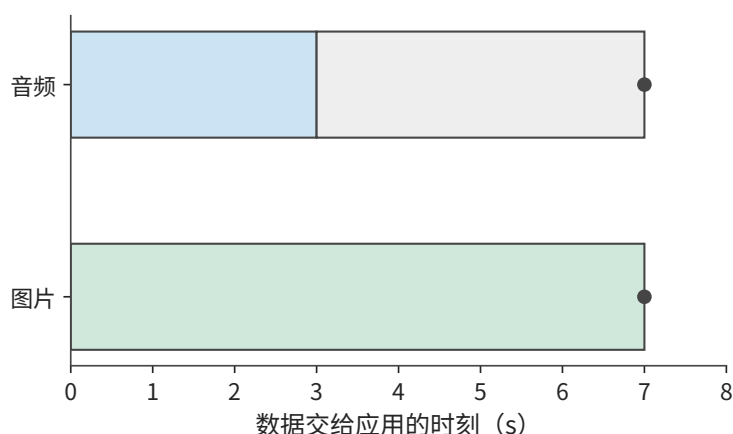
图 12-19：整体有序交付：音频第 3 s 已收齐，却因图片缺口继续等到第 7 s。灰色段表示数据已齐后的等待，圆点表示数据交给应用的时刻。
