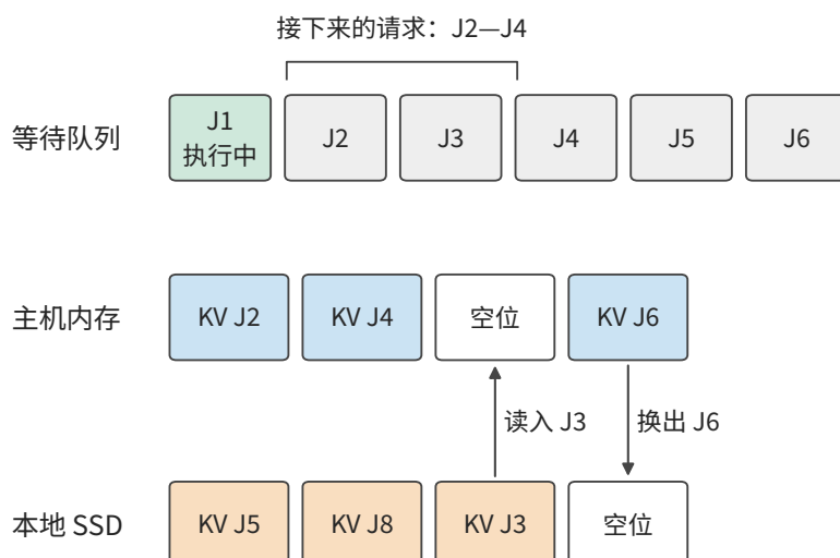
图 9-35: 主机内存有四个存放位置, 其中一个留作空位, 用于接收读入的数据, 其余三个留给队列中接下来的 J2—J4。J3 的状态仍在 SSD 上, 在它排队期间读入空位; J6 排在这三个请求之后, 下次使用最晚, 先换出到 SSD。
