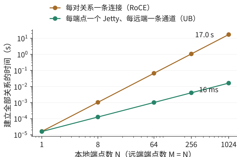
图 6-41：在 N 个本地端点与 N 个远端端点之间建立全部连接所需的时间，32 个核并行执行。逐对连接的时间随 N^2 增长，端点加通道随 N 增长； N = 1024 时二者相差约一千倍。
