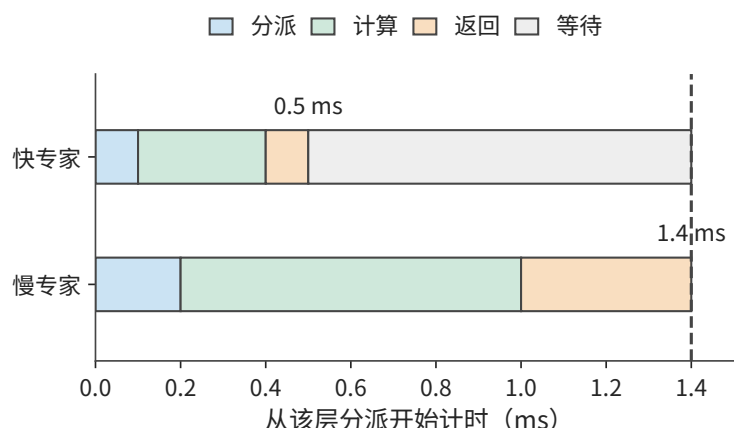
图 9-27：一个 token 选中的两条专家分支，教学时长分别为 0.5 ms 与 1.4 ms。每条都依次经过 dispatch、计算与 combine；同一个 token 要等两份结果，图中忽略本地加权合并的时间。灰色表示快分支的结果到达之后等待的时间。
