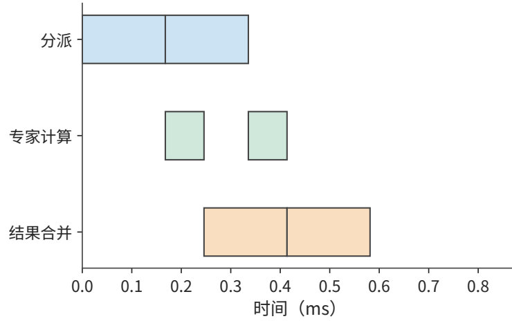
图 9-26: 每个 micro-batch 的各阶段时间减半，三条轨道使用独立资源。第一个 micro-batch 计算时可以 dispatch 第二个 micro-batch，总时间降到 0.581 ms。
