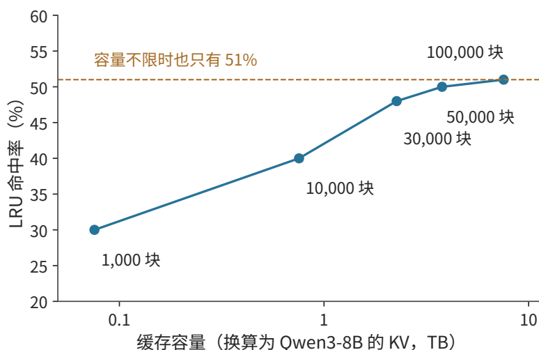
图 9-31：命中率随容量增加而趋于饱和。数据为 Mooncake 一小时采样 trace 在 LRU 淘汰下的命中率，每块 512 个 token；横轴按 Qwen3-8B 每 token 144 KiB 换算为字节。这只是采样得到的一段流量，真实服务所需的容量按流量同比例放大。
