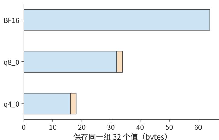
图 8-23：BF16、q8_0、q4_0 保存同一组 32 个数值所需的总空间。横条按字节数成比例绘制；橙色为每组 2 bytes 的 scale。把每组总长度乘以组数，就得到整条上下文的 KV 容量。
