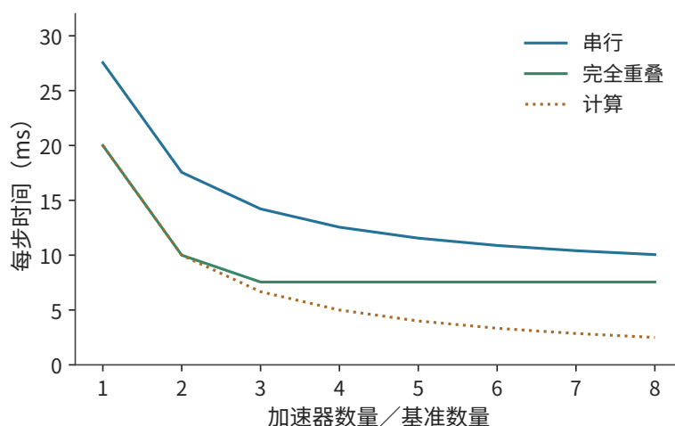
图 7-2: 跨服务器传输量固定时增加卡数的效果。每方向发送 360 MiB，经一张 50 GB/s 网卡；计算时间从 20 ms 开始，随卡数增加按反比缩短。曲线分别按计算与通信串行、完全重叠计算，通信项取割集传输时间。
