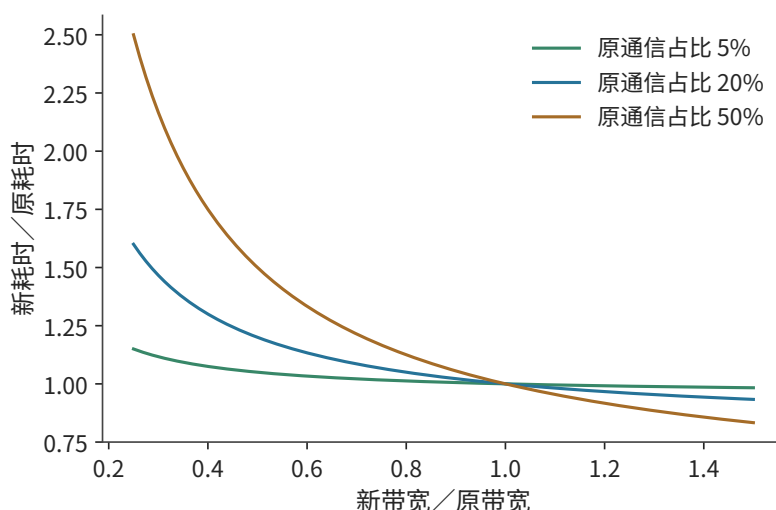
图 10-46：资源能力变化的收益由原有等待时间占比决定。曲线按 T'/T = 1 - f + f/r 计算，固定单卡计算与依赖，通信时间与有效能力成反比。
