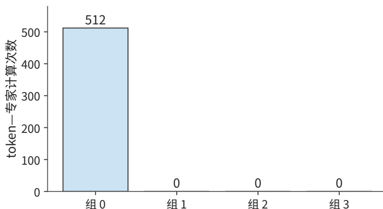
图 6-21：所选八个专家都在组 0：权重读取降到 288 MiB，512 次计算却全部压在同一组。
