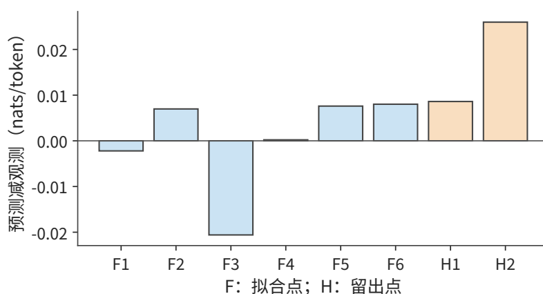
图 3-28 同一组预测误差的放大视图。F1—F6 为拟合点，H1—H2 为留出点；纵轴是预测减观测，保留正负号。
