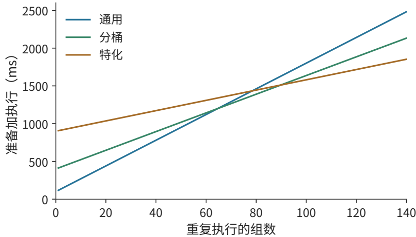
图 5-35：同一组调用反复执行时，最省时的策略随复用次数变化。曲线采用例 5-12 的形状、处理率和准备时间，不同策略适用的整数调用次数范围使用未经四舍五入的数值计算。“通用”使用同一执行方案处理所有形状；“分桶”将相近形状归组；“特化”为具体形状选择专用方案。
