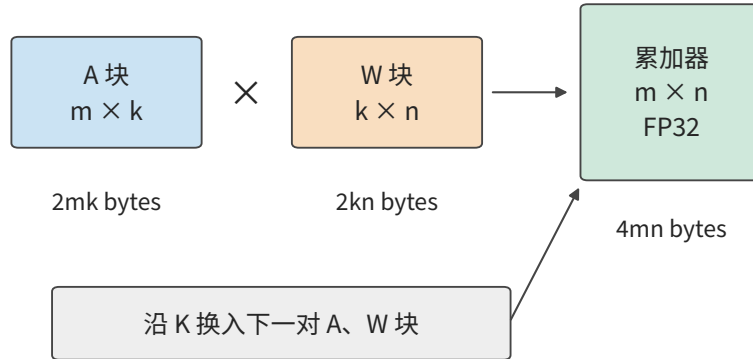
一对输入块，更新整个输出块
