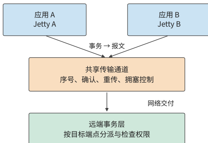
图 6-38: 两个本地应用保留各自的 Jetty, 经共享传输通道访问远端端点。事务层区分操作及其完成归属, 传输层处理报文的可靠交付; 共享通道不取消权限检查, 也不自动建立跨应用的全局顺序。
