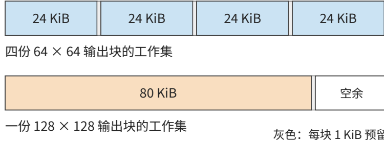
图 5-9：条形总长均表示 RTX PRO 6000 一个 SM 的 100 KB 共享内存。24 KiB 的工作集连同每块 1 KiB 预留，恰好放下四份；80 KiB 的只能放一份。
