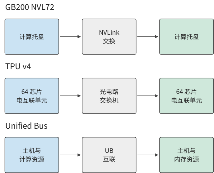
图 6-42：三个公开系统的连接层次。NVIDIA 用 NVLink 连接设备，TPU v4 用 OCS 连接电互联单元，Unified Bus 将主机侧计算和内存资源接入统一互联。
