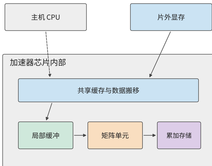
图 4-2 主机、显存与芯片内部的关系。实线表示数据经过缓存、局部缓冲、矩阵单元和累加存储，虚线表示主机提交工作。图按硬件功能分组。
