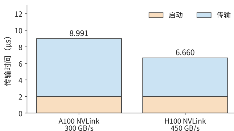
图 4-25 一次 2 MiB 传输在相同启动条件下的时间。蓝色传输项占主要部分，换成 H100 的 NVLink 带来更显著的收益；本图纵轴范围与上一图分别标注。
