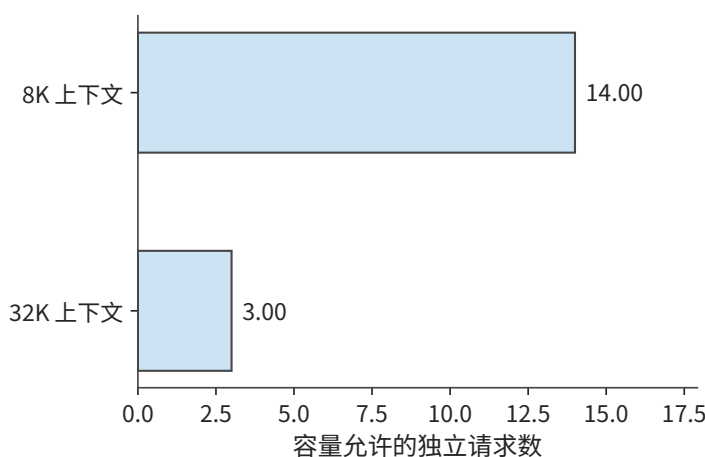
图 2-33 70B 的 4-bit 方案在同一张 80 GB 的 H100 SXM 上，上下文长度从 8K 增至 32K 时可同时容纳的独立请求数。每请求状态增加，使剩余空间容纳的请求数减少。
