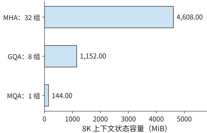
图 2-10 固定 Qwen 层数、头宽、8192 个上下文 token 与 BF16，只改变 KV 组数。实际模型采用 GQA；其余两柱是用于分析共享比例的结构变体。
