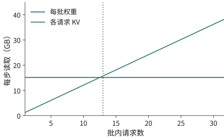
图 4-33 固定权重的同时，各请求仍独立读取 KV。题设每请求保留 8K 上下文，batch 从 13 起 KV 读取超过共享权重读取。
