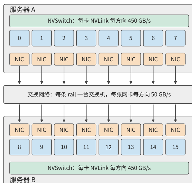
图 7-1：固定两台服务器，每台八张卡。服务器内的卡经 NVLink 与 NVSwitch 互联，每张卡各有一张网卡；跨服务器的数据从发送方的网卡经交换网络到达接收方的网卡，每张网卡每个方向提供 50 GB/s。
