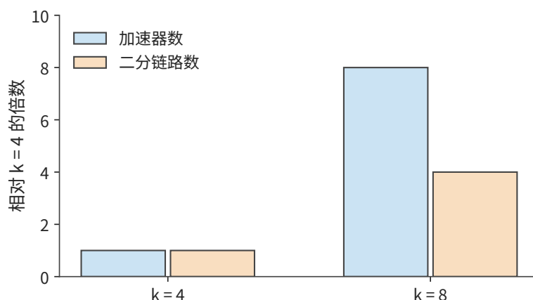
图 6-37: k 从 4 增到 8 时，芯片数从 64 增到 512，二分链路从 32 增到 128。两种增长均以 k = 4 时为基准。 k 表示三维环面每个维度的节点数，总节点数为 k^3 。
