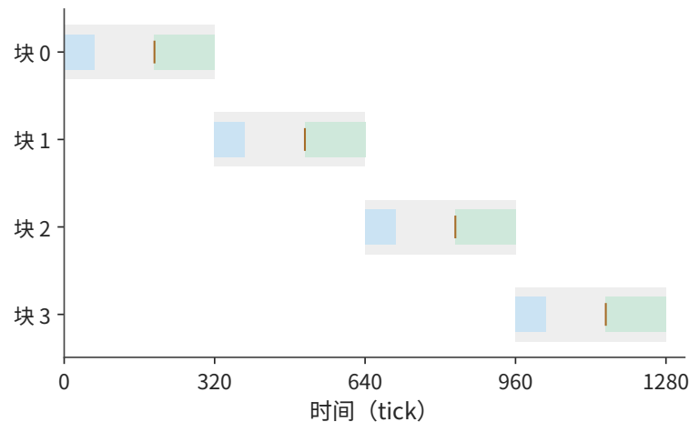
图 4-18 一个输入槽的四块时序。蓝条为传输，橙线为就绪，绿条为计算，浅灰为槽占用；上一块用完后才能再次发起，完成时刻为 1280 tick。一个 tick 为 B200 SM 的一个时钟周期。
