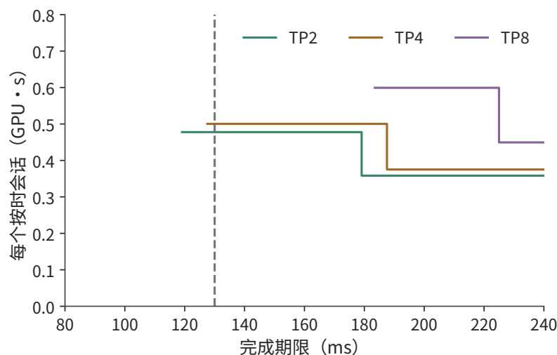
图 6-52：20 ms 时卡 0 故障，受影响实例在 60 ms 从当前会话起点重新执行。采用与无故障图相同的计费方法和纵轴范围。TP 数值为每实例使用的卡数；成本以 H100 的 GPU·s 计。
