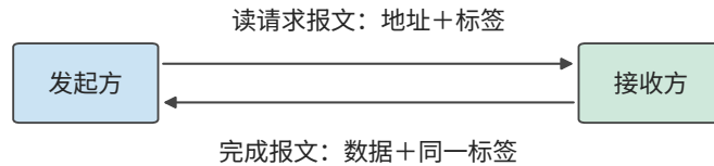
图 7-27: 写是 posted 事务, 一个报文发出即完成; 读要先发带标签的请求报文, 再等带同一标签的完成报文把数据送回, 在途的读不能超过标签数和信用数。
