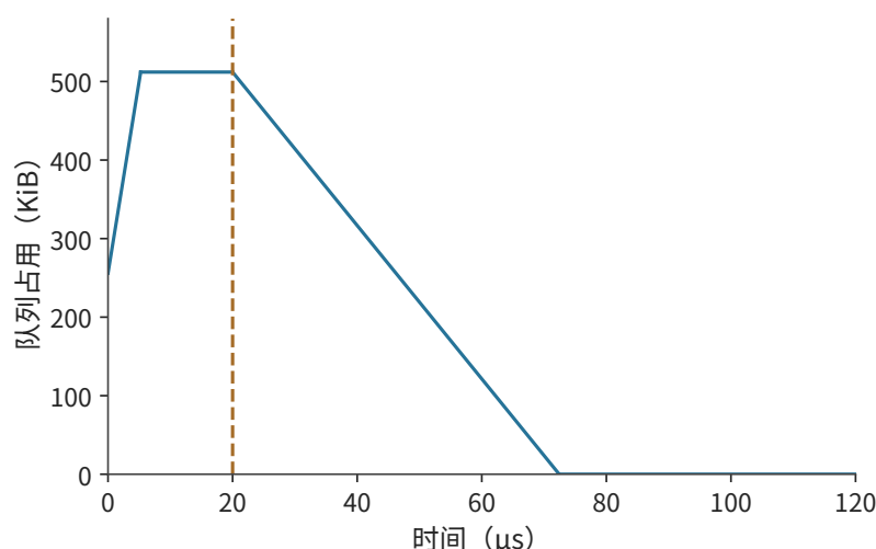
图 7-43: 反馈生效之前，缓冲区还会继续填满。到达速率为 100 GB/s，出口为 50 GB/s，512 KiB 缓冲初始占用一半。5.2 \mu\text{s} 时填满，到 20 \mu\text{s} 降速前持续丢弃超额到达的数据；降至 40 GB/s 后，出口以 10 GB/s 的净速率排空积压。反馈时刻与降速幅度为给定条件。
