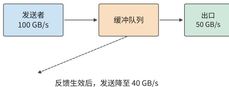
图 7-42: 数据沿实线进入队列并由出口发送；虚线表示拥塞反馈返回发送方。反馈到达并生效前，原发送速率继续填充队列。
