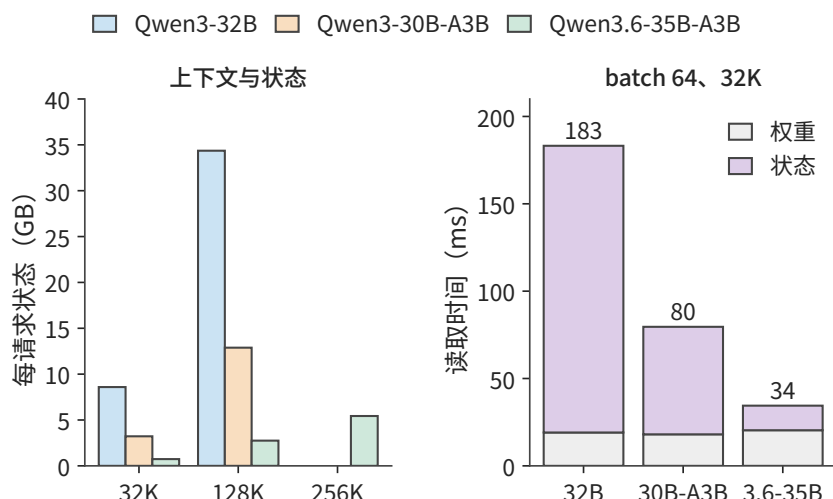
图 6-6: 左图为单个请求在 32K、128K 与 256K 上下文下的状态, Qwen3-32B 与 Qwen3-30B-A3B 的上下文上限为 128K。右图为 batch 64、32K 上下文时一次 decode 读取权重和状态的时间, 按 H100 的 3350 GB/s 计。三种模型的权重读取相近, 状态读取相差十倍以上。
