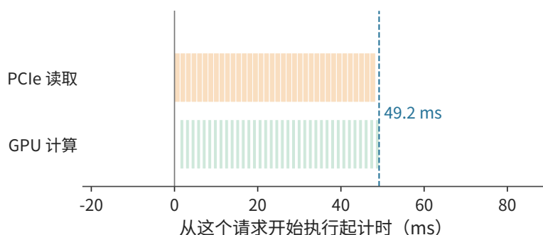
图 9-33：逐层预加载。GPU 计算某一层时，PCIe 读取后面的层；每层读取 1.34 ms、计算 0.857 ms，每层的计算都要等待读取，总时间 49.2 ms 由读取决定。
