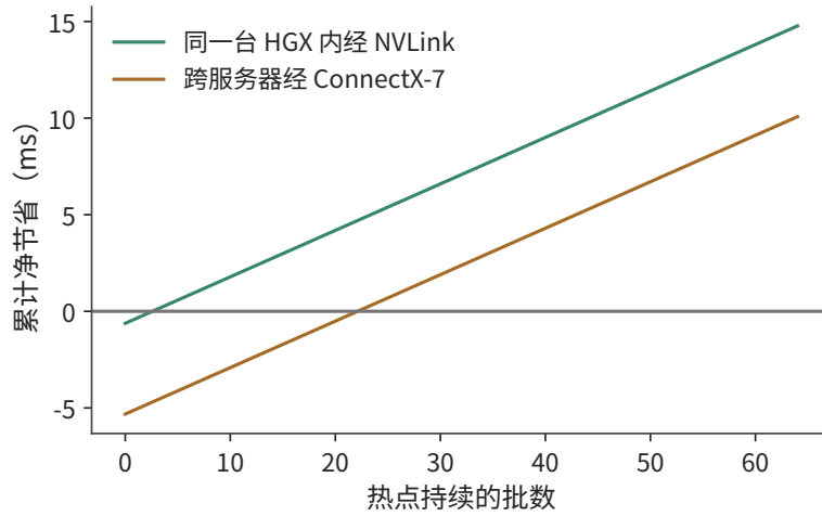
图 9-24：热点持续多久，专家复制才值得。每批节省约 0.240 ms；同一台 HGX H100 内经 NVLink 复制一次约 0.622 ms，第 3 批开始净获益；跨服务器经 ConnectX-7 网卡复制约 5.32 ms，第 23 批开始净获益。曲线使用例 9.6 中未经四舍五入的时间计算；七张接收卡各需额外 36 MiB，假设热点不变。
