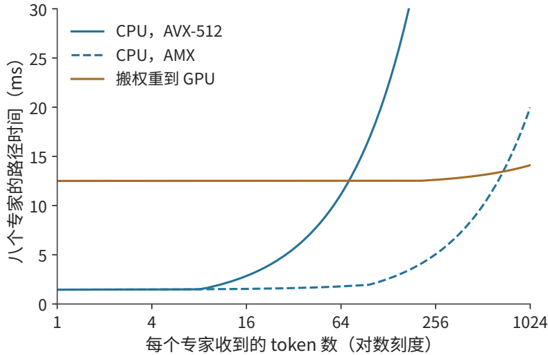
图 9-14：专家复用改变执行位置的选择。八个专家各有 36 MiB BF16 权重。CPU 为单颗 Xeon Platinum 8452Y，AVX-512 与 AMX kernel 分别按论文实测的 1.8 与 21.3 TFLOP/s、同插槽内存 220 GB/s 计；GPU 为 A100 40GB PCIe，按峰值的 50% 计为 156 TFLOP/s、778 GB/s；PCIe 交接 25 GB/s，每次启动 5 \mu s。横轴为对数刻度，曲线按例 9.3 计算单层专家路径，未含格式转换。
