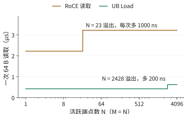
图 7-34: 一次 64 B 读取的延迟随活跃端点数的变化，片上缓存 256 KiB。逐对连接在 23 个端点处上升 1000 ns，端点加通道在 2428 个端点处上升 200 ns。横轴为对数坐标。
