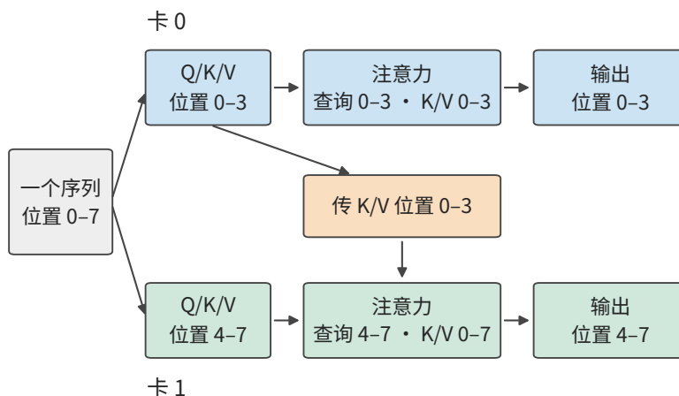
图 6-11：每张卡保存自己那段位置的 Q、K、V。因果注意力下，卡 1 的查询还要用到卡 0 的 K、V，所以 K、V 必须跨卡传递；非因果注意力时两个方向都要传。
