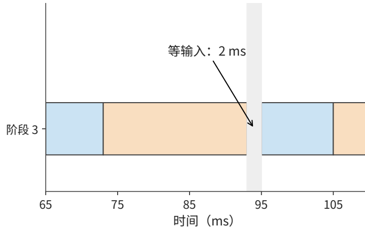
图 10-19: 放大 1F1B 的阶段 3: 第二个 micro-batch 在 93 ms 结束反向, 下一份前向输入于 95 ms 到达, 形成 2 ms 等待。
