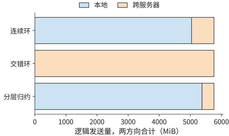
图 7-7: 三方案的逻辑发送总量均为 5760 MiB；橙色跨服务器部分分别为 720、5760、384 MiB。两个方向合计。
