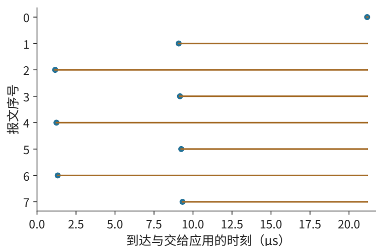
图 7-47：序号 0 丢失后按算例等待时间重传，其他七个报文保留在接收方。只补发缺失报文后，约 21.2 \mu\text{s} 全部可交付。圆点表示报文到达，横线表示到达后等待缺口补齐的时间，纵轴是报文序号。
