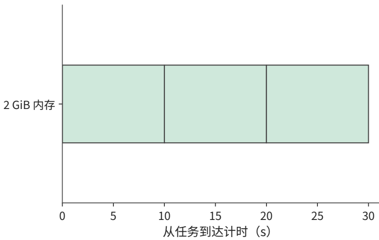
图 11-2：同一任务的环境始终占 2 GiB，持续 30 s，矩形面积为 60 GiB · 秒。等待模型时仍保留环境，因而内存占用持续时间长于工具的 CPU 执行时间。
