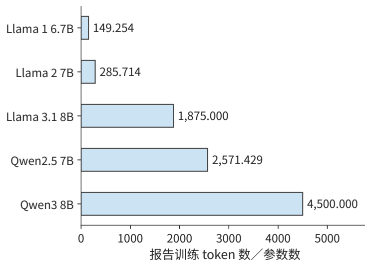
图 3-30 相近参数规模的模型投入不同数量的训练 token。柱值为报告训练数据量除以参数量，Qwen 采用模型系列披露的数据预算。
