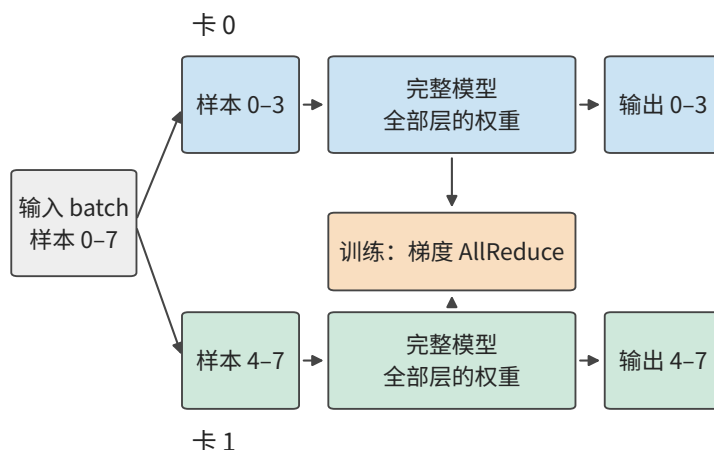
图 6-4：两张卡各保存一份完整模型，分别处理不同样本。推理时两张卡互不等待；训练时两张卡的梯度要先汇合，再各自更新参数副本。
