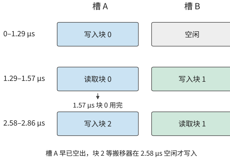
图 5-16：块 0 在 1.29–1.57 \mu\text{s} 使用槽 A，此后槽 A 已经空出；块 2 要等搬移器在 2.58 \mu\text{s} 搬完块 1，才开始写入 A。图中抽取三个时段；1.57–2.58 \mu\text{s} 两个槽里都没有可算的数据，计算单元空等。颜色固定表示槽 A、B，文字说明当前读写的是哪个块。
