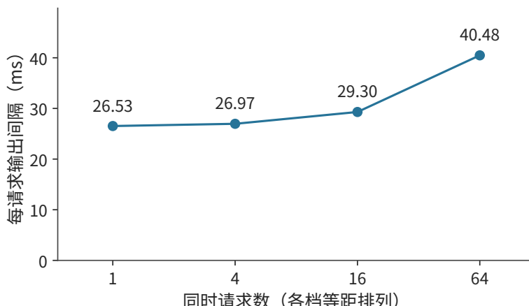
图 1-14 同一组实测中的每请求输出间隔。吞吐增加的同时，单个请求的平均间隔也在增大；两张图分别说明加速器的输出速度和用户的等待时间。
