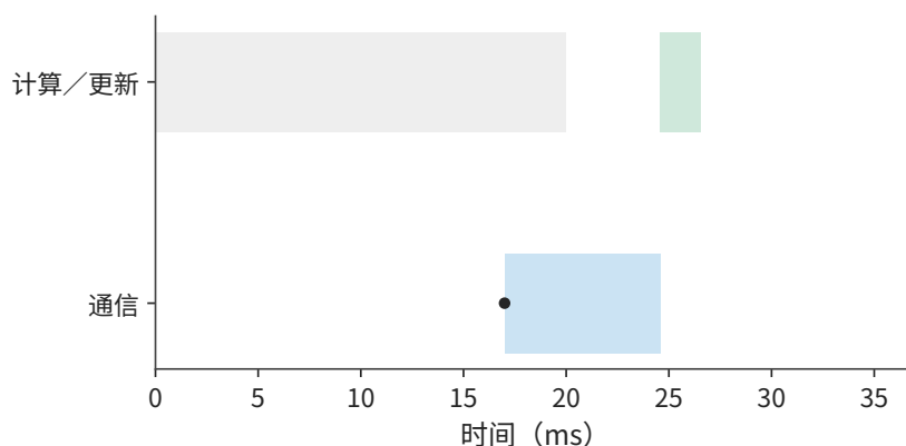
图 7-57：本图把连续环的通信提前到 17 ms 开始，与尚未完成的计算重叠。通信 7.6 ms 超出计算区间，更新等通信结束；整步约 26.6 ms。灰色为计算，蓝色为通信，绿色为更新；圆点为通信数据就绪。
