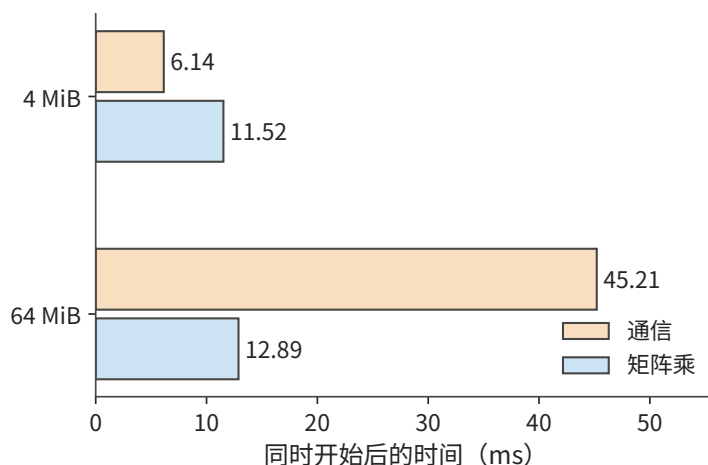
图 6-28: 同一实验中两者同时开始。橙色为通信，蓝色为计算；后续工作等待两者都完成。4 MiB 的通信增至 6.14 ms，仍藏在计算之内；64 MiB 的通信增至 45.21 ms，计算也增至 12.89 ms。
