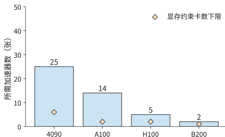
图 10-5: 矩阵计算效率为 50% 时所需的卡数。三图使用相同的型号顺序、纵轴范围、任务与 30 天执行期限。各下限均以卡数计量；容量项是显存约束要求的最少卡数。
