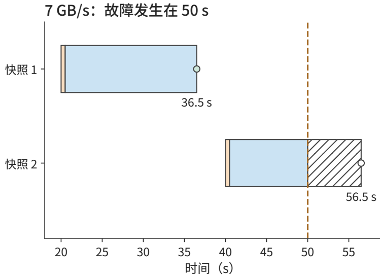
图 10-33：两份 112 GB 快照以 7 GB/s 写入，各先花 0.5 s 复制到缓冲（橙色），随后上传（蓝色）。50 s 故障时第一份已提交，第二份尚未提交；斜线为无故障时剩余上传，空心点为原定提交时刻。
