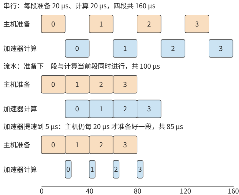
图 5-26：每段主机准备 20\ \mu\text{s} 。串行执行时两种资源轮流工作；流水后主机准备下一段时加速器计算当前段，每 20\ \mu\text{s} 完成一段；加速器提速到 5\ \mu\text{s} 后，每段仍要等主机准备好，加速器大部分时间空闲。图中只画前四段，正文算例为 100 段。
