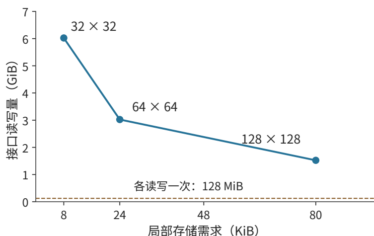
图 5-8：每个点标出输出块形状。扩大输出块能减少跨接口的重复读取，但需要更多局部存储。虚线为三份矩阵各经过一次的 128 MiB；比较条件为 k=32 、单组输入缓冲、各输出块独立读取输入。
