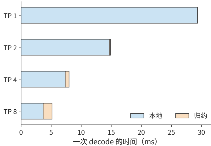
图 6-25：根据式 (6-5) 和环形归约模型绘制的单步时间。本地内存访问随卡数增加而减少，归约时间则增加；条形总长度为单步执行时间。本地项包括权重与 KV 读取，归约项是卡间集合通信。
