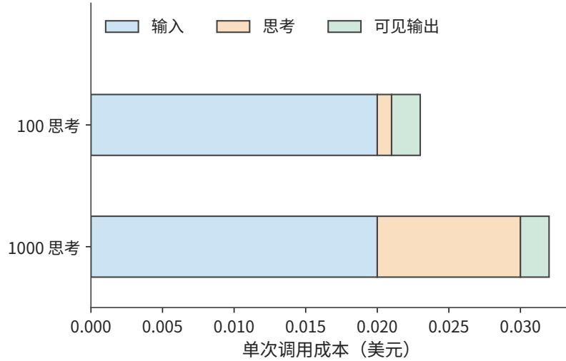
图 11-29：两次调用的输入和可见输出相同，只改变思考长度。橙色成本缩短到原来的十分之一，蓝色和绿色成本保持不变，所以总成本由 0.032 美元降到 0.023 美元，减少约 28%。价格和 token 数见例 11-5。
