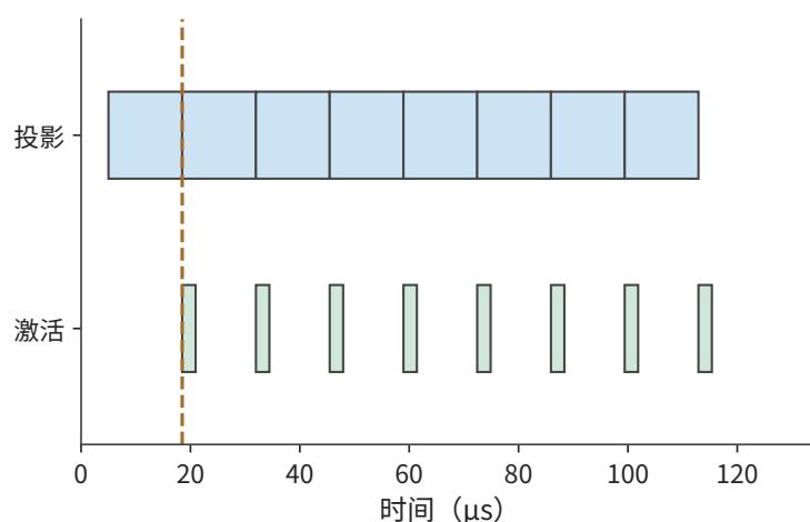
图 5-37：矩阵与向量资源独立、缓冲充足。每个任务另计 0.7 \mu\text{s} 调度与通知，首块投影完成后即可激活；投影首尾相接，激活只在每块投影之后短暂工作，八块流水约 115 \mu\text{s} 结束。
