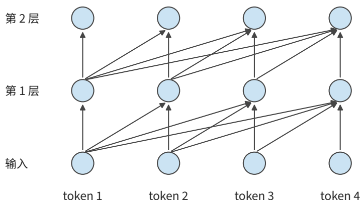
图 2-2 因果 Transformer 的层间依赖。各查询读取上一层中允许访问的位置；上一层完成后，同一层的已知输入 token 可以并行计算。
