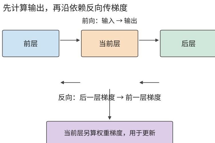
图 3-22 训练沿前向依赖计算输出，再沿反向依赖传递梯度。当前层既向前层传输入梯度，也计算自己的权重梯度，供优化器更新。
