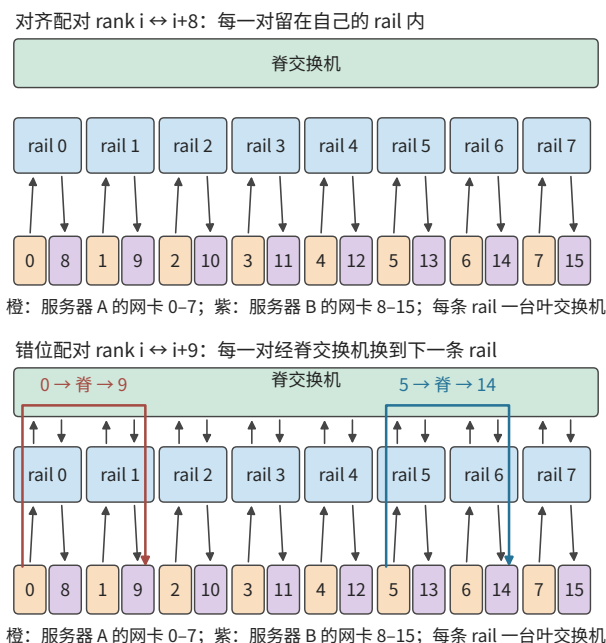
图 7-14：八条 rail 画成八条竖直车道，每条车道里是一台叶交换机和两台服务器上编号相同的网卡。上半图按 rank i 与 rank i + 8 配对，每一对的字节留在自己的车道里，只经过一台叶交换机；下半图按 rank i 与 rank i + 9 配对，每一对都要从第 i 条 rail 经脊交换机换到第 i + 1 条 rail，每个方向 192 MiB 全部经过脊层。
