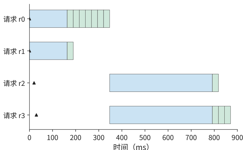
图 8-5：固定 batch 等待整组结束，再接纳 r2、r3。蓝色为 prefill，绿色为 decode，三角为到达时刻。各色带宽度为整次调度迭代耗时，时间按 RTX PRO 6000 上的实测拟合计算。
