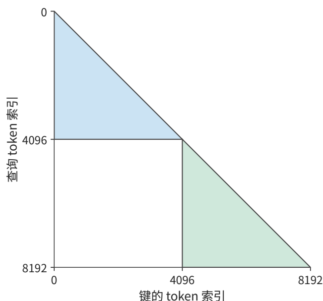
图 10-28：两条 4096 个 token 的序列的因果注意力配对。每个查询 token 读取本序列中不晚于自己的位置，形成两个三角形；两条序列的注意力计算彼此独立，总配对数为 16781312。
