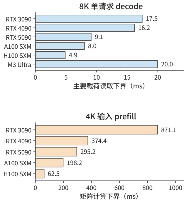
图 4-36 同一 Qwen3-8B 的两种阶段预算。单请求 decode 更直接反映读取带宽，4K prefill 的矩阵预算更直接反映匹配精度的矩阵速率。两图横轴分别标注所计算的时间。
