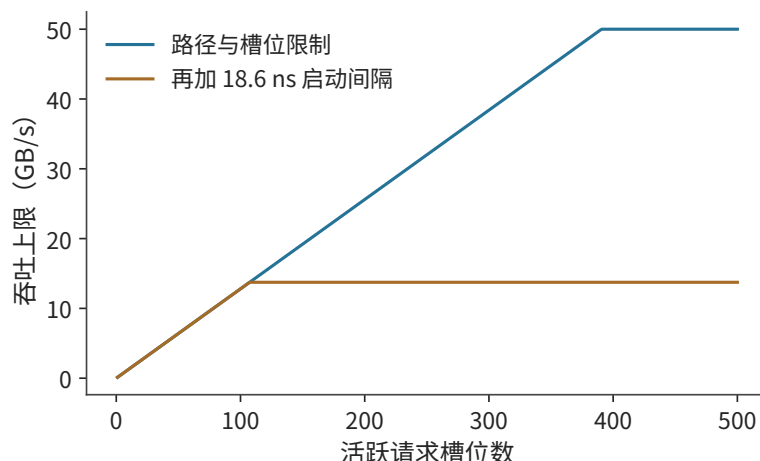
图 7-26: 蓝线只考虑链路和槽位, 橙线再加入每 18.6 ns 发起一次请求的约束。增加槽位使蓝线升高, 橙线仍受约 13.7 GB/s 的提交速率限制。
