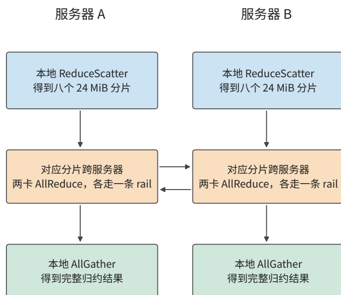
图 7-6：每台服务器先把本机八份贡献归约成分片，再和另一台服务器交换对应的分片，最后在本机收集完整结果。每列从上向下执行，横向箭头表示跨服务器交换，每对参与者各用一条 rail。
