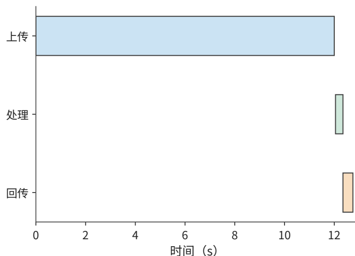
图 12-3: 整图串行: 30 MB 全部上传并传播到服务器后才处理, 随后回传 5 MB。上行 20 Mbit/s、下行 100 Mbit/s、单向传播 0.05 s, 任务于 12.8 s 完成。
