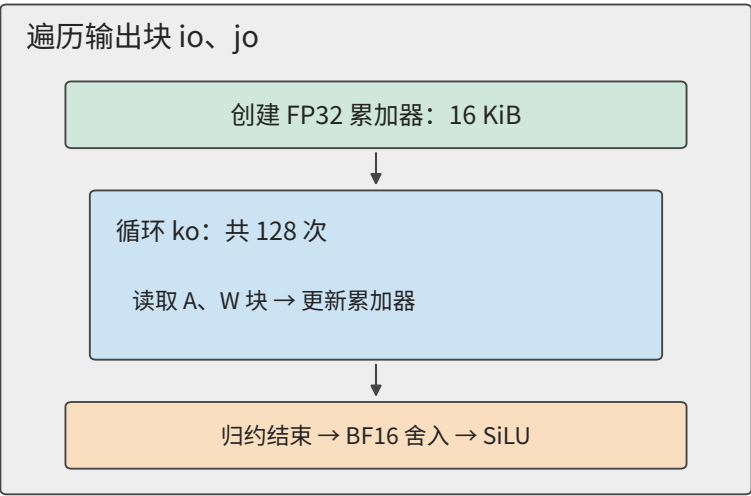
图 5-21：循环层级决定临时数据需要保存多久。外层选输出块，创建 16 KiB 累加器；内层 ko 反复读取 A、W 块，全部归约结束后再舍入并计算激活函数。
