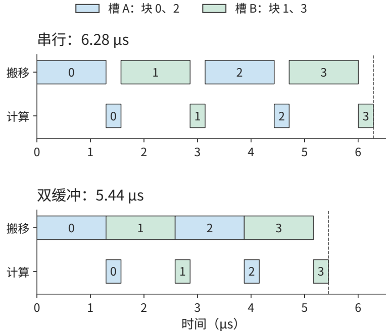
图 5-17: 两个输入槽交替复用, 让搬移与计算重叠。H100 一个 SM 上每块搬移 1.29 \mu\text{s} 、计算 0.28 \mu\text{s} , 资源独立, 忽略同步开销; 同一颜色表示同一槽。重叠只藏住了计算, 完成时间由首尾相接的搬移决定。
