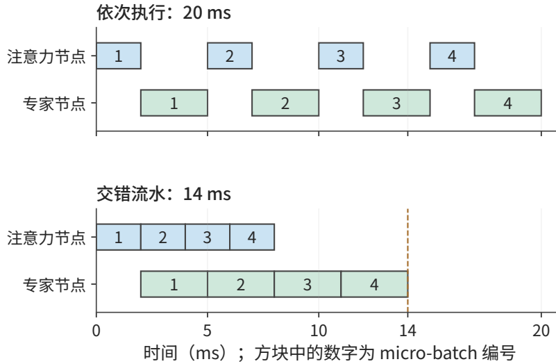
图 9-17: 四个 micro-batch 在注意力节点与专家节点间执行, 每个 micro-batch 注意力 2 ms、专家 3 ms, 忽略交接。上图依次执行, 两个节点轮流空闲; 下图交错执行, micro-batch 1 做专家计算时 micro-batch 2 做注意力。流水稳定后, 专家节点连续工作, 每 3 ms 完成一个 micro-batch。
