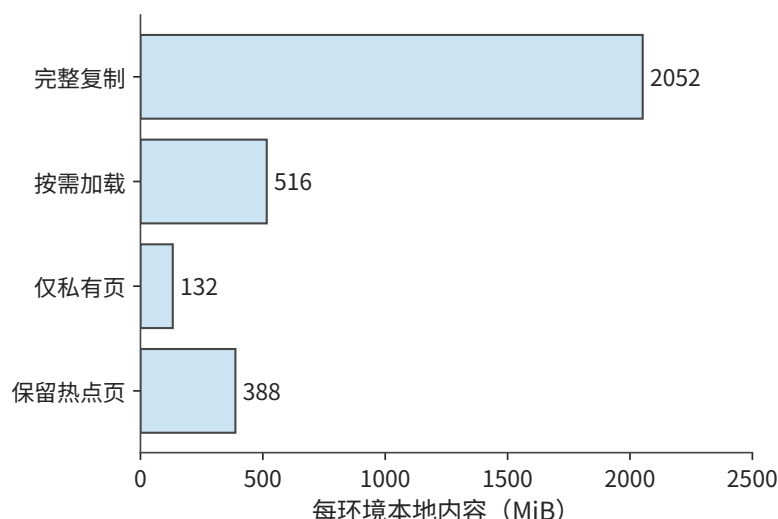
图 11-10：四种方案采用相同的横轴尺度，比较每个环境本地保存的数据。另有一份共享的 2 GiB 模板，不计入各环境的柱长。数值来自例 11-2；管理开销为每环境 4 MiB。
