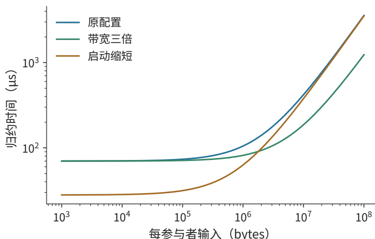
图 7-60：原配置每轮启动 5\ \mu\text{s} 、带宽 50\ \text{GB/s} 。绿色将带宽增至三倍的 150\ \text{GB/s} ，橙色将每轮启动减至 2\ \mu\text{s} ；数据量小时主要受启动影响，数据量大时主要受传输影响。
