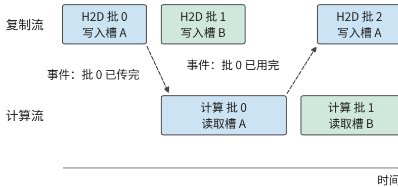
图 5-2: 复制流依次传入各批输入，计算流读取它们。计算批 0 要等“批 0 已传完”事件；批 2 要重新写入槽 A，必须等“批 0 已用完”事件。虚线箭头表示等待事件，不搬移数据。两个槽的交替使用在第 5.3.2 节展开。
