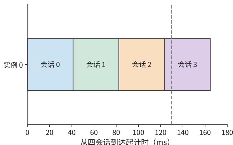
图 6-50: 单会话缩短到约 41.2 ms，四会话依次执行，最后一个约 164.7 ms 完成。三图横轴使用同一尺度。本图使用一个 TP8 实例，共八张卡，每个会话续写八个 token；虚线为 130 ms 期限。
