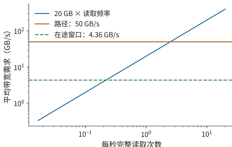
图 6-46: 完整读取 20 GB 的频率与平均带宽需求。路径带宽为 50 GB/s；每事务返回 256 bytes、往返 7.52 \mu s 时，128 个在途事务将有效带宽限制到约 4.36 GB/s。
