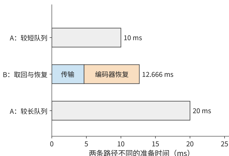
图 9-41：缓存亲和性与空闲执行位置的比较。A 保留全局 KV 与编码器 SWA；B 需要 4.666 ms 全局传输和假设的 8 ms 编码器恢复。两端共同的解码器重放等后续工作略去，只比较不同的串行准备时间；A 的排队时间从 10 ms 增到 20 ms 时，更快的方案由 A 变为 B。灰色为等待队列，其他色块分别为全局状态传输与编码器局部状态恢复。
