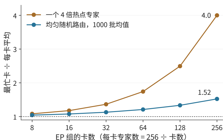
图 9-22：最忙卡行数与每卡平均行数之比随 EP 组卡数的变化。橙线为一个 4 倍热点专家，不含随机波动，可以直接手算；蓝线为均匀随机路由，是固定种子模拟 1000 批的平均值。256 个专家按编号均分，不设副本；横轴为对数刻度。
