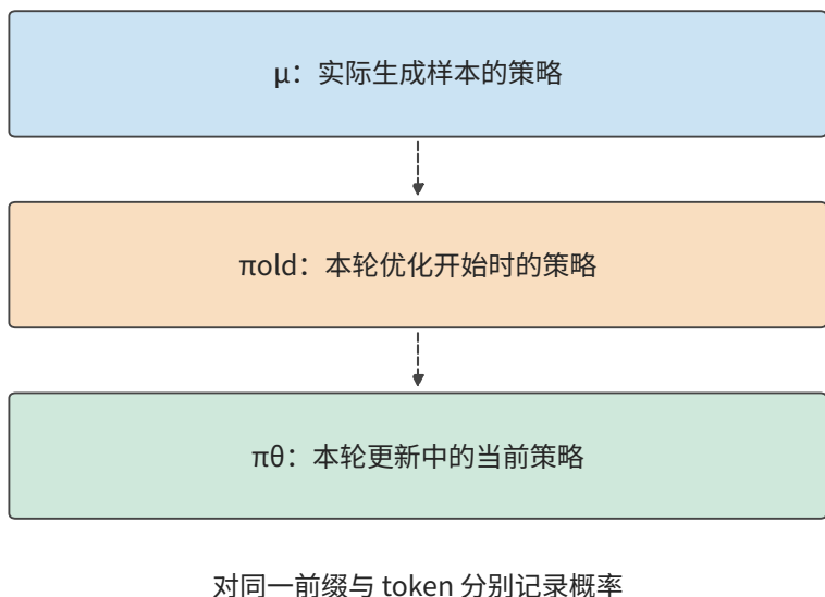
图 10-41： \mu 产生训练样本， \pi_{old} 标识本轮优化的起点， \pi_{\theta} 随本轮更新变化。虚线表示版本演进顺序。三个概率必须针对同一前缀与同一 token 计算。
