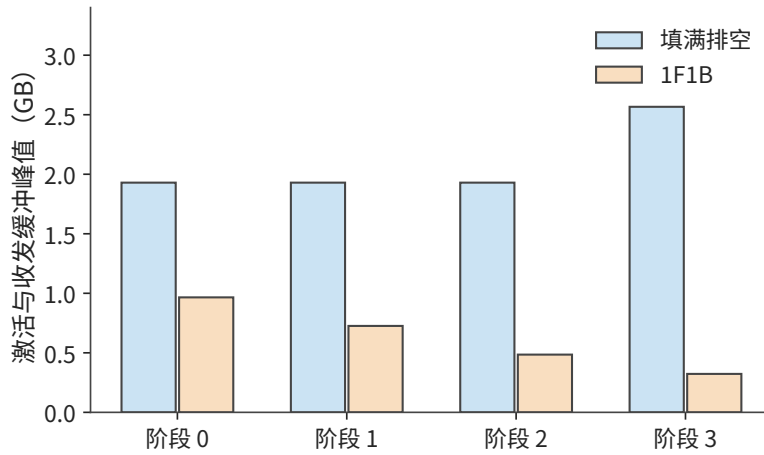
图 10-20: 两种调度中各阶段的激活与收发缓冲峰值。提前反向使激活更早释放, 最大值由约 2.57 GB 降到 0.97 GB。
