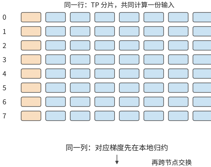
图 7-61：64 卡超节点由八个张量并行组组成。同一行的八张卡处理同一 micro-batch 的不同模型分片；同一列的八张卡先在节点内汇合对应的梯度，再与其他超节点交换同一分片。一个训练作业用上全部的卡，不等于全部的卡组成一个张量并行组。
