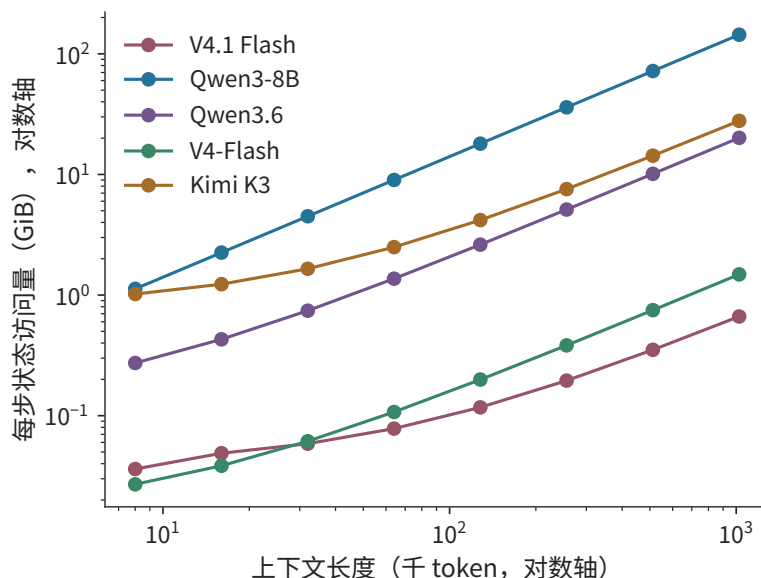
图 2-19 同一组模型每步计入的状态访问。逐 token 上下文读取，递推矩阵计一读一写；这些是指定路径的逻辑数据量，用于比较容量与访问的不同增长方式。每步指为一个请求生成下一个 token 的一次 decode；纵轴不包含模型权重读取。
