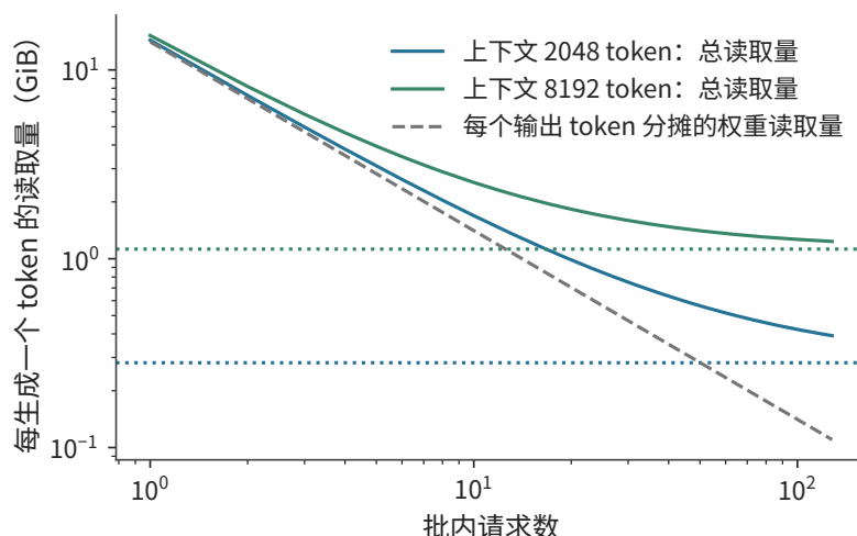
图 8-3: 批处理怎样减少每生成一个 token 所需的读取量。横轴为同时生成的请求数, 纵轴为整批读取字节数除以本轮输出 token 数。蓝、绿实线分别对应每条请求已有 2048、8192 个 token 的上下文, 包含权重与 KV 读取; 同色水平点线仅表示该长度下的 KV 读取量。灰色虚线表示批内共用的权重读取量除以请求数。模型为 Qwen3-8B, 使用 BF16; 每份矩阵权重每轮读取一次, 各请求的 KV 独立。两轴均为对数刻度。
