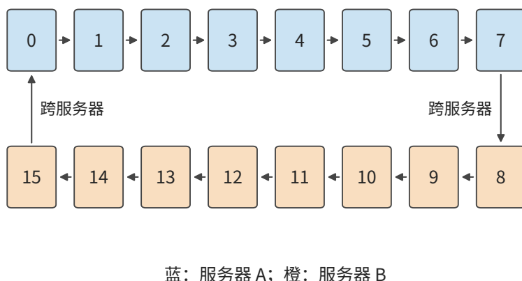
图 7-4：连续环将同一服务器内的参与者排在一起。十六条有向边中只有 7→8 与 15→0 跨服务器，跨服务器流量集中在两张网卡上。颜色表示参与者所在服务器。
