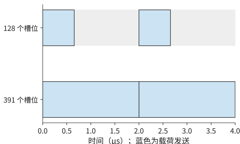
图 7-25：128 个槽位在约 0.66 \mu s 内全部用完，要等最早的槽位在 2 \mu s 释放后继续提交。391 个槽位足以覆盖等待。蓝色表示载荷发送，灰色表示链路空闲。
