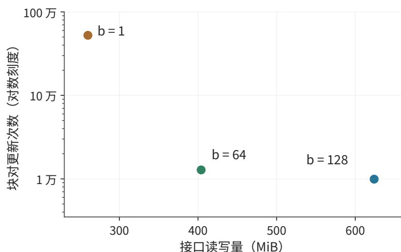
图 5-20：快速缓冲为 RTX PRO 6000 一个线程块的 99 KB 共享内存，序列长 8192、头维度 128，无掩码；每个点对应正文表格的一种 K/V 块大小。横轴为缓冲与下一级存储之间的访问量，纵轴为在线更新次数，采用对数刻度。从 b=64 的点移到 b=1 的点，读取减少，更新次数却约增至 41 倍。 b 表示一个 K/V 块中包含的 token 数。
