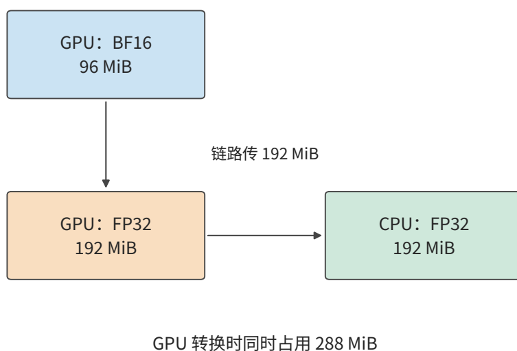
图 10-15：先在 GPU 将 96 MiB BF16 梯度转为 192 MiB FP32，再传到 CPU。转换时输入与输出共存，GPU 峰值为 288 MiB。
