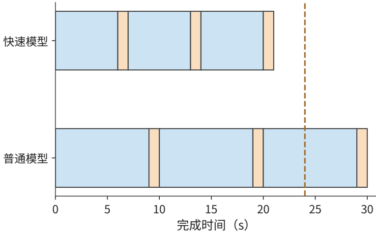
图 11-40：两种方案均在模型调用期间准备环境，工具执行均为每轮 1 秒。模型调用从每轮 9 秒降至 6 秒，三轮结束时刻从第 30 秒移到第 21 秒，从 24 秒期限之后提前到期限之内。
