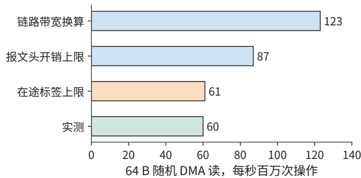
图 7-28: KV-Direct 平台上 64 B 随机 DMA 读的上限与实测。链路带宽换算为每秒 1.23 亿次, 报文头开销把上限压到 8700 万次, 64 个标签除以 1050 ns 往返只允许 6100 万次; 实测 6000 万次, 说明在途标签数是这个平台上读的瓶颈。
