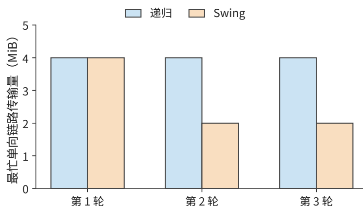
图 6-33: 把所有发送方的数据累加到各条有向链路上, 取每轮的最大值。递归前三轮均为 4 MiB, Swing 为 4、2、2 MiB。
