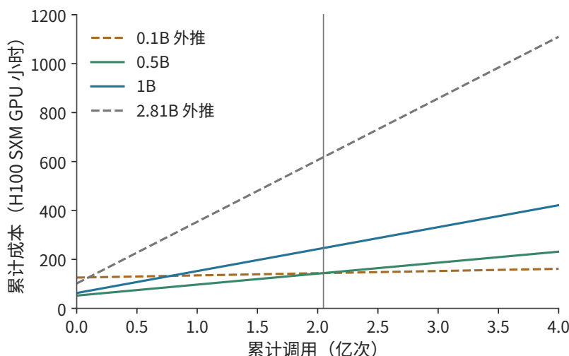
图 3-29 训练与服务累计成本的题设比较。截距是训练投入，斜率是单次调用成本；虚线标出超出拟合参数或数据范围的方案，竖线为约 2.048 亿次的成本交点。图例中的 B 表示十亿个模型参数；纵轴为按 40% MFU 折算的 H100 SXM GPU 小时。
