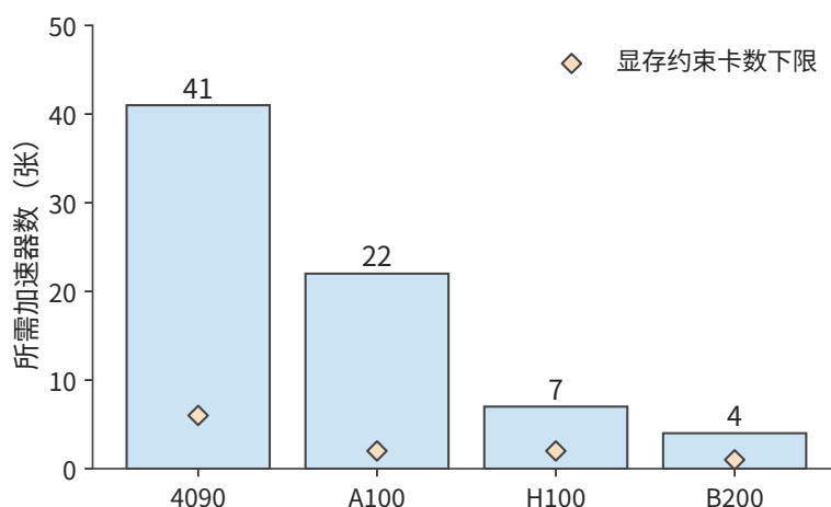
图 10-3：矩阵计算效率为 30% 时所需的卡数。任务为 Qwen3-8B 处理 100B token，序列长 8192，全部 30 天用于执行；蓝柱为计算需求，橙色菱形为训练状态容量下限。A100 为 80 GB SXM，H100 为 SXM。
