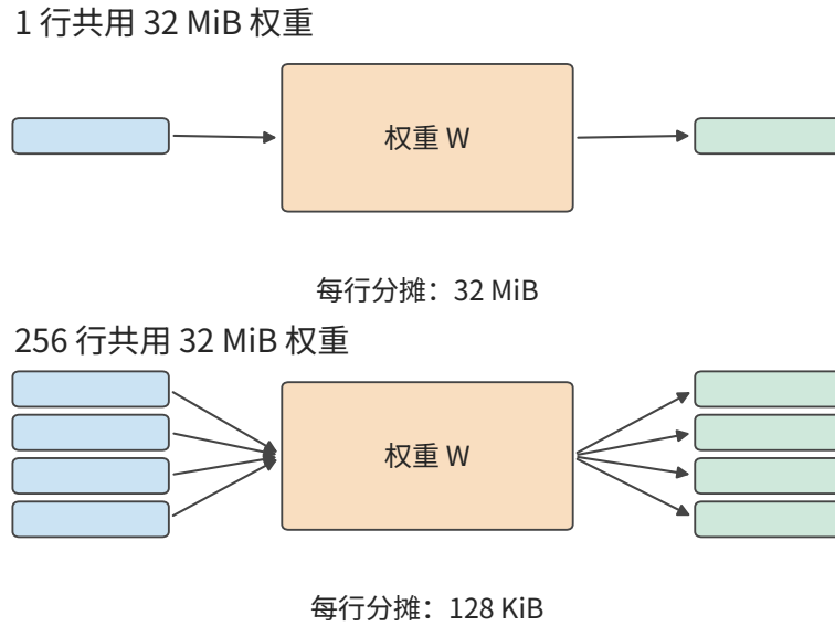
图 4-1 两种调用都使用同一份 32 MiB 权重。上方是一行输入，下方以部分条带示意 256 行；每行分摊的权重读取从 32 MiB 减至 128 KiB。
