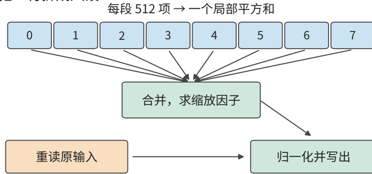
图 5-11：上行由一组处理完整一行，输入保留到归一化结束；下行把一行分为八段，先求局部和，再合并，最后重读输入并归一化。每行 4096 个 BF16 元素；图中仅画一行，推广到 1024 行时，第一阶段任务数由 1024 增至 8192。橙色框表示增加的原输入读取。
