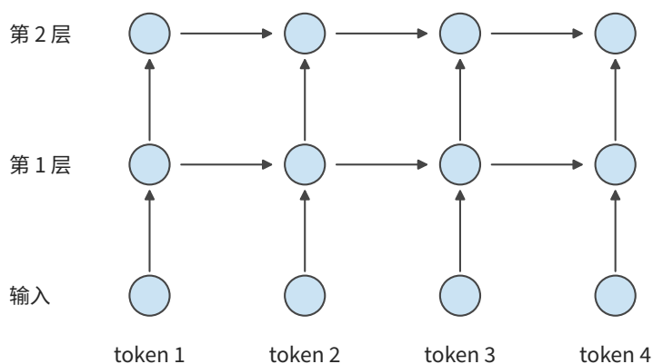
图 2-1 循环神经网络的依赖。相同颜色的圆点表示各 token 位置的计算，箭头指向需要前一结果的节点；同层 token 位置沿横向逐次推进。
