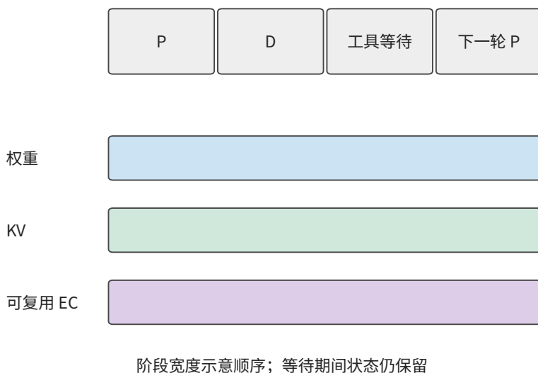
图 9-5：计算暂停期间，状态仍需保留。示意同一请求从 prefill、decode 到工具等待和下一轮的状态驻留时间；横轴按阶段排列，不表示相等时长，EC 仅在在有视觉输入时出现。E 为视觉编码，EC 为保存的视觉编码结果，P 为 prefill，D 为 decode。
