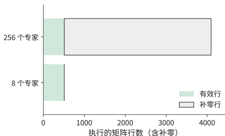
图 4-10 相同 512 行有效输入在全部专家上的执行量。分散到 256 个专家后总计执行 4096 行，集中到八个专家时只执行 512 行。
