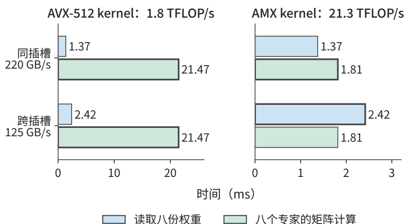
图 9-15: 八个 Qwen3-235B-A22B 专家各处理 128 个 token 时，单颗 Xeon Platinum 8452Y 上的两项时间：读取八份 BF16 权重共 288 MiB，矩阵计算共 38.7 GFLOPs。粗框标出较长的一项，即这条路径的耗时下界。左右两图横轴刻度不同；AVX-512 与 AMX kernel 的算力、同插槽与跨插槽带宽均为论文实测值。
