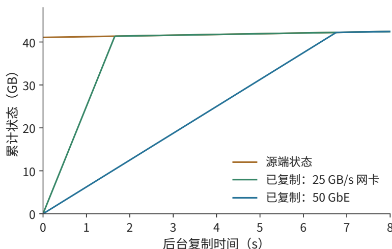
图 9-43：后台复制需要赶上仍在增长的状态。开始时待复制状态为 41.1 GB，源端每秒增长约 0.172 GB；目标经 25 GB/s 的网卡约 1.65 秒赶上，经 6.25 GB/s 的 50 GbE 约 6.76 秒赶上。曲线相交前，垂直距离就是尚未复制的数据量；相交后，目标只需跟随源端的新增状态。
