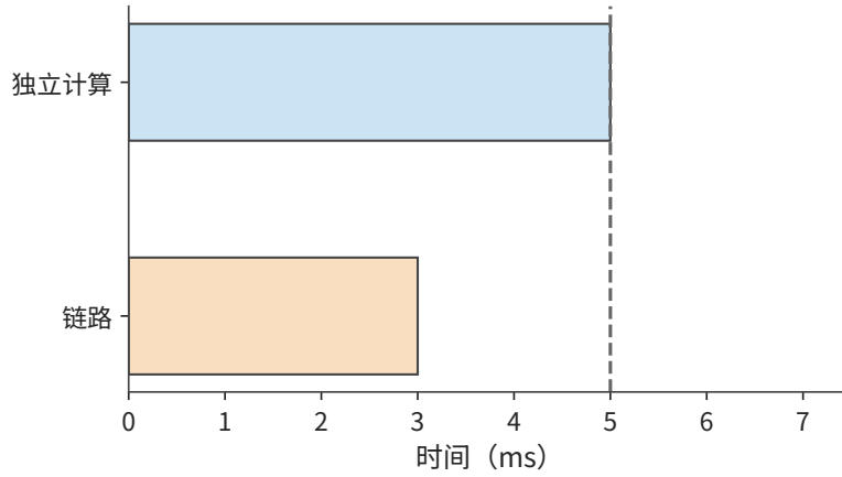
图 10-25：链路空闲时，3 ms 归约（橙色）可以在 5 ms 独立计算（蓝色）结束前完成。虚线标出计算结束。
