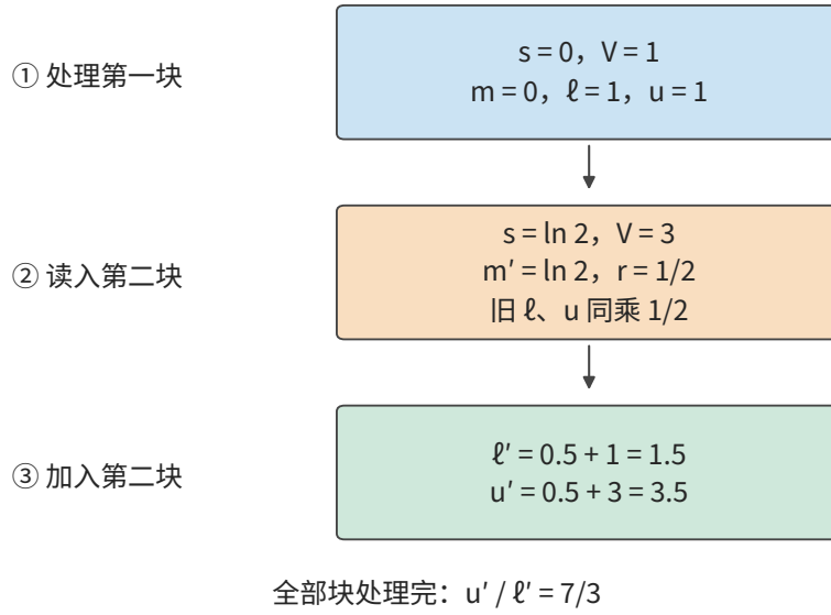
图 5-19: 两个块的分数分别为 0、 \ln 2 ，值分别为 1、3。最大值增大后，将旧指数和与旧加权值同时乘以 1/2 ，再加上新块的贡献，最后才做除法。箭头传递的是统计量，旧分数无需保留。 m 是已处理分数的最大值， \ell 是以 m 为基准的指数和， u 是对应的值向量加权和， r 是更换最大值基准时的缩放系数。
