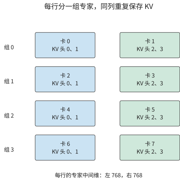
图 6-17：八张卡排成四个专家分组，每组两卡沿专家中间维分工。同一列的注意力头与 KV 重复四份；每组因此都能在本地产得到相同的专家输入。
