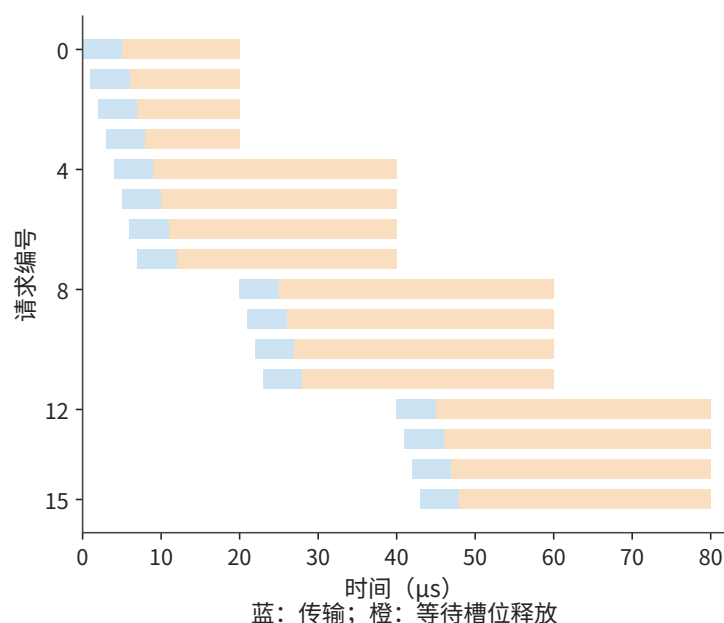
图 7-38：蓝色表示提交到传输完成，橙色表示等待软件处理完成通知，橙色结束才释放槽位。所有请求的时刻取自事件记录。
