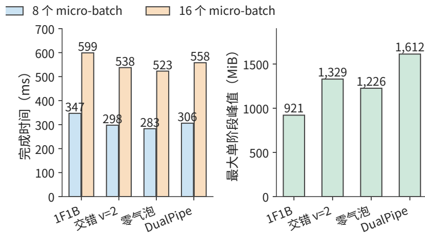
图 10-24: 四种流水线调度在八个与十六个 micro-batch 下的完成时间，以及八个 micro-batch 时各调度最大的单阶段激活与收发缓冲峰值。四种调度使用相同的前向 10 ms、反向 20 ms、边界传输 1 ms、参数更新 1 ms 条件。
