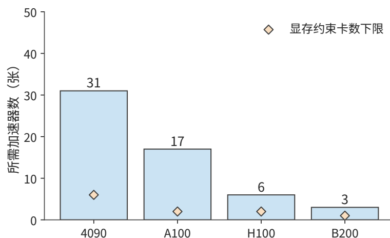
图 10-4: 矩阵计算效率提高到 40%，同一任务所需的卡数下降；橙色菱形仍表示状态容量下限。各下限均以卡数计量；容量项是显存约束要求的最少卡数。
