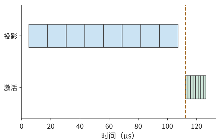
图 5-36：粗粒度执行先完成八块投影，再启动八块激活。按 RTX PRO 6000 的矩阵峰值与显存带宽，每块投影约 12.8 \mu\text{s} 、激活约 1.76 \mu\text{s} ，两次 kernel launch 各 5 \mu\text{s} ；竖线为激活开始。
