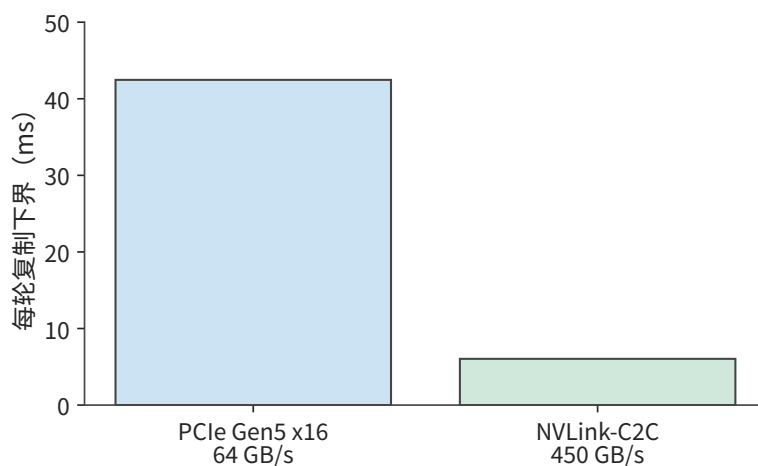
图 8-25: 每轮复制量保持为 2592 MiB (2.72 GB)。经 PCIe Gen5 x16（每方向 64 GB/s）至少需要约 42.5 ms，经 GH200 的 NVLink-C2C（每方向 450 GB/s）至少需要约 6.0 ms。
