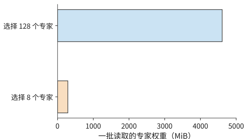
图 6-19：64 个 token、每 token 八个专家，共 512 次分派。均匀覆盖与集中选择的有效计算量相同，被选中专家的权重读取相差 16 倍。每个专家 BF16 权重为 36 MiB，批内读取一次。
