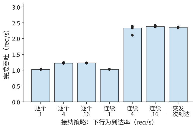
图 8-33: 每种接纳与到达条件使用三个 16 请求窗口。柱为全部完成请求的吞吐中位数，圆点为各窗口结果。时间从计划到达起计算。
