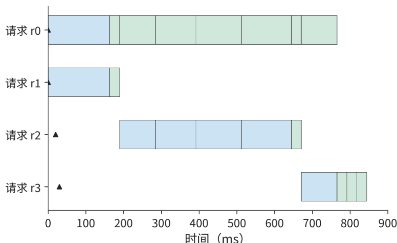
图 8-7: 将长输入分块处理，每轮先安排已有请求生成，再处理一块新输入。每行是一条请求；蓝色为输入处理，绿色为输出生成，三角形为到达时刻。分块使最长输出间隔降至约 133 ms，全部请求约 844 ms 完成。横轴与图 8-5、8-6 使用相同时间尺度。
