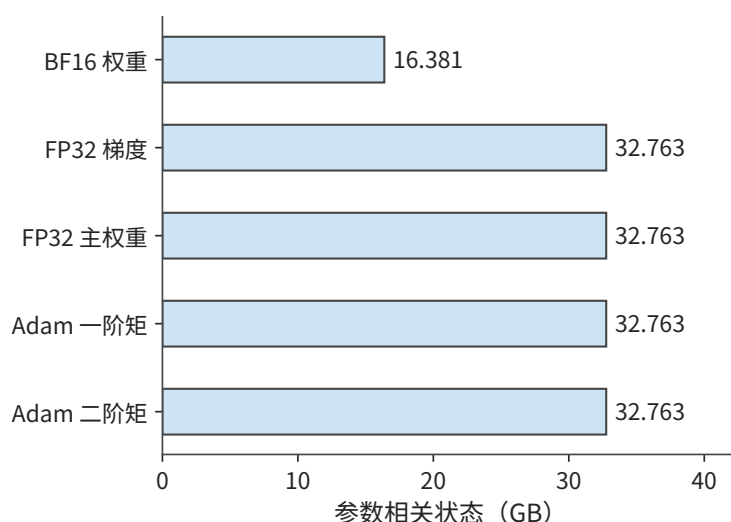
图 3-23 Qwen3-8B 全参数训练的参数相关状态。每参数包括 2 字节计算权重和 4 组 4 字节状态，共 18 字节；激活和工作区的容量需求按各自的生命周期单独计算。
