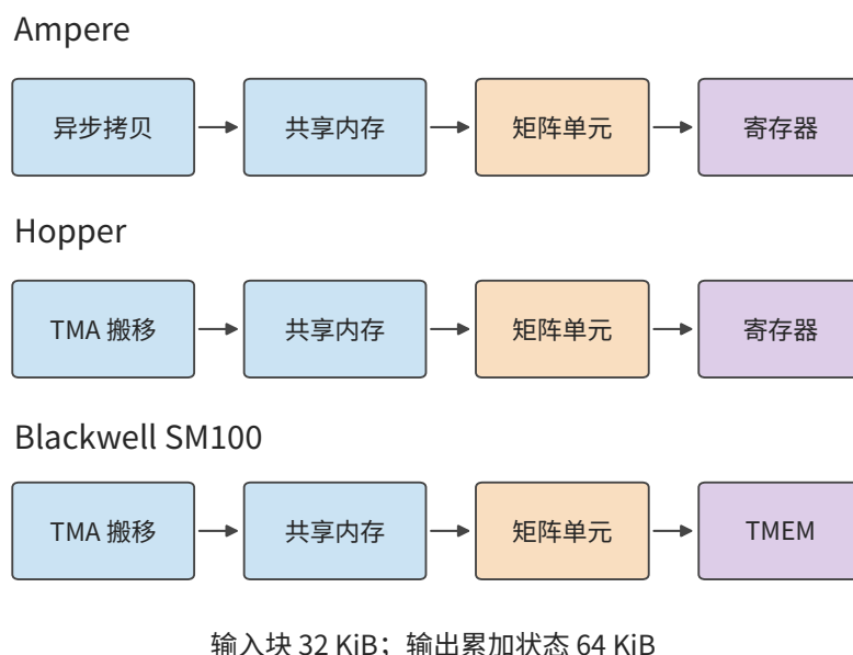
图 4-28 从异步拷贝、TMA 到 TMEM，专门部件承担更多数据准备与累加状态管理。蓝色表示数据存储与搬移，橙色表示矩阵计算，紫色表示累加结果。
