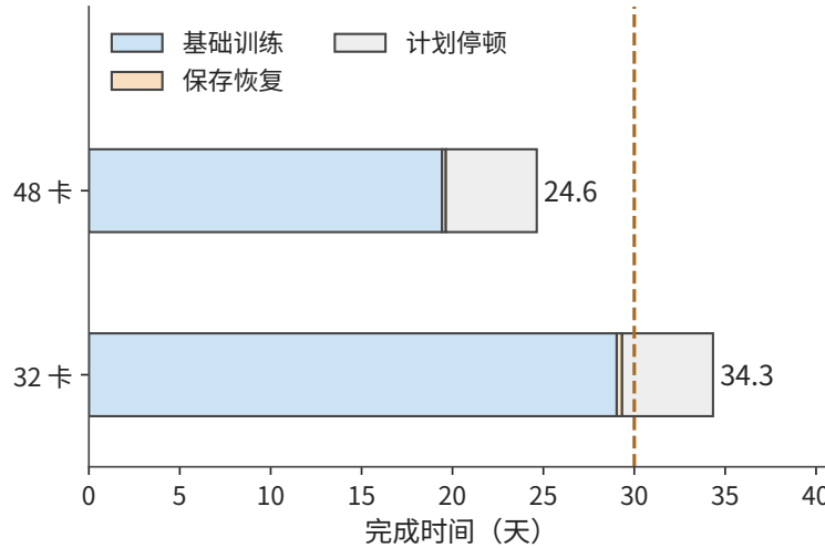
图 10-45：每条横条依次累计基础训练时间、保存与故障恢复的附加时间，以及预留的 5 天计划性停顿。基础训练时间已经包括通信和输入等待；橙色小段为 checkpoint 模型得到的额外耗时。两套方案使用相同任务和全局 batch，虚线标出 30 天期限。
