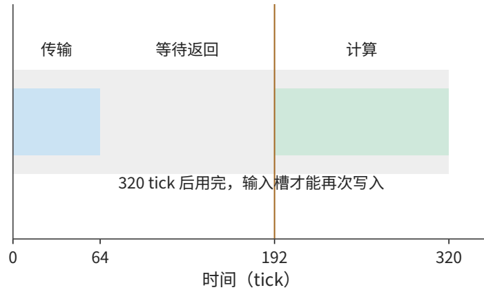
图 4-17 一个输入槽从发起到释放的完整生命周期。传输 64 tick，额外等待 128 tick，数据在 192 tick 就绪，再计算 128 tick，于 320 tick 释放。一个 tick 为 B200 SM 的一个时钟周期。
