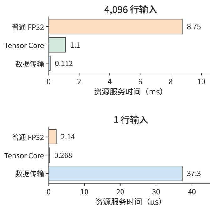
图 4-26 同一 V100 上的 Q 投影。4,096 行时，Tensor Core 大幅缩短矩阵计算；一行时，两条计算路径都短于权重传输。上下两组使用分别标注的时间单位。
