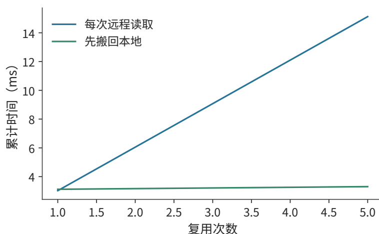
图 7-22：每次读取完整 144 MiB 快照时，两种方法的累计耗时。先搬回本地需要一次固定成本，从第二次读取开始节省时间。
