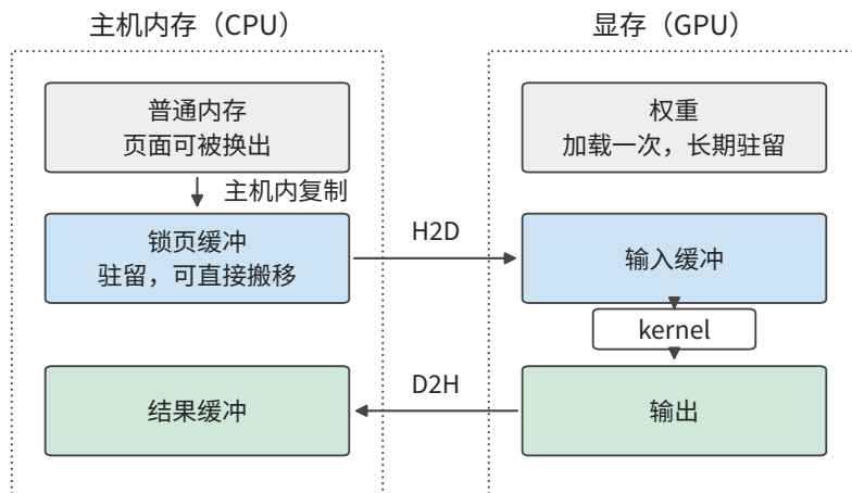
图 5-1: H2D 把输入从主机的锁页缓冲搬进显存, D2H 把结果搬回主机; 权重加载一次后留在显存, kernel 直接读取显存中的输入并写出输出。普通内存中的数据要先复制到锁页缓冲, 才能由复制引擎直接搬移。
