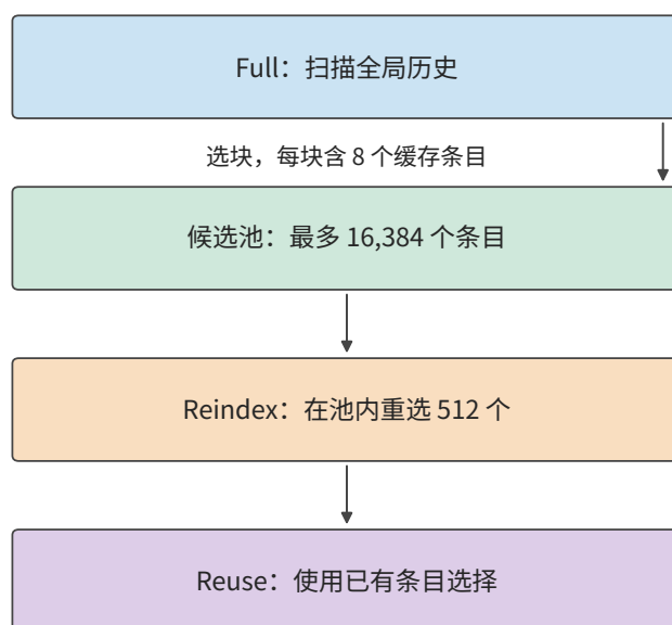
图 2-22 V4.1 解码器的分层缓存条目选择。首个 Full 层先扫描全局，选出最多 16,384 个候选条目；后续 Reindex 在候选内重新选 512 个，Reuse 使用已有选择。示意条目数量不按比例；各层独立 Q 与局部 SWA 未画出。
