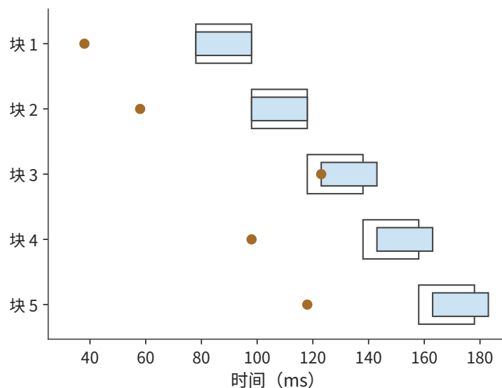
图 12-6：第三块晚到使后续各块的播放时间都推迟 5 ms。每块长 20 ms，模型处理 12 ms、发送 1 ms；通常传播耗时为 5 ms，第三块传播 50 ms，初始缓冲 40 ms。实线段表示实际播放，浅色轮廓表示原定播放区间，圆点表示到达；所有时间均从开始采集第一块起算。图为上述流水线的计算结果，播放器等待缺块而不丢弃。
