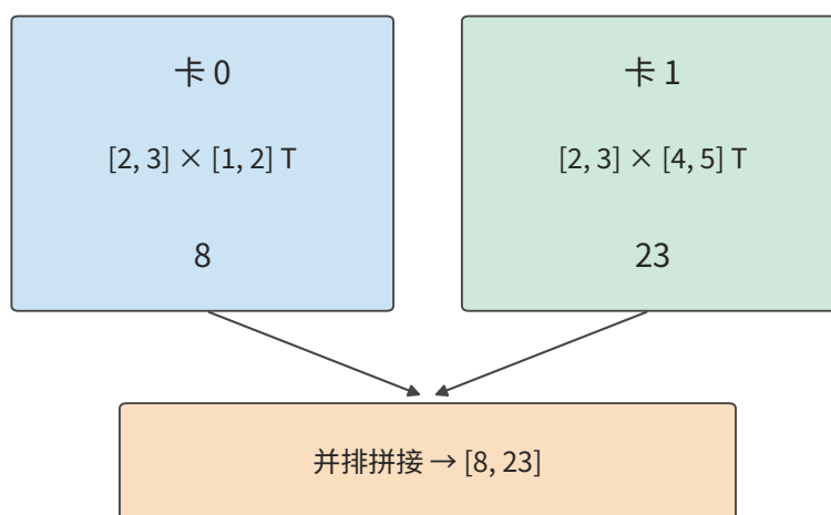
图 6-7：按权重矩阵的列切分时，每张卡使用完整输入，计算不同的输出元素。格内的转置符号 T 表示把方括号中横排的数当作列向量。
