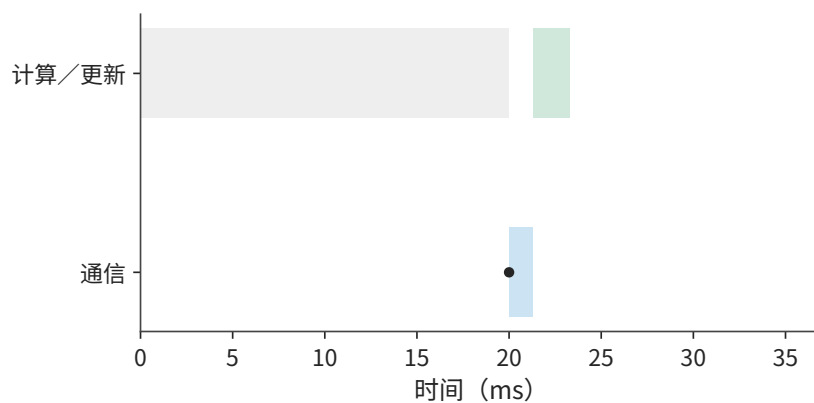
图 7-55：本图改用分层归约，仍按计算、通信、更新串行执行。通信缩短到约 1.3 ms，整步约 23.3 ms。灰色为计算，蓝色为通信，绿色为更新；圆点为通信数据就绪。
