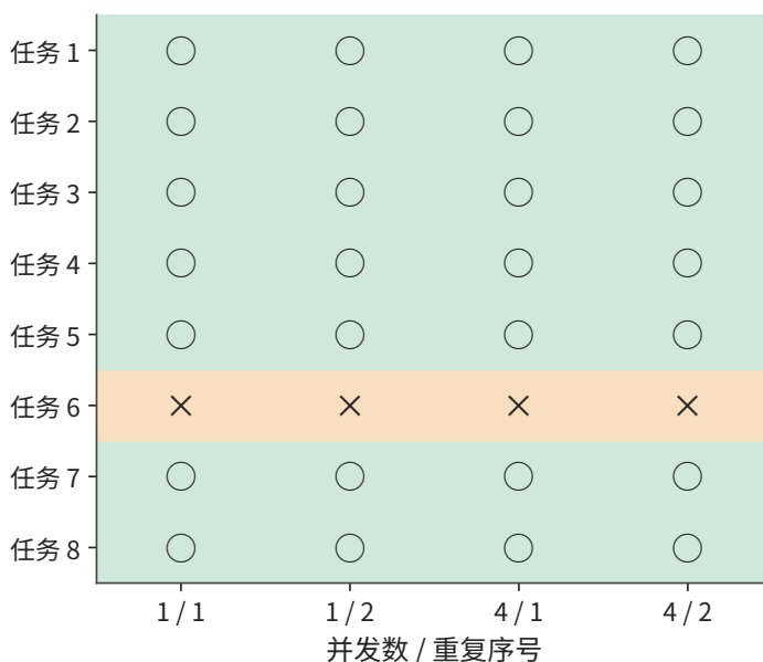
图 8-28：将查询 Q 保持为 BF16，KV 仍用 FP8，共 28/32 正确；答错的题目与 BF16 基线不同。三幅图使用相同任务和列顺序，模型权重均为 BF16。圆圈表示回答正确，叉号表示回答错误；每行对应同一道题，列表示并发数与重复运行序号。
