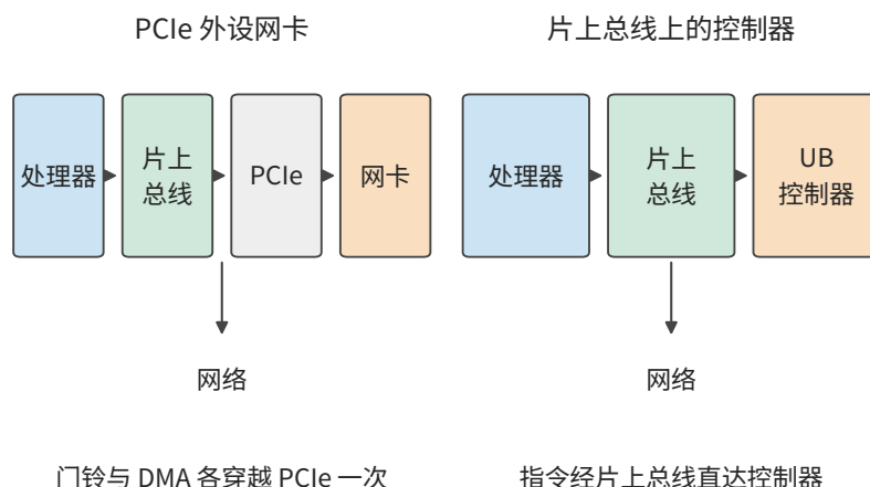
一次远程读取的发起路径
