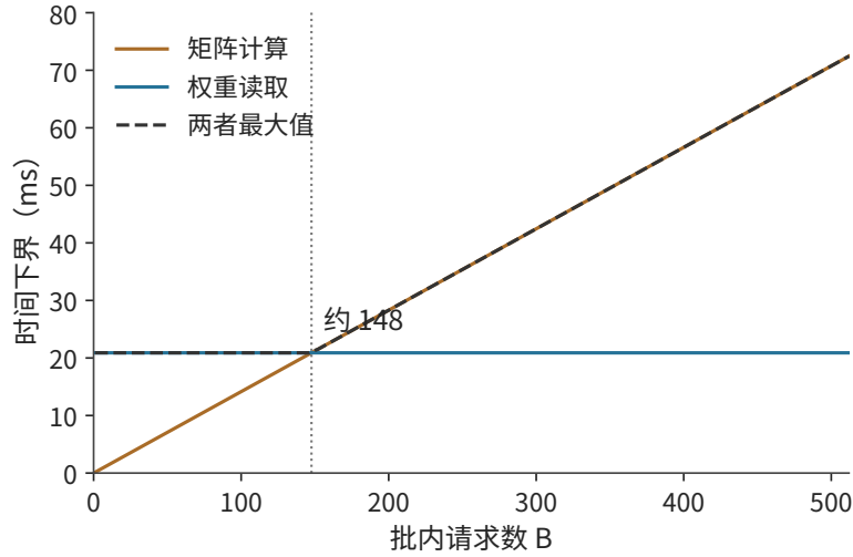
图 1-11 批内请求增加时，矩阵运算量按 2BN 增长，权重读取保持每批 70 GB。约 148 个请求处两项下界相等，随后计算耗时决定整体速度。
