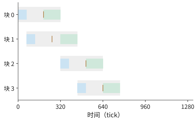
图 4-19 两个输入槽使用相同时间尺度。前两块可提前发起，但第三块到 512 tick 才就绪，第二块在 448 tick 已结束，留下 64 tick 空闲。横轴一个 tick 为 B200 SM 的一个时钟周期；各行对应一个数据块，灰色表示输入槽占用，蓝色表示传输，绿色表示计算，竖标记表示数据就绪。
