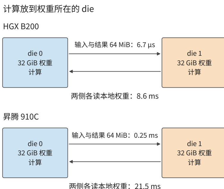
图 4-23 计算放到权重所在的 die 后, 链路上只交换 64 MiB 输入与结果, 两侧各读本地权重。B200 仍约 8.6 ms; 昇腾 910C 从约 127 ms 降到约 21.5 ms。
