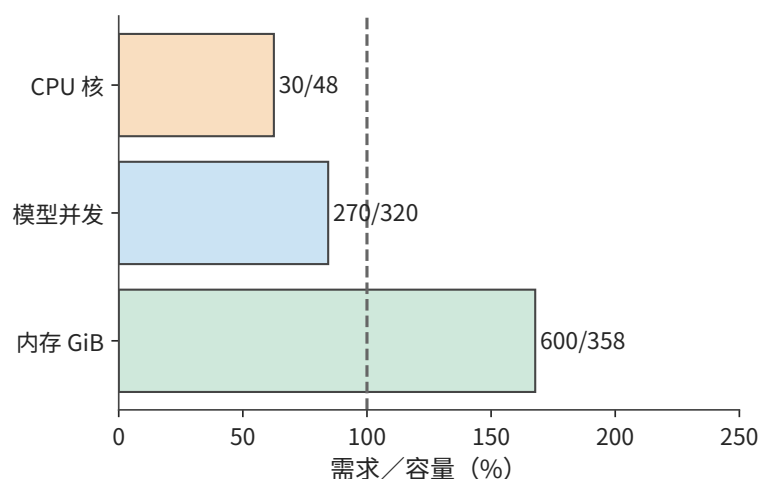
图 11-3：每秒 10 项任务、每次模型调用 9 s 时，三种资源的需求占容量比例。柱末给出需求量/可用容量；虚线为 100%。
