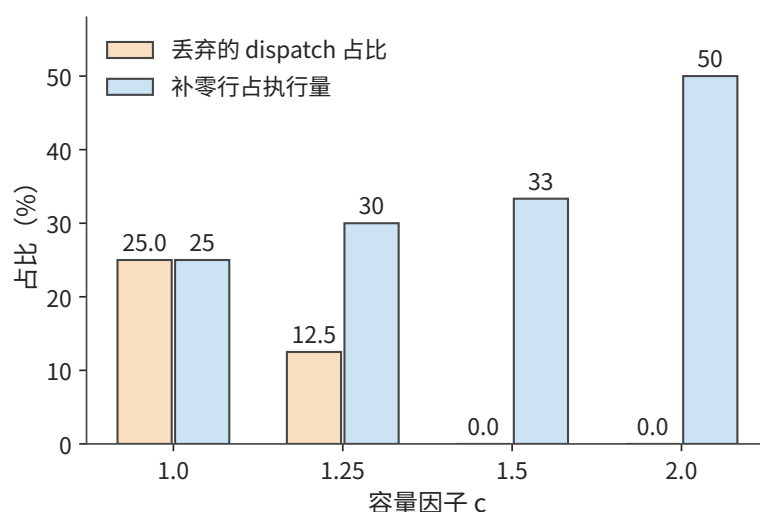
图 10-27: Qwen3-235B-A22B 的路由形状 ( E=128 、 k=8 、8,192 个 token、一半专家 1.5 倍热) 下，容量因子增大时丢弃的 dispatch 占比下降、补零行占比上升。
