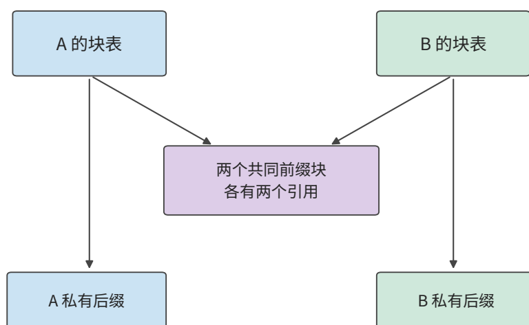
图 8-13: A、B 的两个共同前缀块只保存一次, 各自块表都指向它们。A、B 保留各自的私有尾块; 四条请求实际分配的 KV 容量进一步降至 44 个 token。
