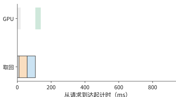
图 9-40：远端链路换成 200 GbE (25 GB/s) 后，首 token 约 137 ms 返回。橙为远端读取，蓝为主存到 GPU；四图均从请求到达起计时，横轴相同。
