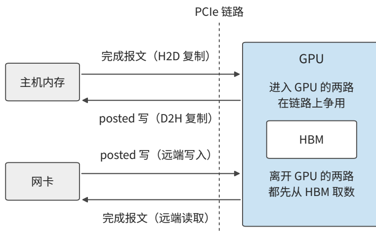
图 7-29: 进入 GPU 的方向上, 网卡的 posted 写与主机内存返回给复制引擎的完成报文争用链路, 前者不等回应, 后者受在途标签限制。离开 GPU 的方向上, D2H 复制的 posted 写与远端读取的完成报文都要先从 HBM 取数, 共用 GPU 内部的发送通路。
