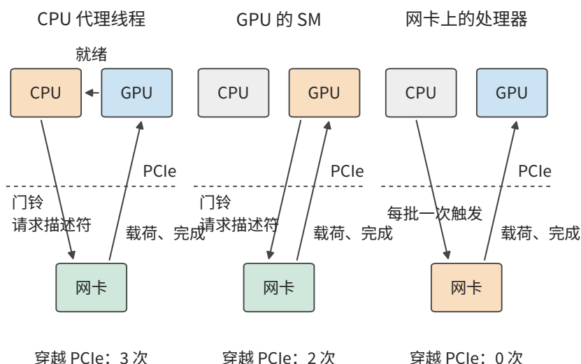
图 6-29：三种发起位置。橙色是构造请求描述符的部件；虚线是 PCIe 边界。CPU 代理线程的控制路径穿越 PCIe 三次，GPU 发起两次，网卡上的处理器零次；发起端的载荷与完成记录在三种方式下都各穿越一次。
