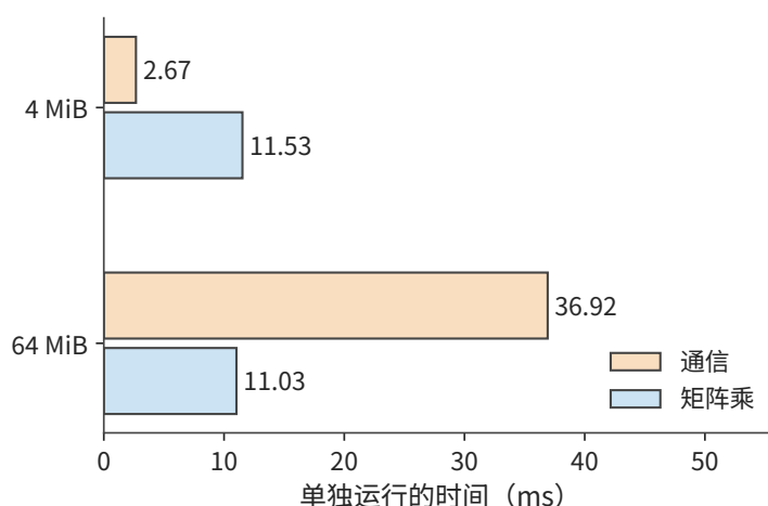
图 6-27：实验 6-5 中通信与矩阵乘单独运行的时间，四个 CPU 进程，五组中位数。4 MiB 通信约 2.67 ms，64 MiB 通信约 36.92 ms，矩阵乘约 11 ms。
