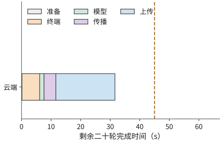
图 12-30: 云端 (H100 SXM): 准备 0.14 s, 二十轮终端 6 s、模型 1.5 s、传播 4 s、上传 20 s, 共 31.6 s。计算更快而传输更久, 比附近工作站慢约 20.6 s, 仍在期限之内。虚线表示 45 s 完成期限。
