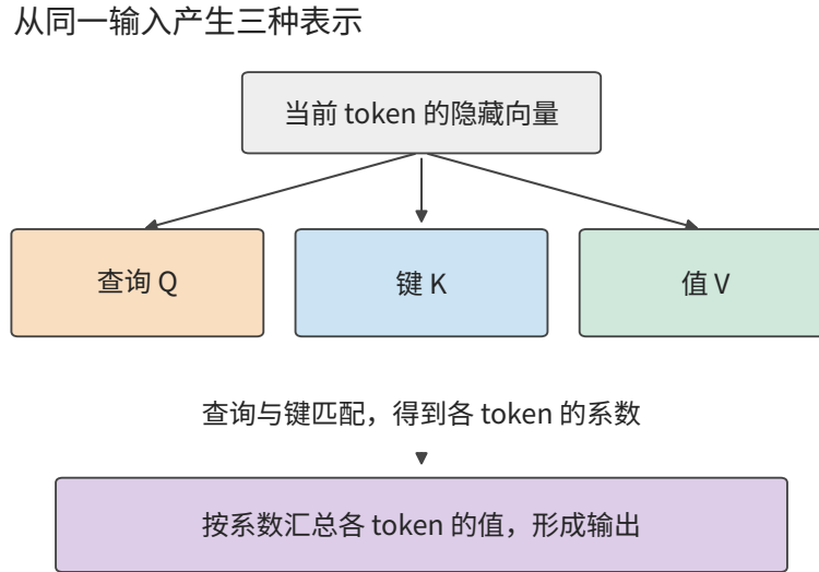
图 2-3 同一个 token 的输入经不同投影产生查询、键和值。注意力先用查询与键计算 token 之间的关系，再用这些关系汇总值。
