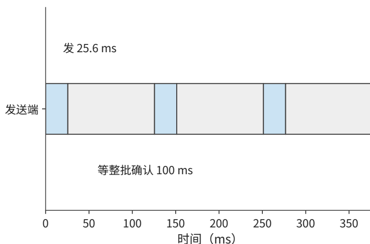
图 12-17：固定窗口 64 KB，链路 20 Mbit/s，一批数据发送需 25.6 ms。为单独显示停等，图设接收方收齐一批后统一确认，从这批数据全部发出到收到整批确认再需 100 ms；每批完整周期为 125.6 ms。
