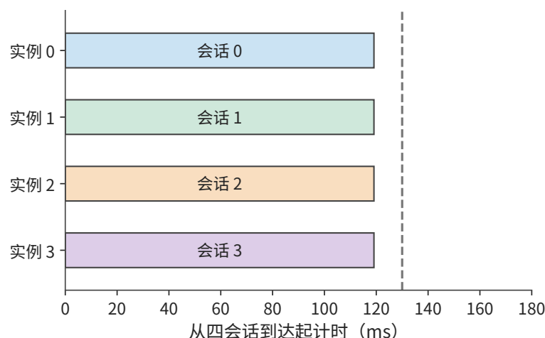
图 6-48：四会话同时推进，每个约 119.1 ms 完成。颜色与相邻配置图中的会话一致。本图使用四个 TP2 实例，每实例两张卡，每个会话续写八个 token；虚线为 130 ms 期限。
