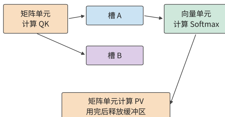
图 4-21 矩阵与向量单元通过完整行组交接。QK 产生分数，Softmax 产生概率，PV 使用概率后释放槽；另一槽容纳相邻行组，使不同组可以重叠推进。
