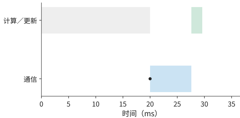
图 7-54：连续环串行安排：计算 20 ms，通信约 7.6 ms，更新 2 ms。灰为计算，蓝为通信，绿为更新；圆点为通信数据就绪。
