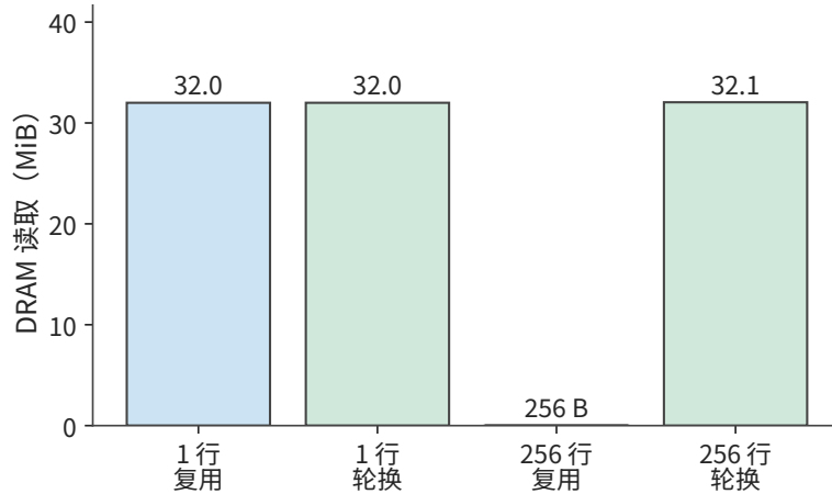
图 4-38 相同四个条件下另行采集的 DRAM 读取计数。单行均约 32 MiB，256 行复用为 256 bytes、轮换约 32.1 MiB。访问计数与常规计时分别测量。“复用”与“轮换”分别表示保持和更换权重地址。
