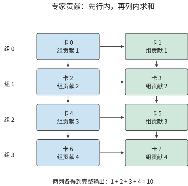
图 6-18：横向箭头表示组内两卡求和，纵向箭头表示四个组求和。格内数字是某个输出元素经组内求和后的值，两列各自都得到相同的完整结果 10。
