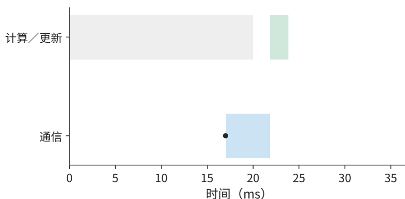
图 7-59：本图从提前通信的分层配置出发，只把可用网卡减为一张。跨服务器两轮各要挤过 96 MiB，通信约 4.8 ms，超出计算区间，整步约 23.8 ms。上述时间线采用同一横轴范围。灰色为计算，蓝色为通信，绿色为更新；圆点为通信数据就绪。
