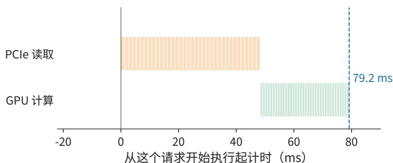
图 9-32：先把 1.125 GiB 历史 KV 整份从主机内存读入，再计算 256 个新 token，共 79.2 ms。橙色为 PCIe 读取，绿色为 GPU 计算，每一小段对应一层。
