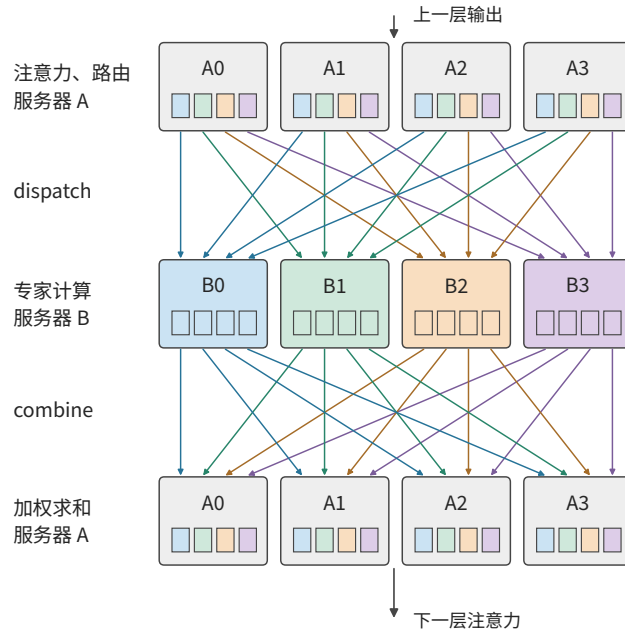
图 9-16：一层 MoE 在两台服务器间的执行顺序，时间从上到下。A0–A3 执行注意力与路由，B0–B3 执行专家。小方块表示一张 A 卡发往一张 B 卡的一组输入，颜色标出它去往哪张 B 卡；dispatch 把各色方块送到同色的 B 卡，combine 再把结果送回原来的 A 卡。两次交换都是 4 \times 4 的 All-to-All。
