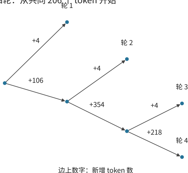
图 8-17：前四轮代码 Agent 输入的压缩前缀树。根部已有 206 个共同 token，边上是新增数量，叶子是输入轮次。分叉表示后续内容不同。
