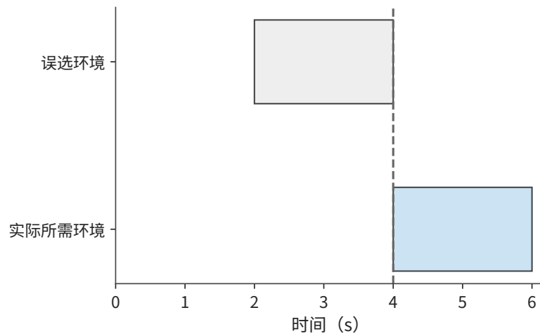
图 11-19：预测错误：第 2–4 s 准备了不必要的环境（灰色）；第 4 s 取消后，再花 2 s 准备实际所需环境。此图采用立即取消、无资源争用的题设。
