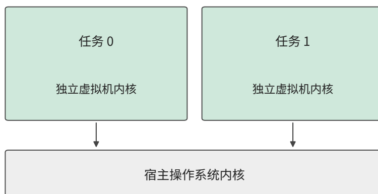
microVM的隔离边界
