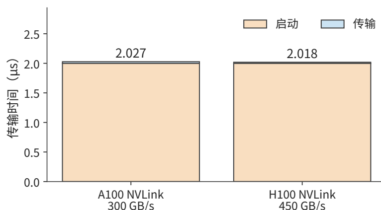
图 4-24 一次 8 KiB 传输的启动与传输时间。固定启动开销 2 \mu s，NVLink 从 A100 的每方向 300 GB/s 换成 H100 的 450 GB/s，只缩短很薄的蓝色传输项。
