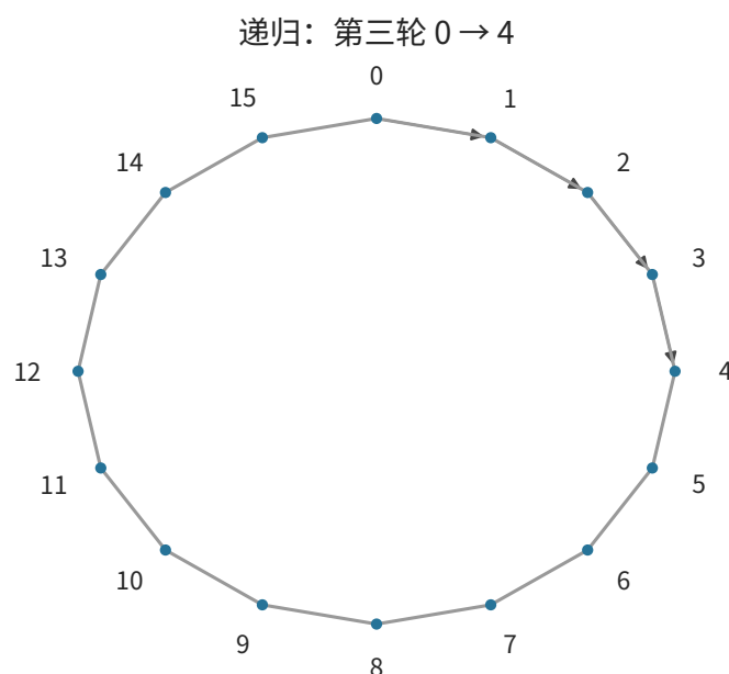
图 6-31：递归算法第三轮，卡 0 发往卡 4。细线为 16 张卡组成的物理环，箭头标出经过的四条链路。
