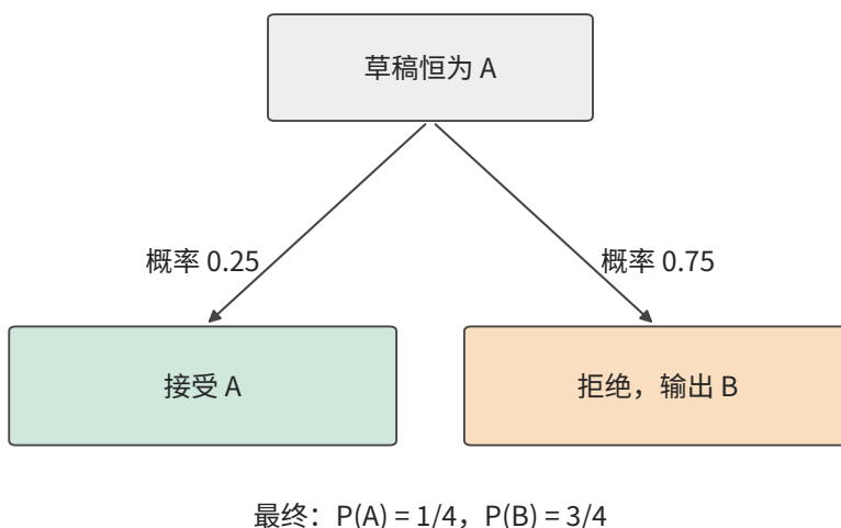
图 8-30: 接受 A 的概率为 1/4 ，拒绝后输出 B 的概率为 3/4 。两条路径合起来给出目标分布。
