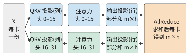
注意力子层：按头切分，输出投影产生部分和
