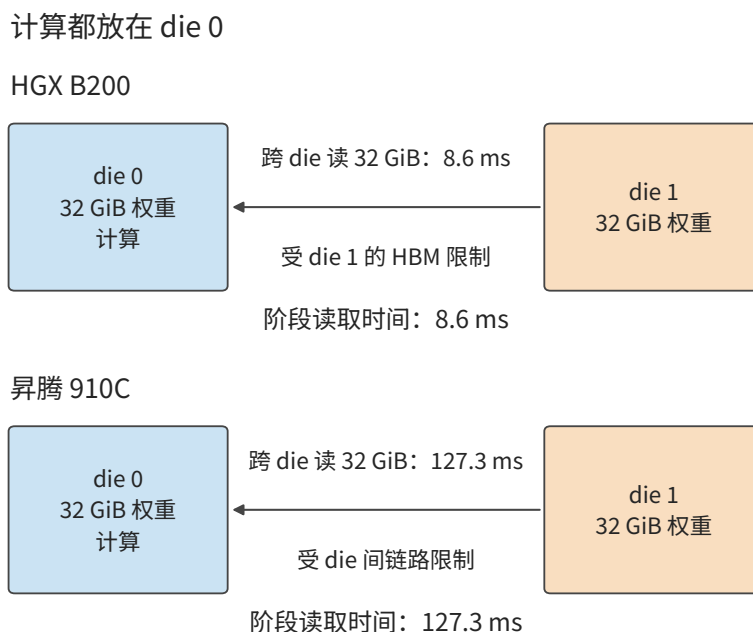
图 4-22 计算都放在 die 0 时, 要跨 die 读取 die 1 上的 32 GiB 权重。B200 的跨 die 读取受 die 1 的 HBM 限制, 约 8.6 ms, 与本地读取相同; 昇腾 910C 受 die 间链路限制, 约 127 ms。
