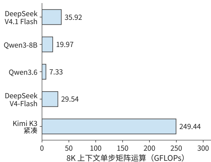
图 2-29 相同单请求、已有 8K 上下文时的单步矩阵运算量。按各模型在表 2-C 说明的执行路径累计，Kimi K3 采用紧凑 MLA。
