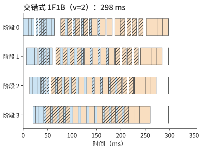
图 10-21：交错式 1F1B ( v=2 ) 的各阶段时间线，完成时间 298 ms。蓝色为前向，橙色为反向，绿色为参数更新，斜线块为每卡的第二个层块。每个块约为图 10-18 中的一半长，预热与排空阶段的空隙被另一个层块的计算填上，阶段 3 的第一个前向从 33 ms 提前到约 20 ms；每个 micro-batch 要多穿过四条边界。
