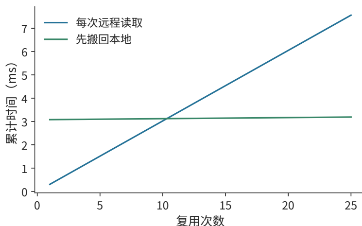
图 7-23：每次远程读取和本地读取都只访问 10%，但搬回时仍复制全部快照；因此需要更多复用才能抵消固定成本。
