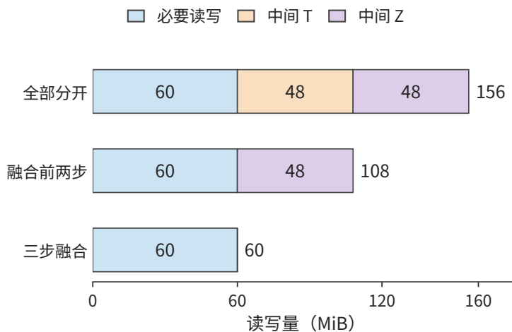
图 5-15：每少保存一个 24 MiB 中间量，就少一次写出和一次读入，共 48 MiB。G、U 为 BF16，最终输出占 1 byte/元素，量化 scale 预先给定。各方案采用相同的运算与舍入顺序。
