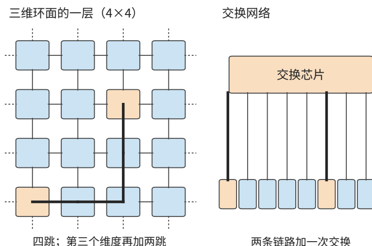
图 6-34：左侧是三维环面的一层，每张卡与四个邻居直连，虚线表示每一维首尾相连；从角上的卡到中心的卡要经过四跳，加上第三个维度最多六跳。右侧是交换网络，任意两张卡之间都是两条链路加一次交换。橙色是相距最远的一对卡，粗线是它们之间传输经过的路径。
