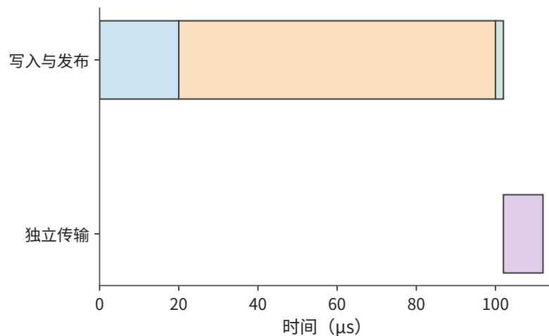
图 7-35：将独立传输也排在发布之后：先写入 20 \mu\text{s} ，恢复并使数据可见 80 \mu\text{s} ，通知 2 \mu\text{s} ，再执行独立传输 10 \mu\text{s} 。
