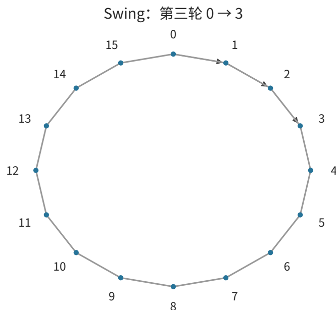
图 6-32: 同一物理环上, Swing 第三轮卡 0 发往卡 3, 经过三条链路。每张卡这一轮的发送量仍为 1 MiB。
