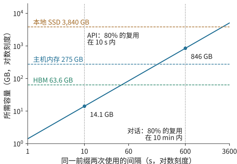
图 9-30：所需容量随复用间隔线性增长。斜线为 C = rT ，其中 r \approx 1.41 \text{ GB/s} 是一张 A100 连续执行无命中 8K prefill 时产生 KV 的速率；三条虚线是每张 GPU 在三级存储中的容量；两条竖线标出两类负载 80% 复用所在的时间范围。两轴均为对数刻度。
