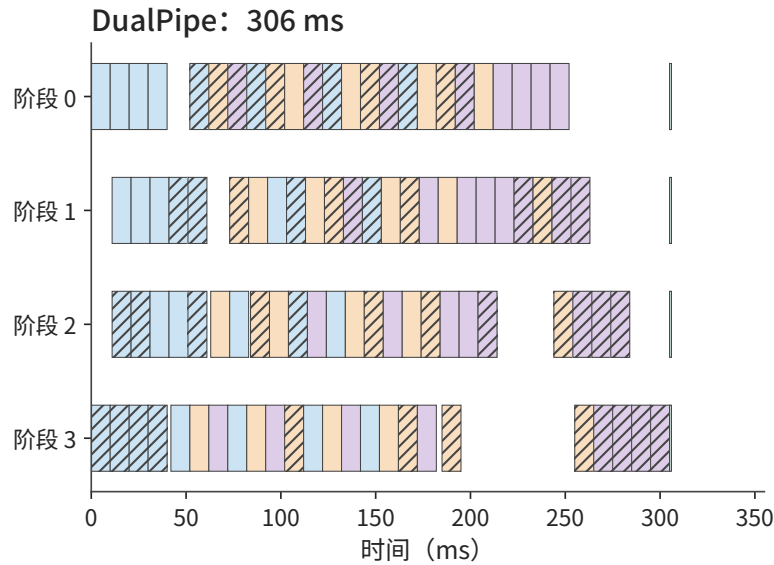
图 10-23: DualPipe 的各阶段时间线，完成时间 306 ms。颜色同图 10-22，斜线块为从阶段 3 进入的另一半 micro-batch（反方向）的计算。每个阶段同时承载两个方向，一个方向的预热和排空空隙由另一个方向的块填上；代价是每卡保存两份参数。
