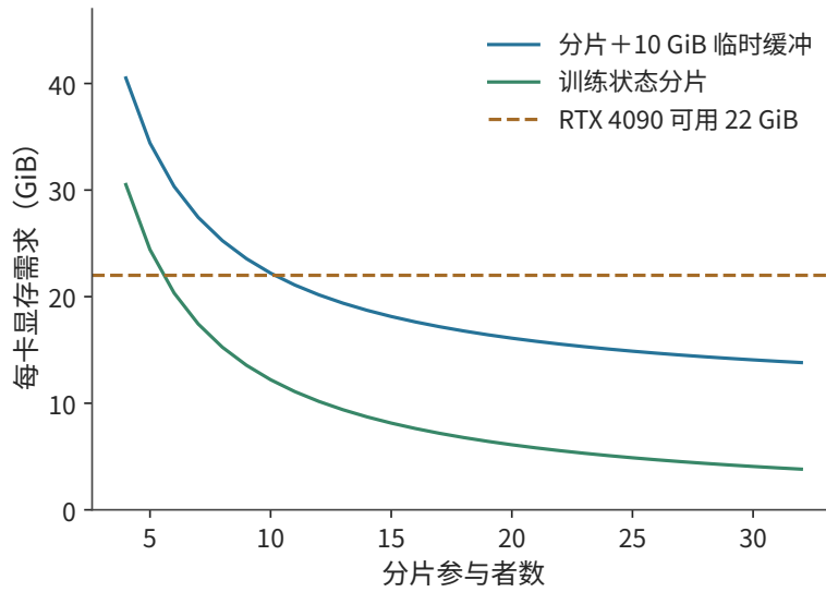
图 10-16：给定附加存储需求时，分片数决定哪些方案满足容量要求。曲线为 16N/d + 10 GiB，水平线为 RTX 4090 每卡 22 GiB 可用显存。曲线低于预算的区域可以容纳这些训练状态和缓冲区；纵向距离给出容量余量。
