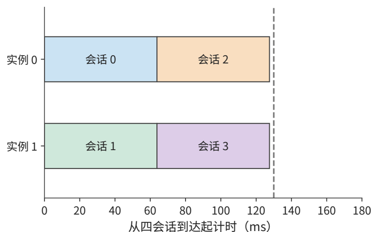
图 6-49：每个实例顺序处理两个会话，分别在约 63.8 ms 和 127.6 ms 完成。本图使用两个 TP4 实例，每实例四张卡，每个会话续写八个 token；虚线为 130 ms 期限。
