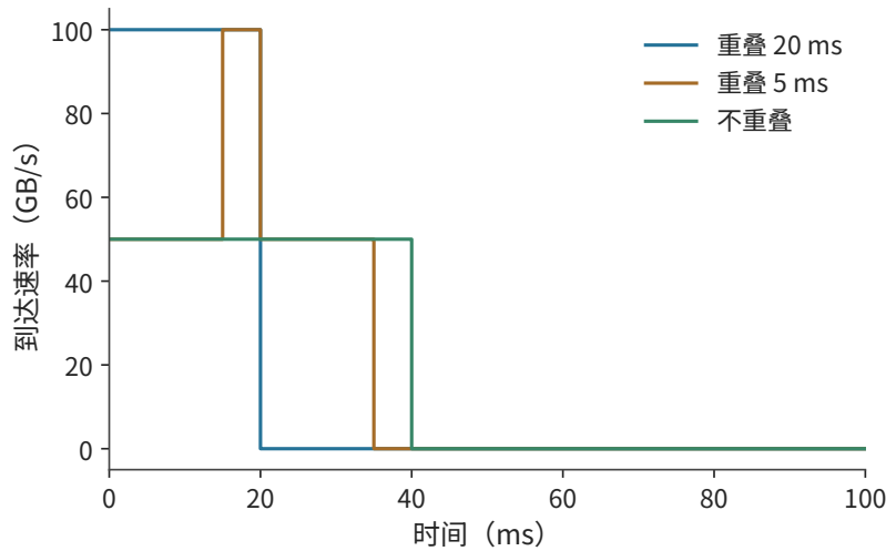
图 7-40：两作业每 100 ms 各发送 20 ms，单作业速率 50 GB/s。不同高峰重叠程度产生不同的总到达速率，共享出口为 50 GB/s。
