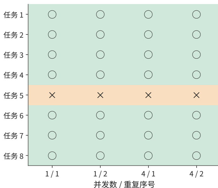
图 8-26: BF16 KV 基线。每行是一道固定任务，四列为并发 1、4 下各两次自然生成。绿色圆圈正确，橙色叉号错误，共 28/32 正确。
