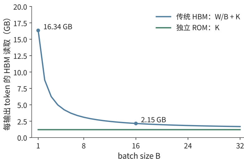
图 8-4: 每输出 token 分摊的 HBM 读取量。固定 8K 上下文，传统路径为 W/B+K ，独立快速 ROM 路径为 K ；纵轴按上述公式计算读取量。 W 是整批读取的权重字节数， B 是批内请求数， K 是单请求本步读取的 KV 字节数； W/B+K 为每个输出 token 分摊的读取量。
