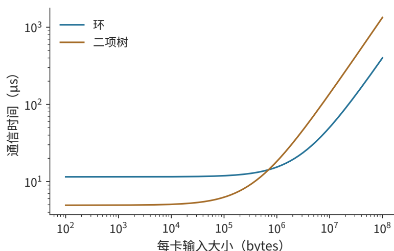
图 6-26: 八卡环形算法与未分段二项树的时间模型，每轮 0.822 \mu\text{s} 、每方向 450 \text{ GB/s} 。交点约为 680 \text{ KiB} ； 10 \text{ KiB} 的 decode 输入位于主要受启动开销影响的一侧， 80 \text{ MiB} 的 prefill 输入位于主要受数据传输时间影响的一侧。
