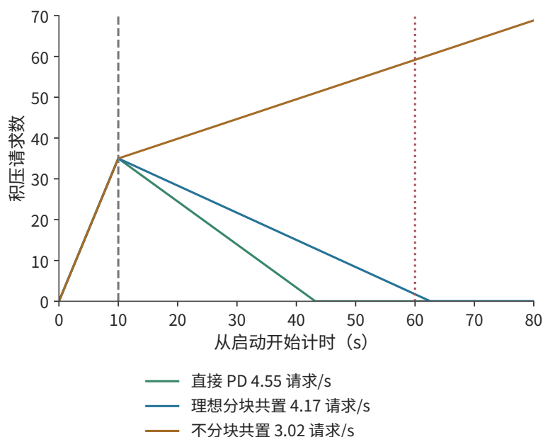
图 9-42：服务余量决定启动积压的消退速度。连续流量模型，每秒到达 3.5 个请求，启动 10 秒后积压 35 个。就绪后服务率分别为直接 PD 的 4.55、理想分块共置的 4.17 和不分块共置的 3.02 请求/s；前两者从开始启动算起在第 43 与第 63 秒排空，后者持续积压。例 9.8 的排空期限为第 60 秒。
