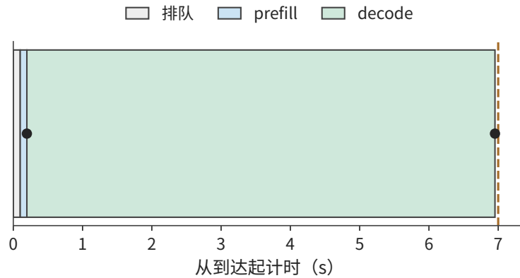
图 8-2: 一条输出 256 个 token 的请求。排队 0.1 秒、prefill 0.096 秒，后续 255 个输出间隔各为 26.5 ms（实验 8-1 的 batch 1 实测）。横条按实际时间比例绘制，点标出首、末 token；7 秒虚线是完成时限。
