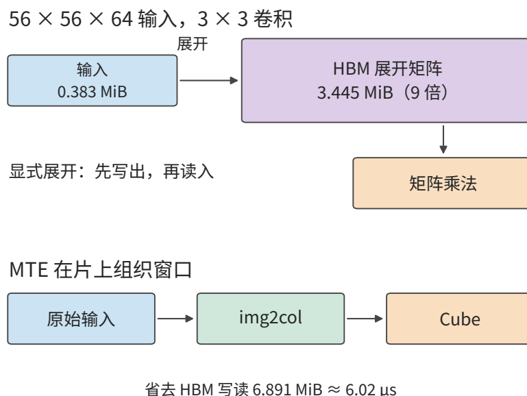
图 4-29 同一个 3×3 卷积的两条准备路径。显式展开形成九倍大小的中间矩阵；MTE 在片上组织窗口，省去 HBM 上 6.891 MiB 的中间结果读写。
