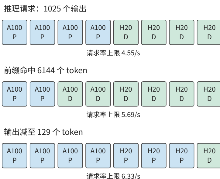
图 9-11：请求组成改变资源分配。四张 A100 与四张 H20，阶段能力按例 9.2 的方法推出；第一行为 8192 输入、1025 输出的推理请求，第二行只减少 P 的新输入，第三行恢复完整输入并将输出减至 129 个 token。方块表示卡，每行下方为对应的吞吐率上限。P 为 prefill 池，D 为 decode 池。
