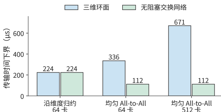
图 6-35：每张卡六个 50 GB/s 端口、每卡发送 32 MiB。沿维度归约时两种拓扑都用满端口带宽；均匀 All-to-All 时环面上的数据平均要走三跳，共享链路承载的数据随之增加，512 卡时增至六跳。图中是链路负载给出的下界，不含启动开销与排队；交换网络按无阻塞计，即交换层不限制各端口同时满速收发。
