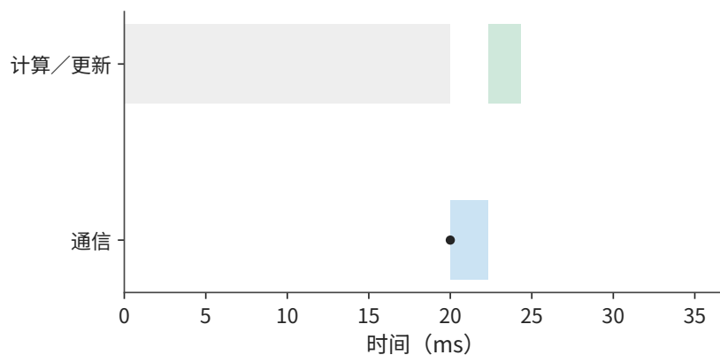
图 7-56：本图采用分层归约，其他计算与更新时间不变。每张网卡 128 个在途事务限制远端吞吐，通信拉长到约 2.3 ms，整步约 24.3 ms。灰色为计算，蓝色为通信，绿色为更新；圆点为通信数据就绪。
