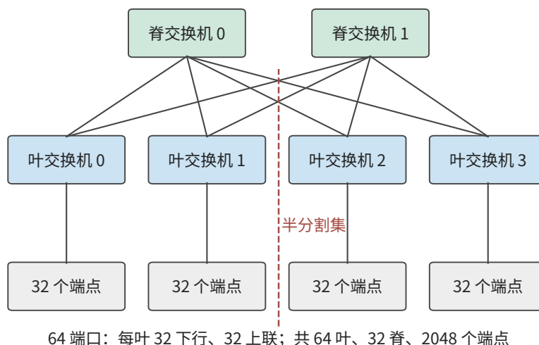
图 7-3：两层 Clos 网络。每台叶交换机一半端口接服务器、一半接脊交换机，任意两台叶交换机之间经任一脊交换机相通；虚线把端点分成两半，穿过它的叶—脊链路就是半分分割集。图中画出四台叶交换机和两台脊交换机作代表，64 端口时实际为 64 台叶交换机、32 台脊交换机。
