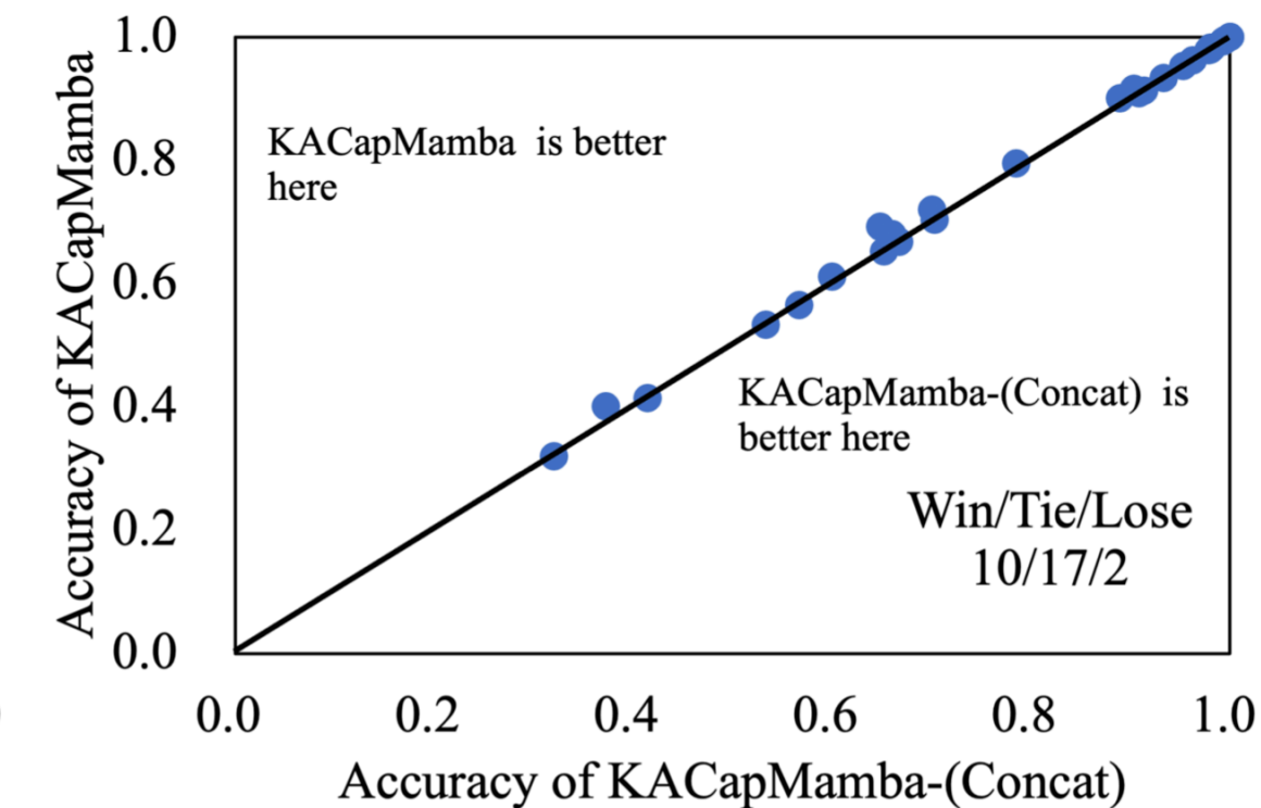
(f) KACapMamba-(Concat) vs. KACapMamba
