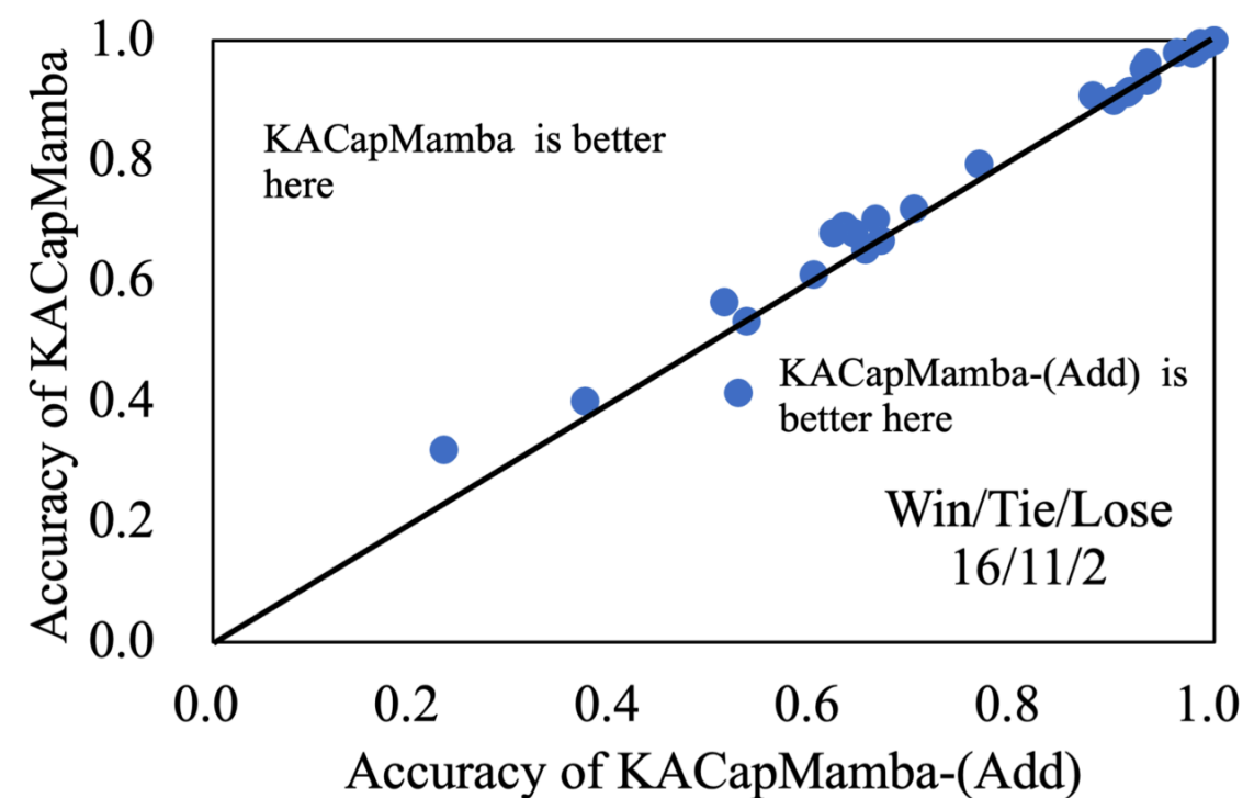
(d) KACapMamba-(Add) vs. KACapMamba
