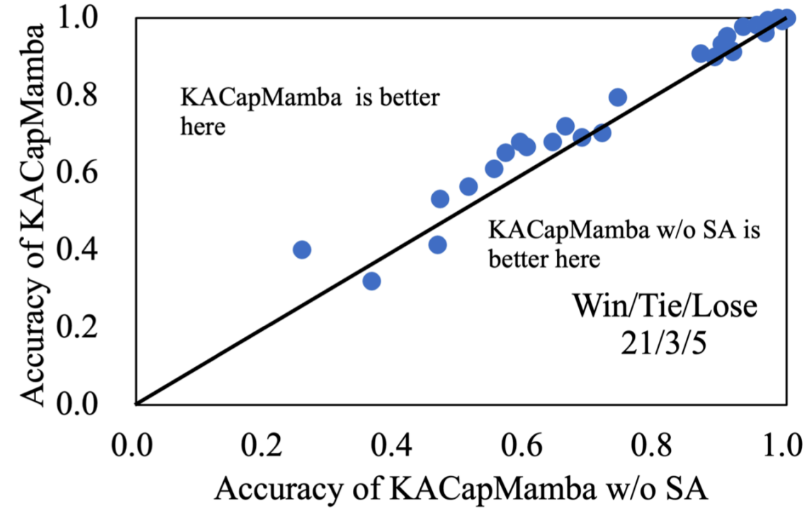
(c) KACapMamba w/o SA vs. KACapMamba
