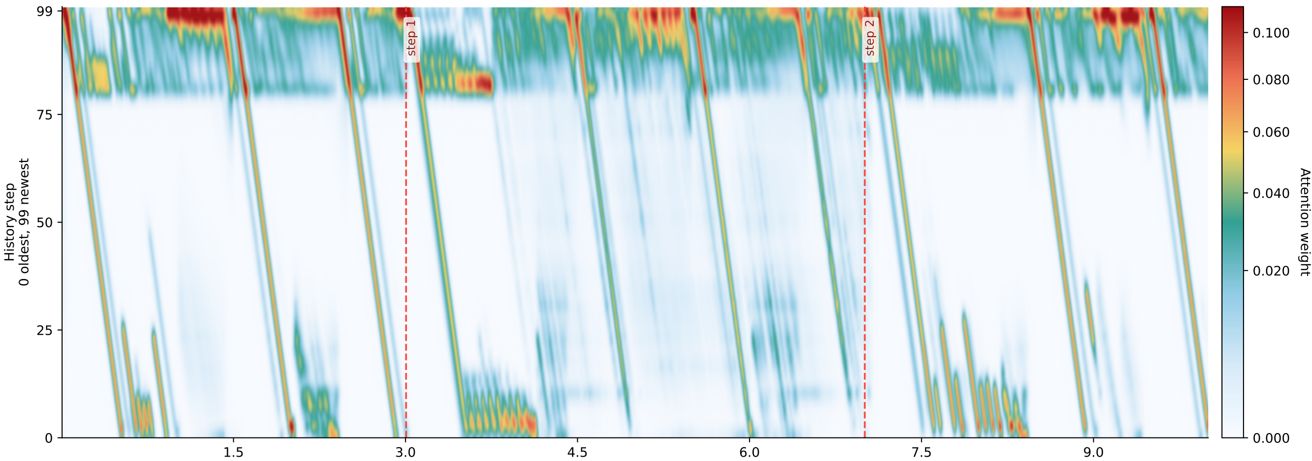
TRACE Fast Attention v2
