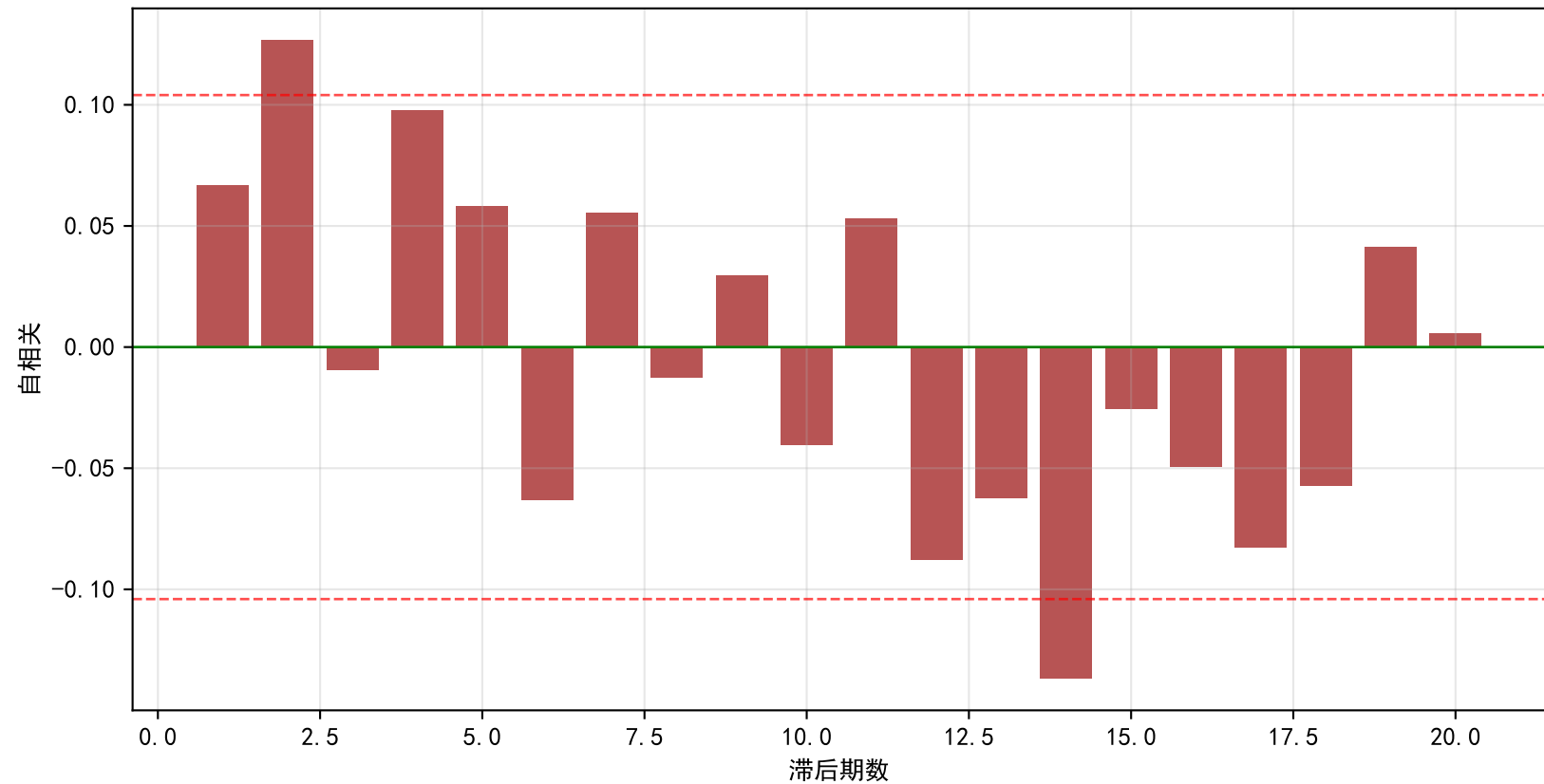
月度收益率自相关函数
