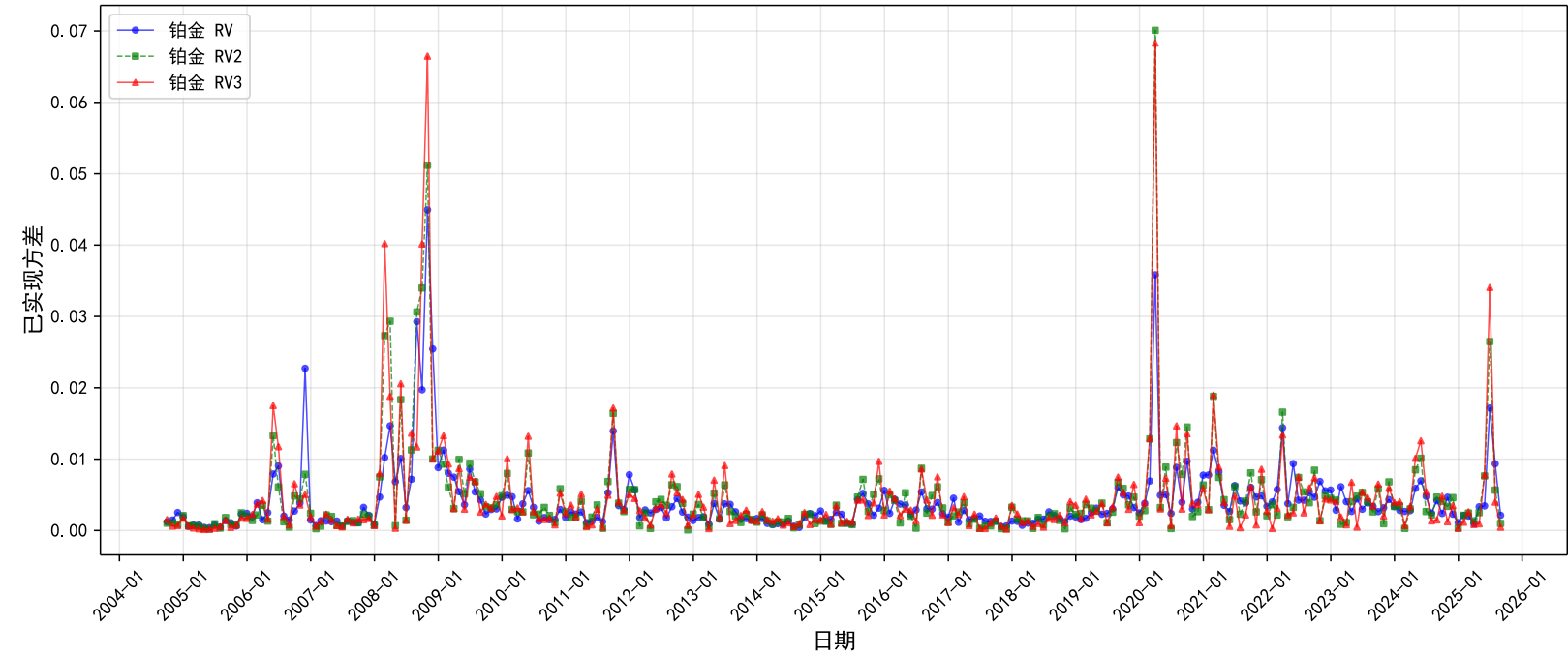
铂金月度已实现方差 (RV、RV2、RV3)
