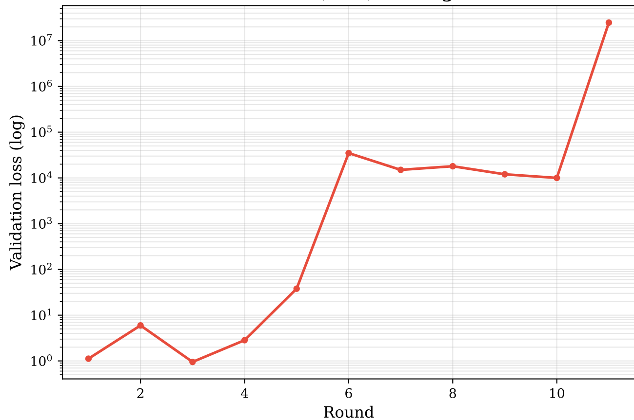
NYU V2: B2 (HCA) - divergence
