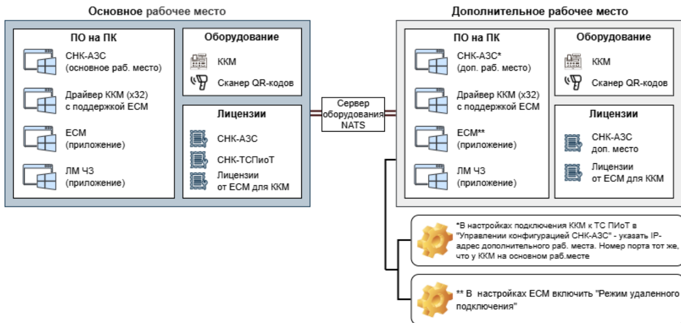
Рисунок 1. Схема необходимого ПО, лицензий и оборудования для рабочих мест
