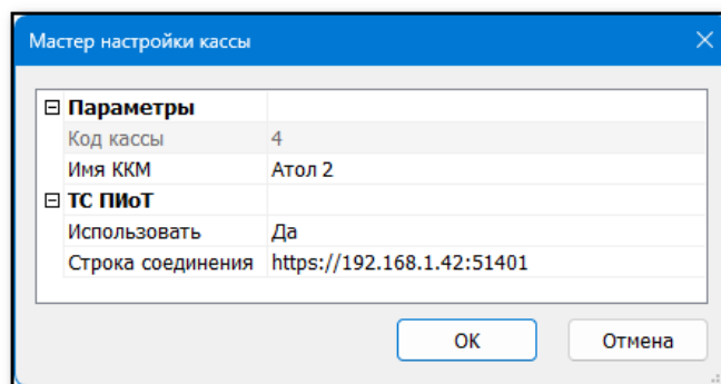
Рисунок 4. Настройка для ККМ дополнительного рабочего места
