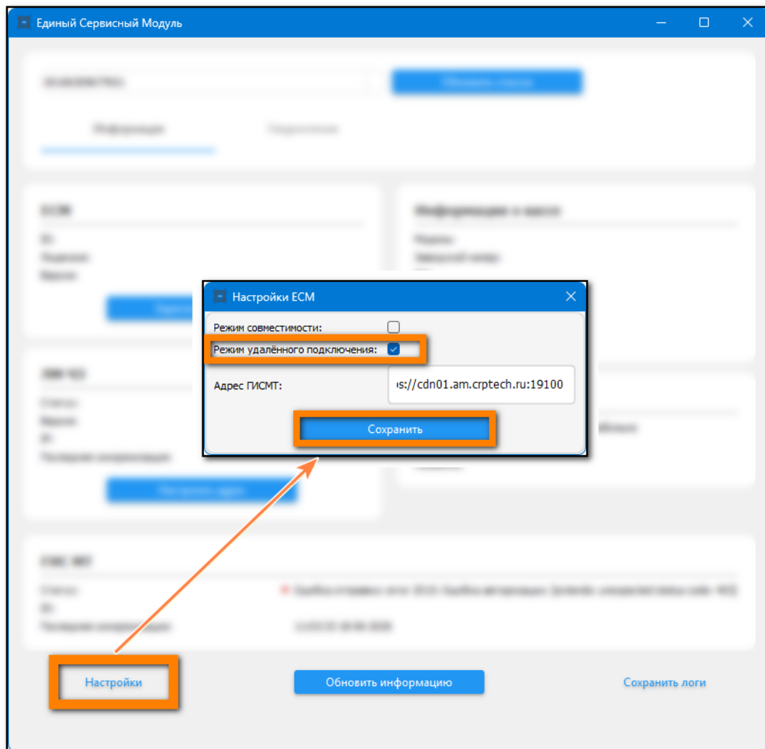
Рисунок 5. Настройки в ЕСМ на дополнительном рабочем месте
