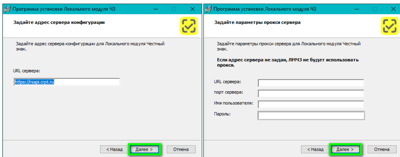
Рисунок 3. Настройка соединения с сервером ЧЗ
