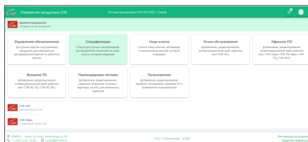
Рисунок 21. Раздел "Спецификации"
