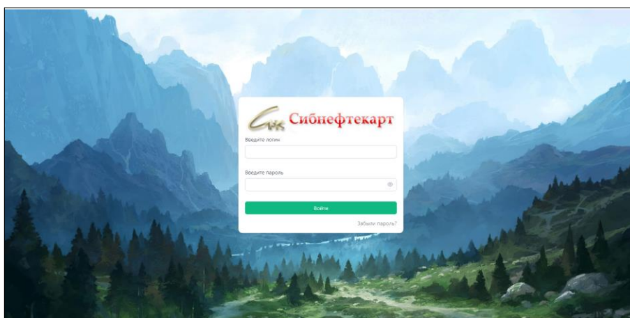
Рисунок 1. Страница авторизации
