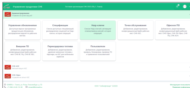
Рисунок 23. Раздел "Наср-ключи"
