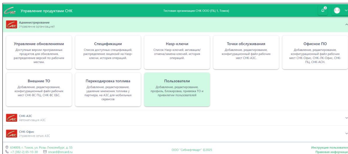
Рисунок 3. Раздел "Пользователи"
