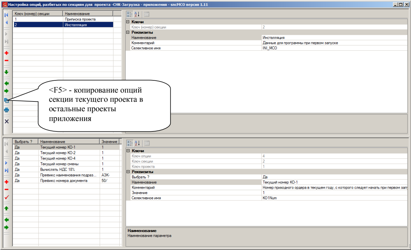
Рисунок 14. Настройка конфигурации. Опции секции "Инсталляция".
