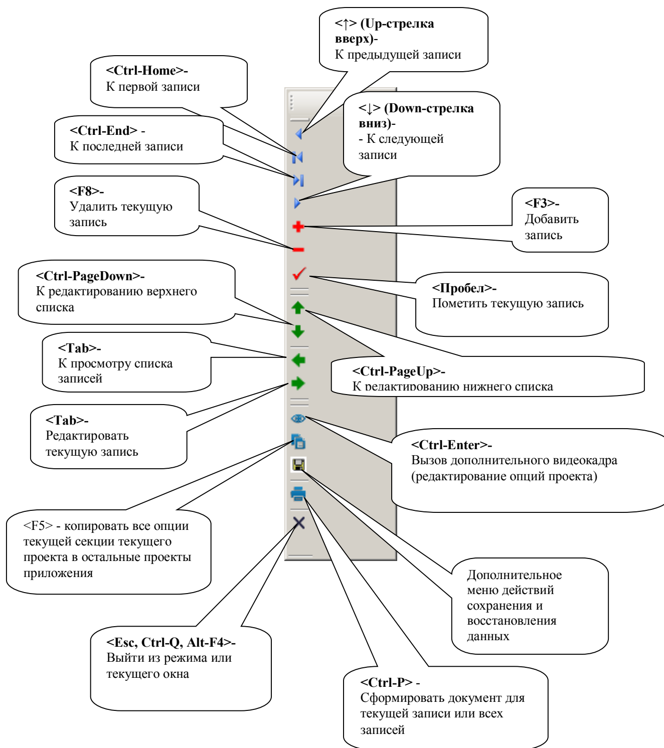
Рисунок 12 . Назначение клавиш навигатора
