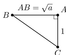
图 2：最大面积临界状态 \angle BAC = 90^\circ 时， S_{\max} = \frac{1}{2}\sqrt{a}
