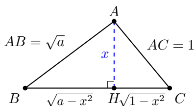
图 1：一般状态下的三角形拼接 底边 BC = \sqrt{a-x^2} + \sqrt{1-x^2}
