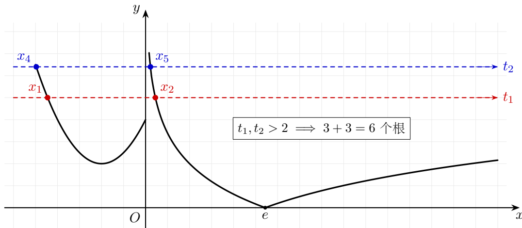
图 2： 0 < a < \frac{7-2\sqrt{10}}{9} 时，两个 t 根均大于 2 对应 6 个实数根示意图
